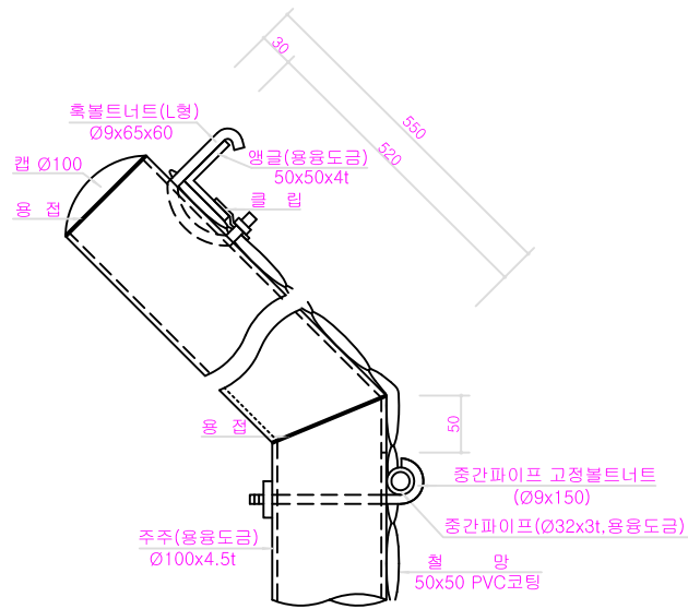
"A" 상세도
