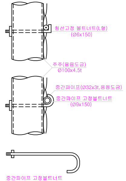
"B" 상세도
