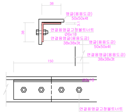
"D" 상세도
