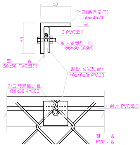
"C" 상세도
