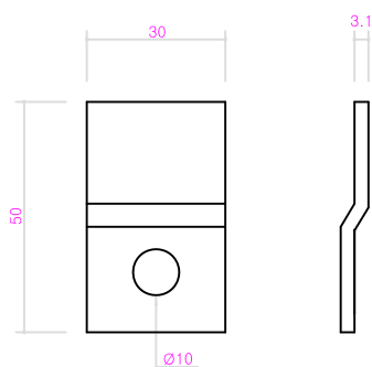
클립 상세도
