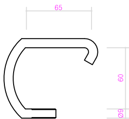
클립 상세도
