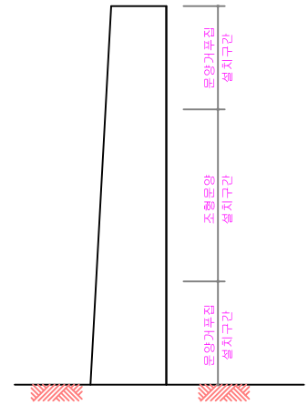
단면도
