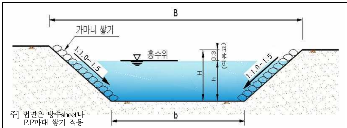
<그림 4.3> 가배수로 표준단면도
