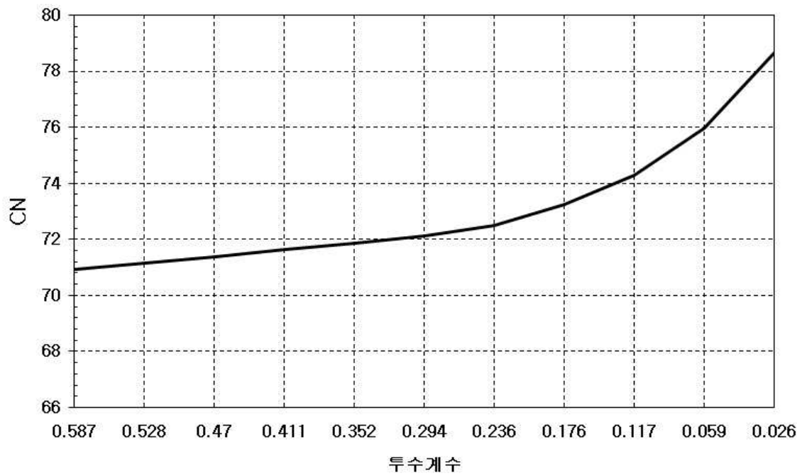
<그림 B.5> 투수성 보도블록 투수계수별 CN
