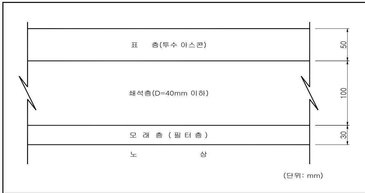
<그림 B.8> 투수성 포장 일반도
