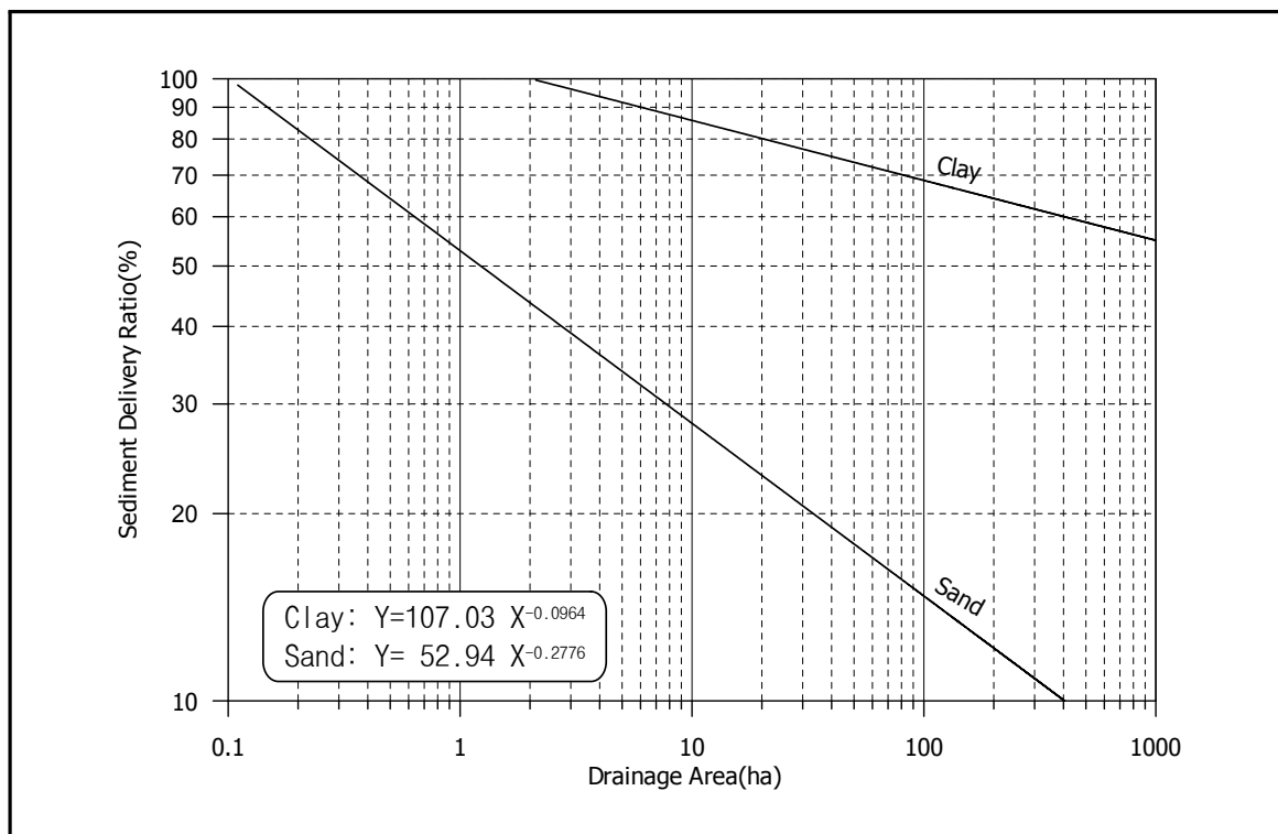
<그림 4.1> TRB(1980) 도표
