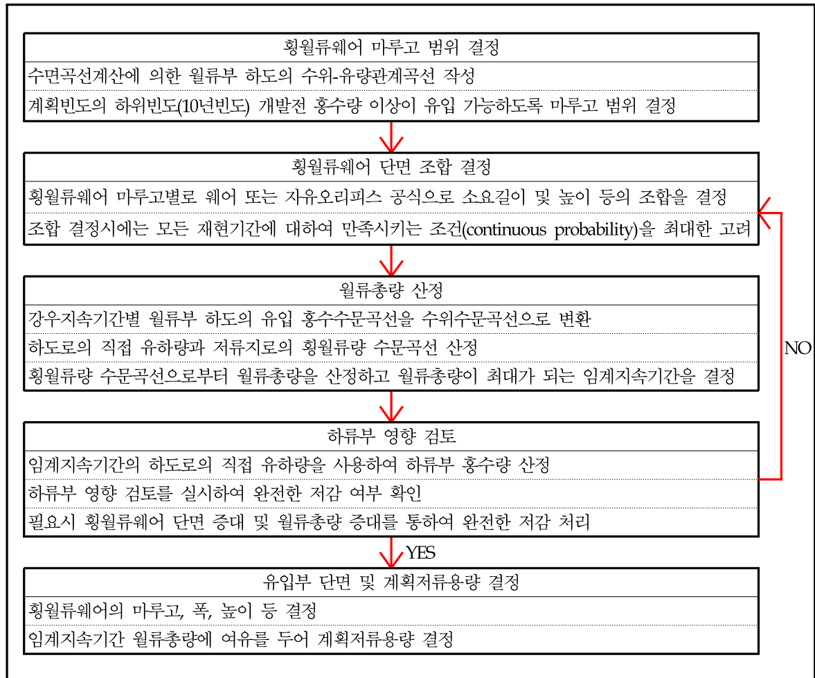
<그림 4.6> 유입부 단면 및 계획저류용량 결정
