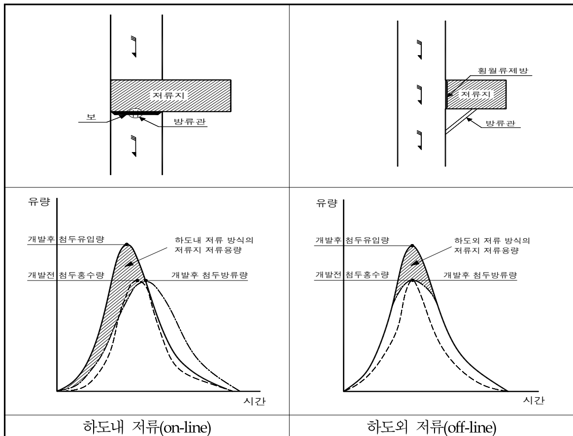
<그림 4.5> 저류지의 홍수조절 방식
