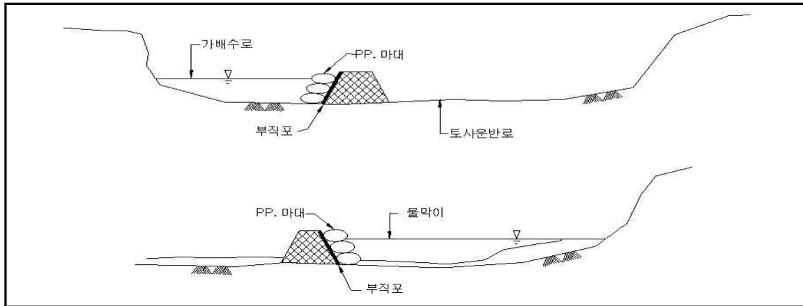
<그림 4.2> 가배수로 및 물막이공의 개요도
