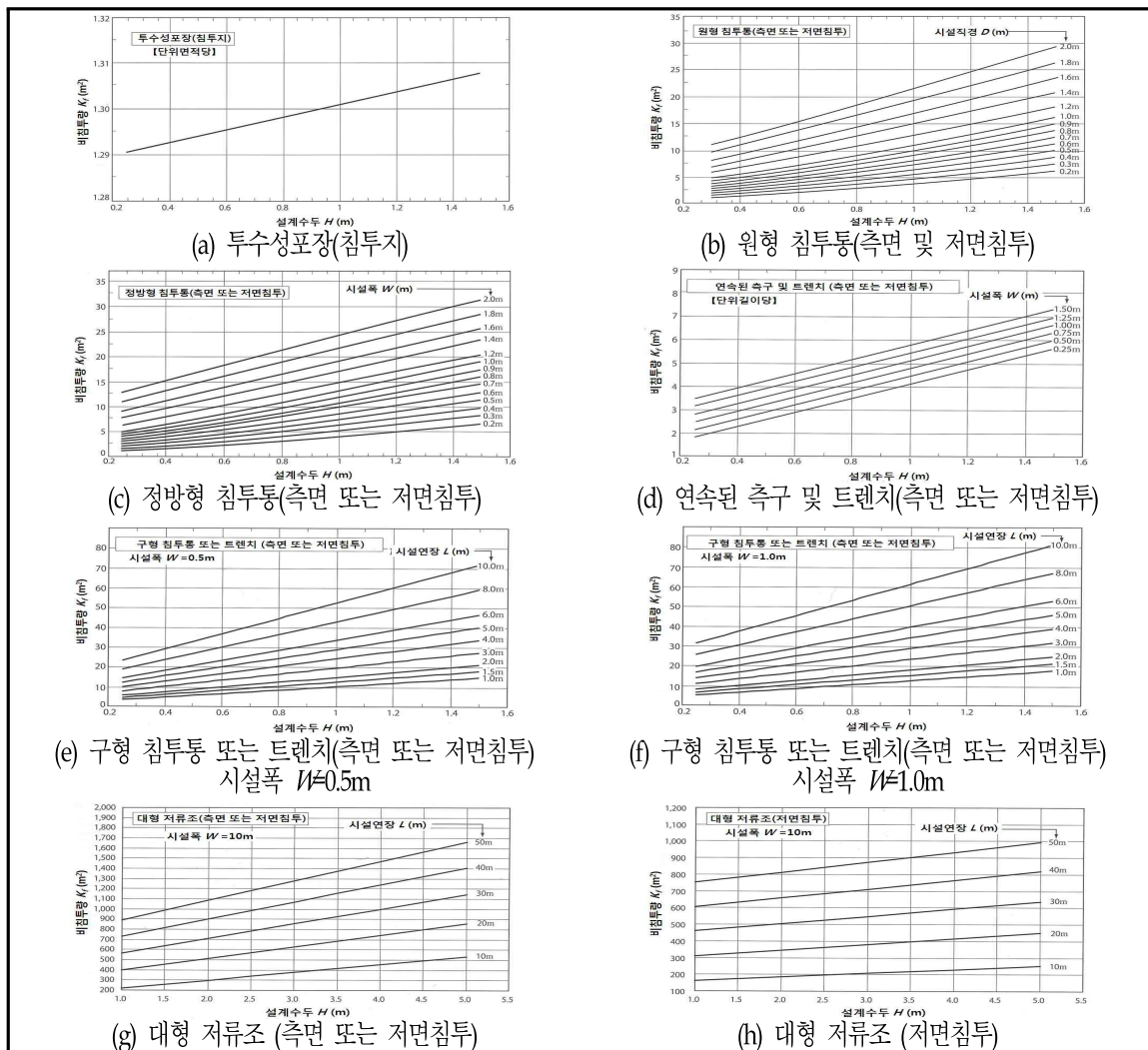
<그림 B.2> 침투시설별 비침투량
