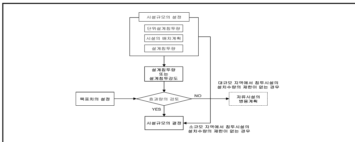
<그림 B.1> 침투시설 규모 결정 절차
