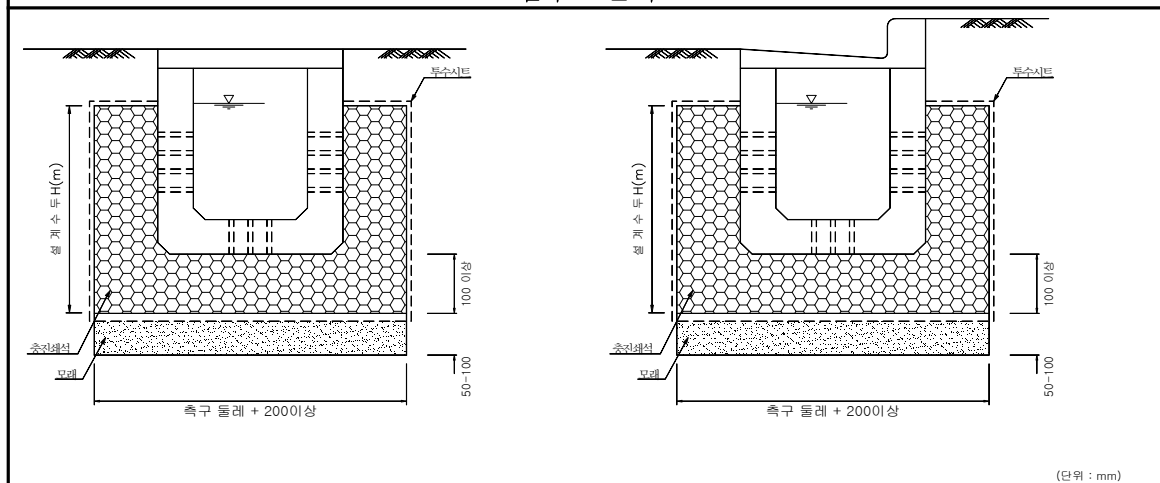
<그림 B.7> 침투통, 침투트렌치, 침투측구 일반도
