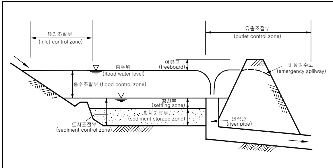
<그림 4.4> 침사지의 구성
