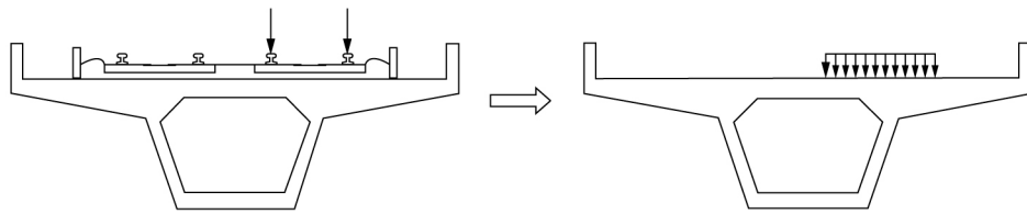
그림 4.2.2 도상의 하중 분포효과를 고려한 모델링
