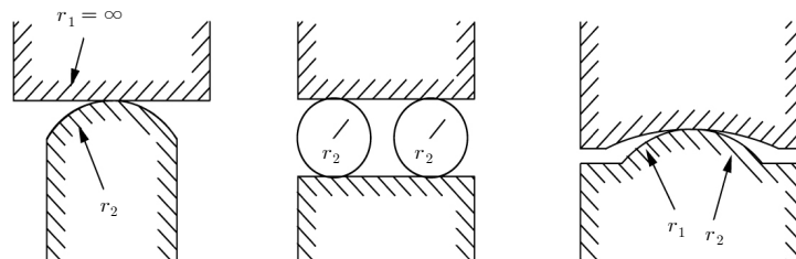
그림 3.1.1 선반침, 로울러받침, 구면받침
