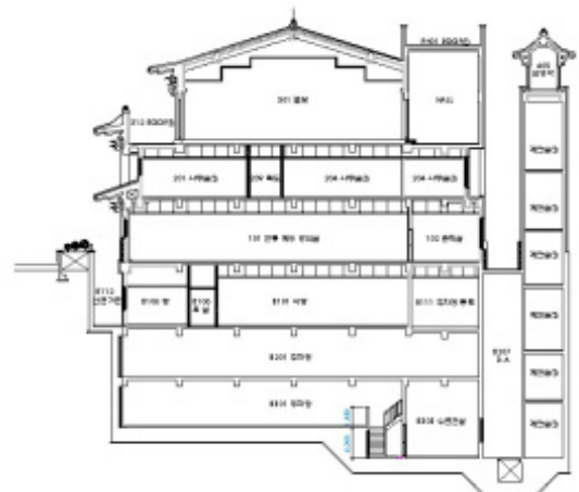
종단면도
