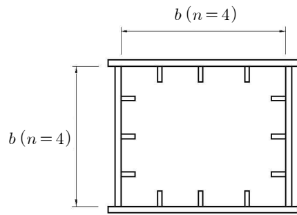
그림 3.4.4 보강된 판의 전폭
