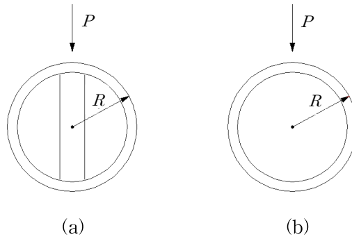
그림 3.13.6 환보강재의 구조
