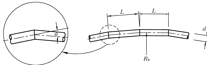
그림 3.13.9 굴곡관
