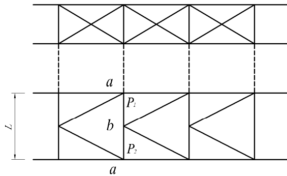
그림 3.10.4 축력이 다른 트러스 부재의 면외 유효좌굴길이(2)
