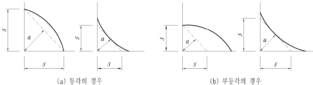
그림 3.5.3 필릿용접의 목두께
