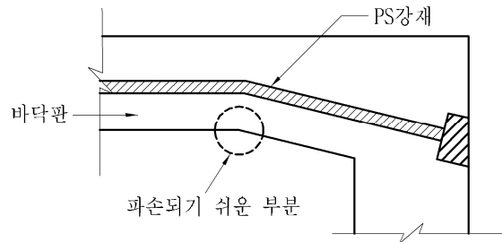
그림 4.3.4 바닥판의 현치부에서 파손되기 쉬운 부분
