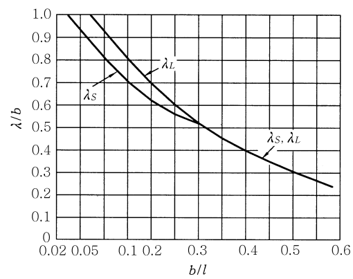
그림 3.8.4 플랜지의 유효폭 결정
