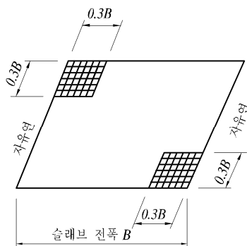
그림 4.8.13 둔각부 슬래브 아래쪽의 가외철근
