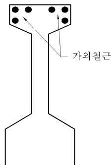
그림 4.3.5 가느다란 보의 가외철근
