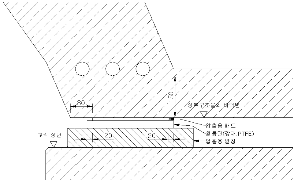
그림 4.15.13 압출용 패드의 위치
