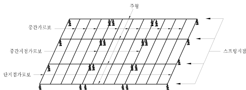
그림 4.11.1 5경간 연속격자형으로 해석한 방법의 예
