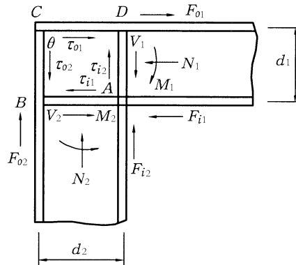
그림 3.14.2 모서리부에 작용하는 외력
