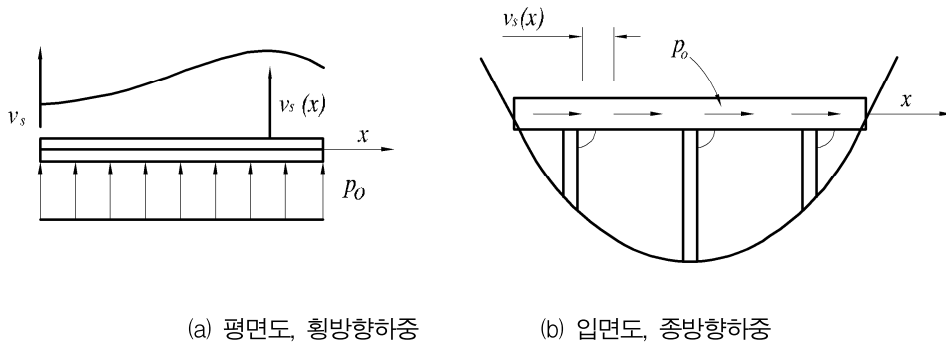
그림 6.5.1 횡방향 및 종방향으로 가정된 하중을 받는 교량 상판
