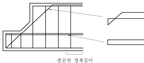
그림 4.15.3 엇갈림부에서의 철근의 정착
