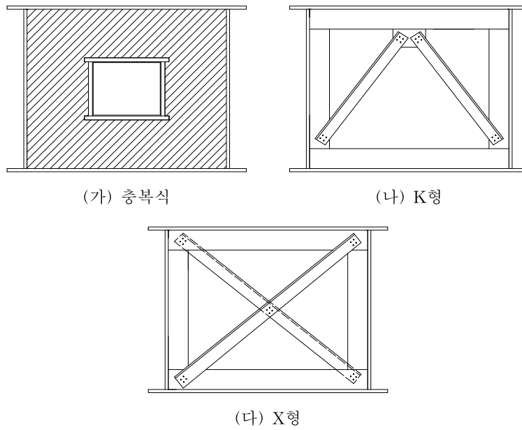
그림 3.8.9 중간다이아프램의 형식
