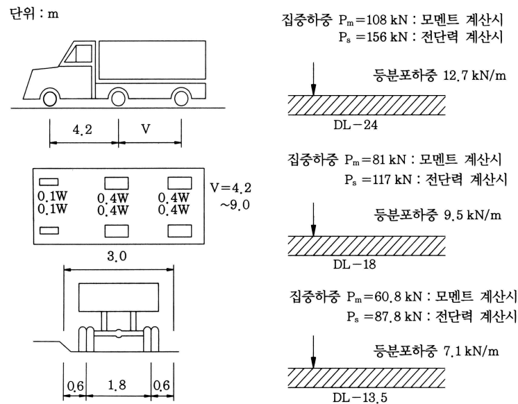
그림 2.1.1 DB 및 DL하중
