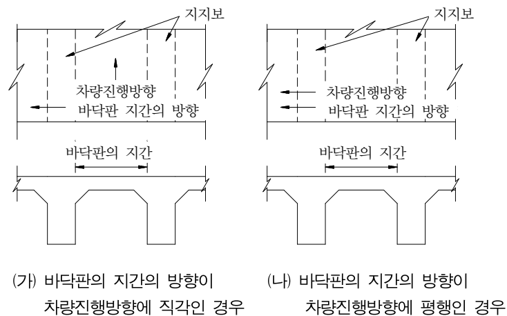
그림 4.7.3 바닥판 지간의 방향
