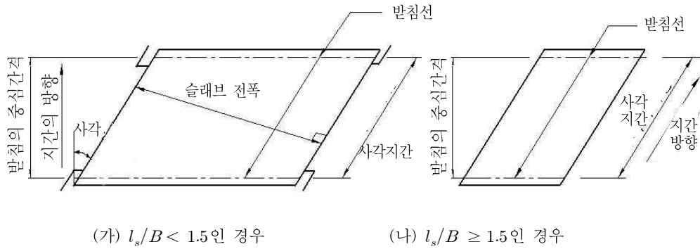
그림 4.8.2 경사슬래브교의 경간방향
