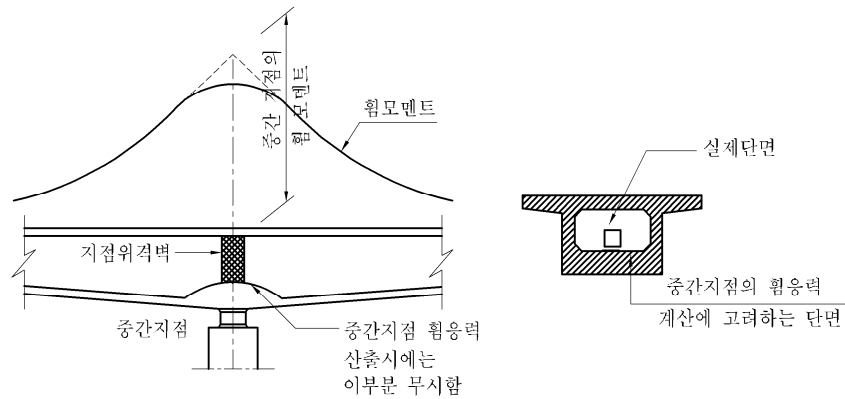
그림 4.11.5 중간받침점의 휨모멘트에 대한 응력계산에 쓰이는 단면
