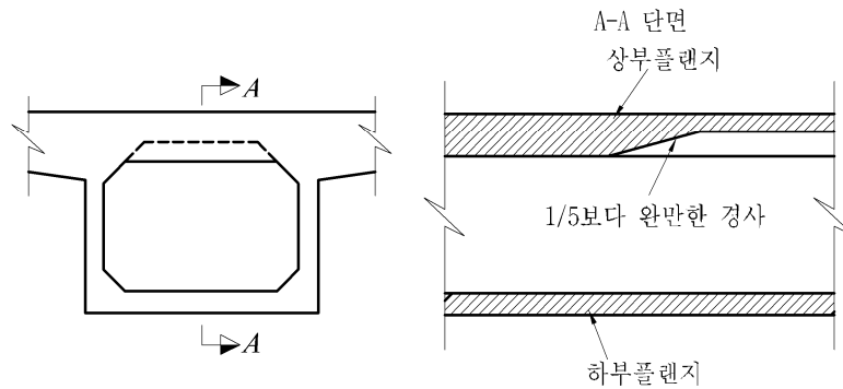
그림 4.10.5 플랜지 두께의 변화
