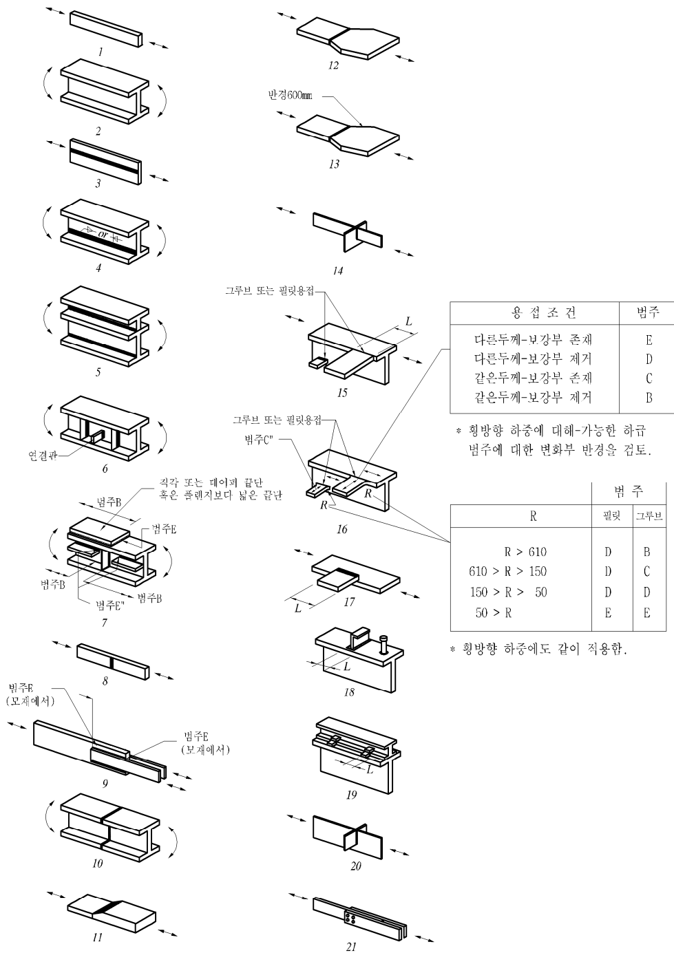
그림 3.3.4 범주의 분류 예
