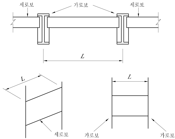
그림 3.7.1 세로보의 지간
