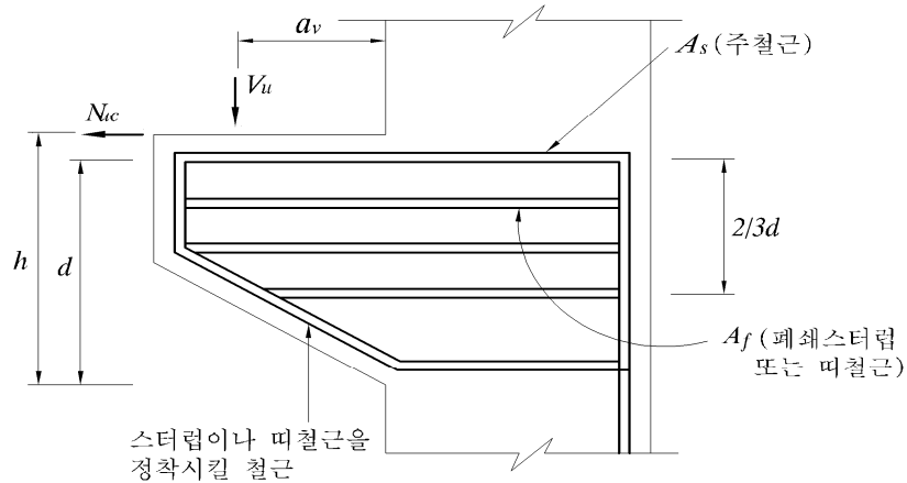
그림 4.4.4 브래킷 및 코벨의 전단
