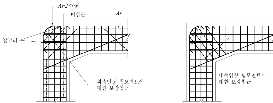
그림 4.12.11 라멘 단절점부의 철근의 배치
