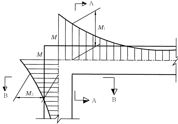
그림 3.14.1 모서리부의 설계휨모멘트
