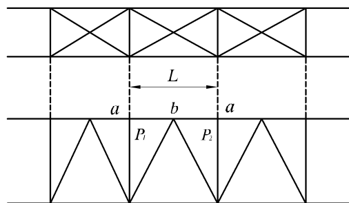
그림 3.10.3 축력이 다른 트러스 부재의 면외 유효좌굴길이(1)
