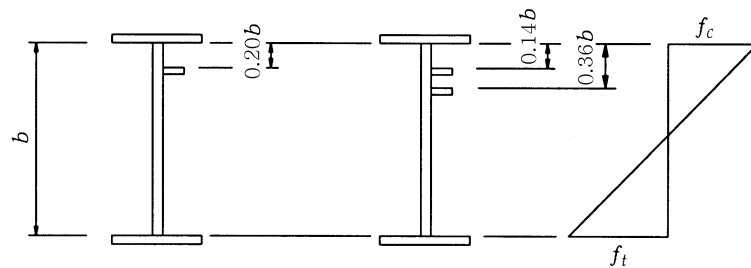
그림 3.8.5 복부판의 응력과 수평보강재의 위치
