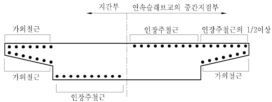
그림 4.8.5 캔틸레버 슬래브의 가외철근
