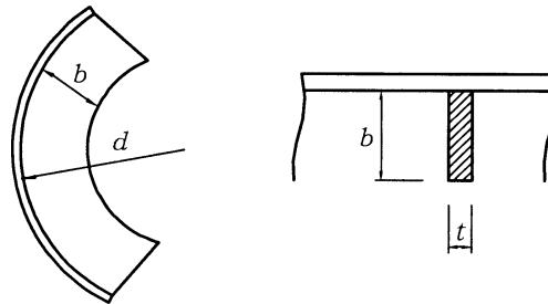
그림 3.13.1 환보강재
