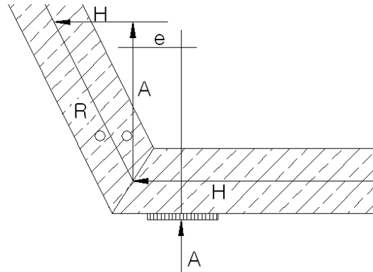
그림 4.15.14 압출용 패드에서의 지점 반력의 영향
