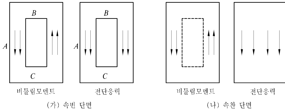
그림 4.4.6 전단응력과 비틀림응력의 합
