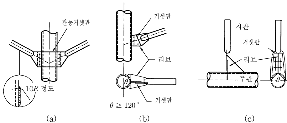
그림 3.13.3 거셋판 연결
