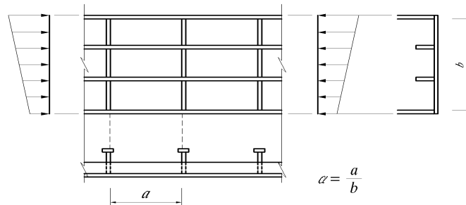
그림 3.4.6 보강판의 종횡치수비, \alpha
