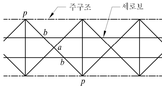
그림 3.10.1 수평브레이싱에서 부재의 길이
