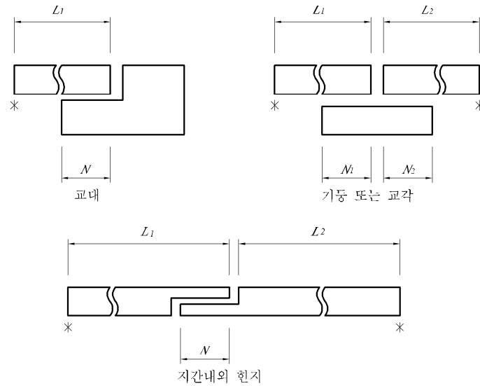
그림 6.4.1 최소 받침지지길이 규정에 관한 치수
