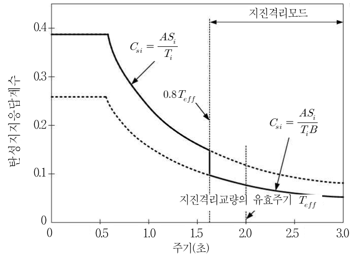
그림 6.9.2 지진격리교량의 탄성지진응답계수
