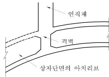
그림 4.13.4 박스 단면 아치리브의 격벽
