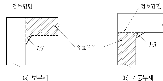
그림 4.12.4 헌치의 유효부분
