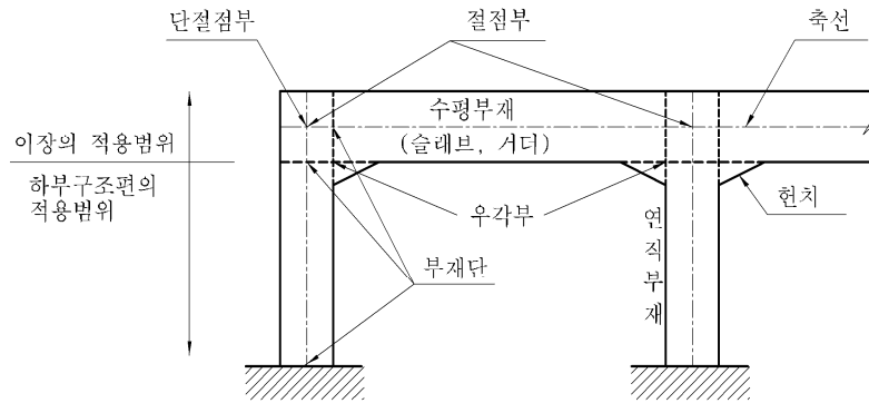
그림 4.12.1 라멘교 각부의 명칭
