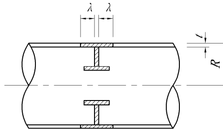
그림 3.13.7 강관의 유효폭
