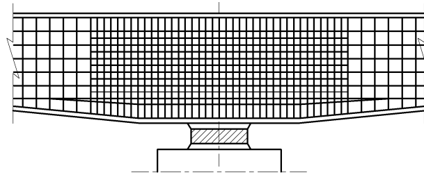
그림 4.11.8 중간받침점 부근에서의 복부 가외철근의 배치 예
