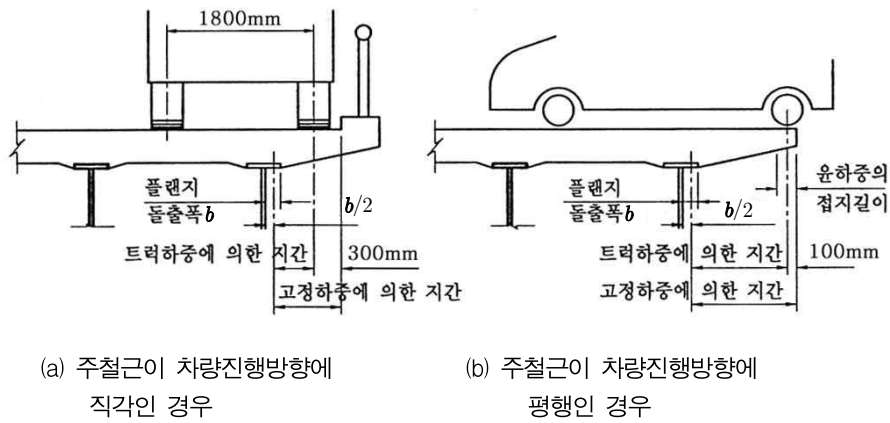
그림 3.6.2 캔틸레버판의 지간
