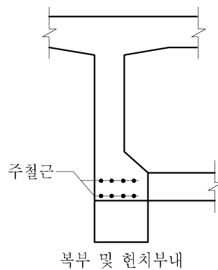
그림 4.10.6 주철근의 배치
