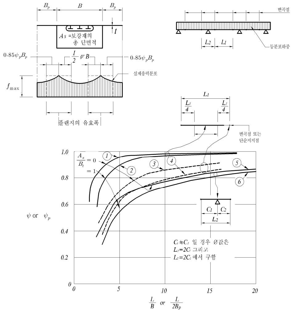
그림 3.6.6 바닥강판의 유효폭
