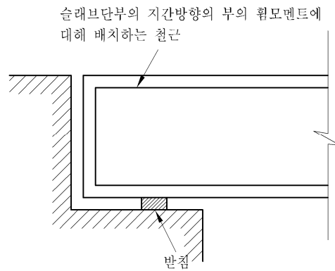
그림 4.8.10 슬래브 단부에서의 경간방향의 철근 배치
