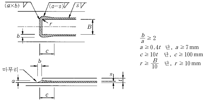
그림 3.8.2 부등치수의 연속필릿용접
