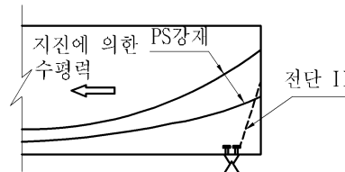
(가) 단받침점을 고정받침부로 하는 경우
