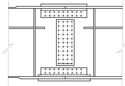
그림 3.8.6 수평보강재의 생략
