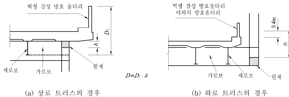
그림 2.1.3 2주구 트러스의 바닥판 총높이 D
