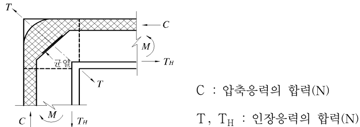
그림 4.12.10 내측인장 휨모멘트에 의한 절점부의 균열
