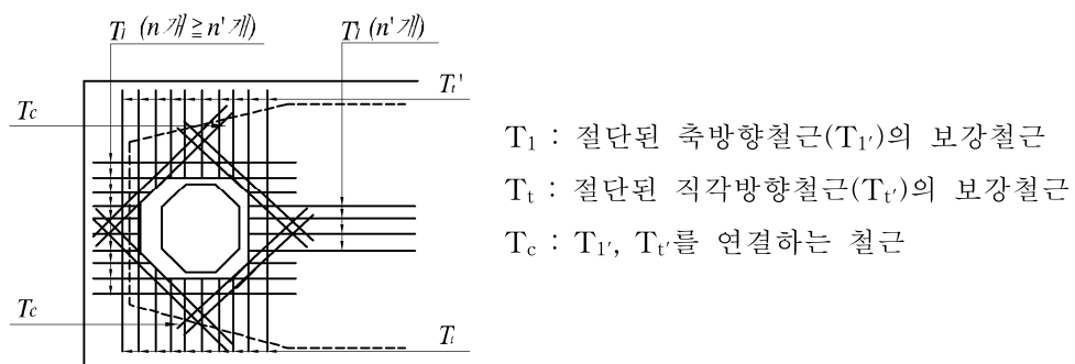
그림 4.10.7 하부플랜지 개구부 구조의 한 예
