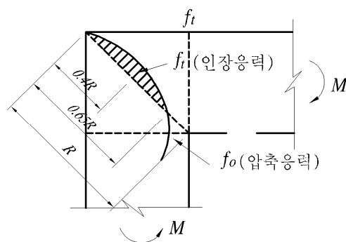
그림 4.12.7 외측인장 휨모멘트가 작용한 경우의 응력분포
