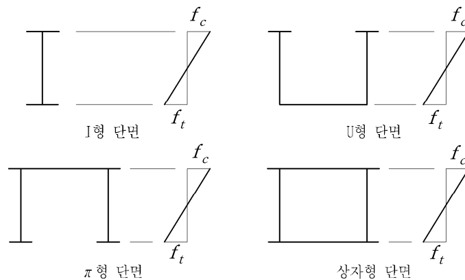
그림 3.3.1 단면의 분류
