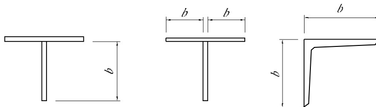
그림 3.4.3 자유돌출폭
