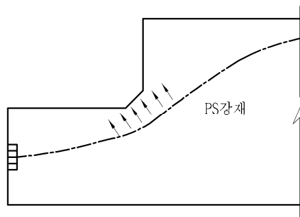
그림 4.15.5 엇갈림부의 PS강재의 배치
