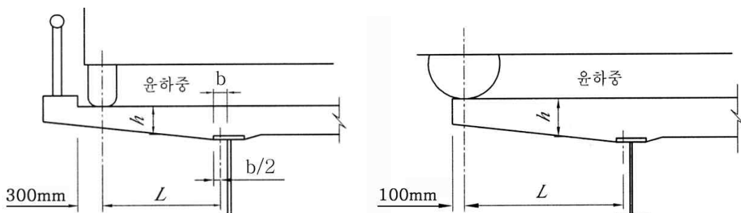
(a) 주철근이 차량방향에 직각인 경우 (b) 주철근이 차량방향에 평행인 경우
