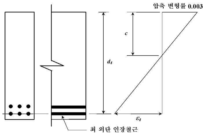
그림 4.4.1 변형률 분포 및 순인장변형률
