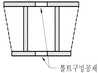
그림 3.14.8 거더구조
