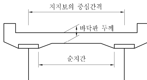
그림 3.6.1 단순판의 지간
