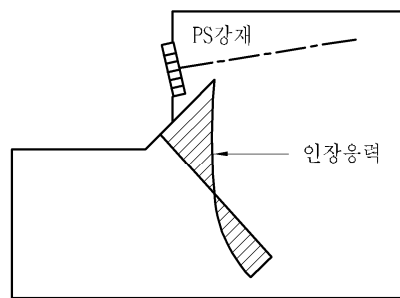
그림 4.15.4 도려낸 부분에서의 인장응력
