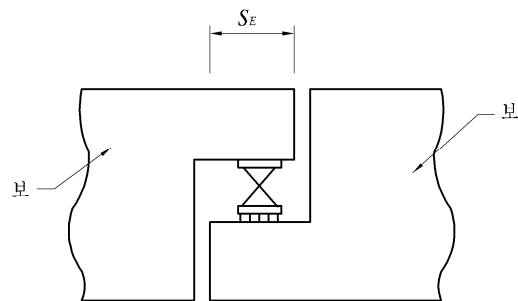
그림 4.15.2 보의 엇갈림길이
