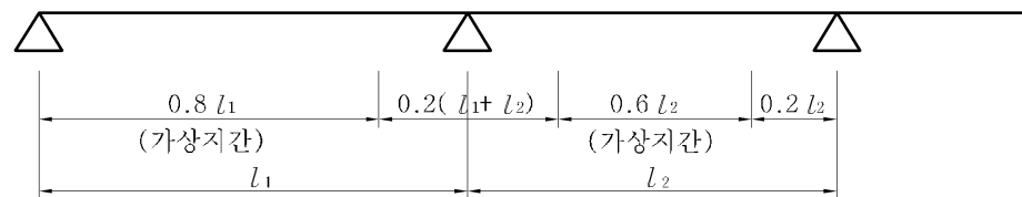
그림 4.11.2 연속슬래브교의 가상경간
