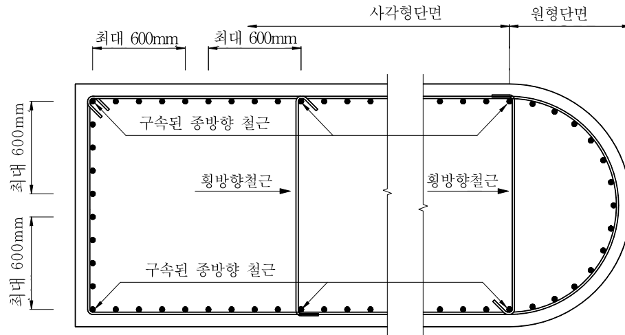
그림 4.3.6 띠철근으로 횡지지된 기둥단면(비내진)
