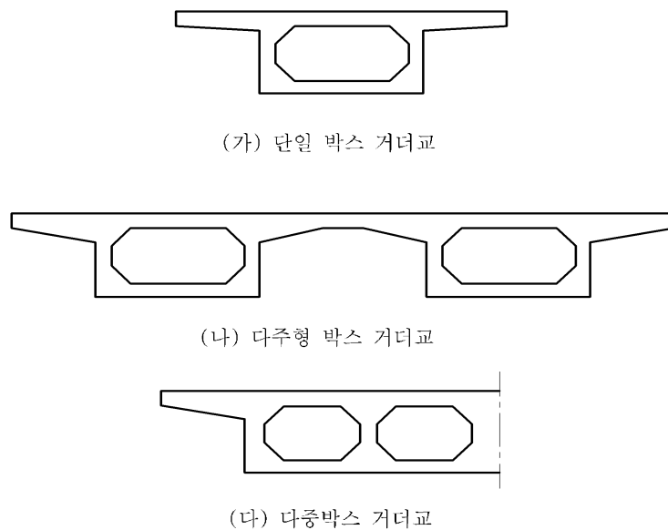
그림 4.10.1 박스거더교의 기본 단면 형상
