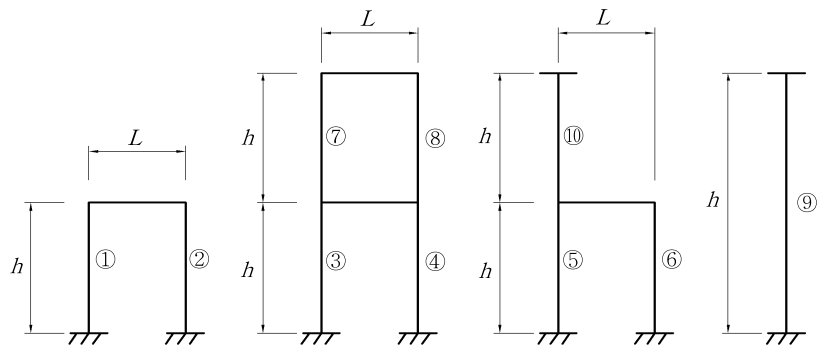
그림 3.14.11 라멘의 부재길이
