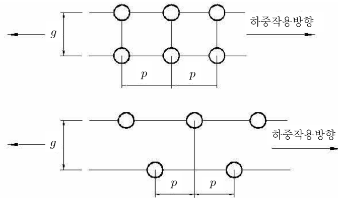
그림 3.5.6 볼트의 피치와 간격
