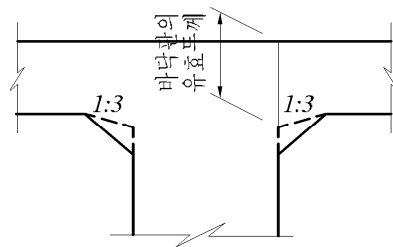
그림 4.7.4 현치부근 바닥판의 유효두께
