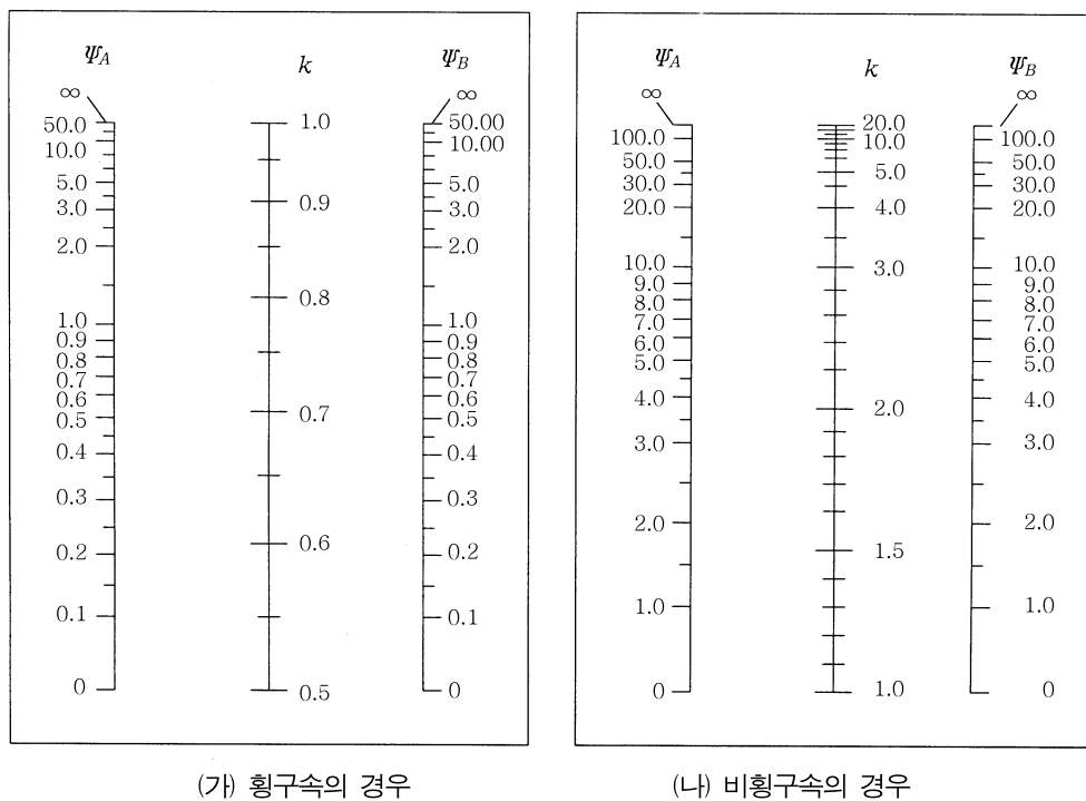
그림 4.4.2 압축부재의 유효길이계수
