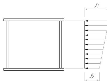
그림 3.4.2 압축과 휨에 의한 연응력
