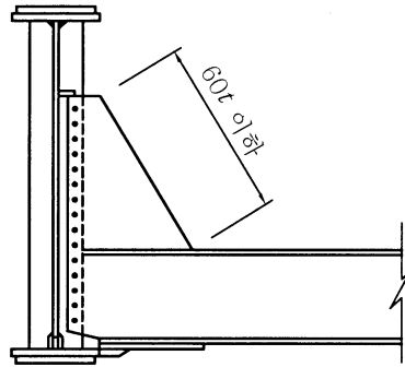
그림 3.8.8 니브레이스의 자유변
