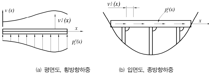
그림 6.5.2 횡방향 및 종방향으로 등가하중을 받는 교량 상판
