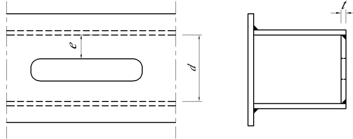
그림 3.4.7 구멍 뚫린 판
