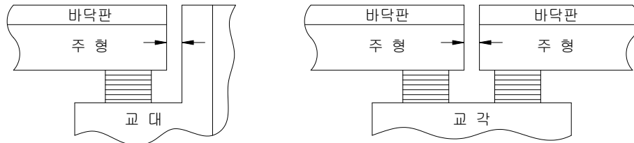
그림 6.4.2 교량의 여유간격
