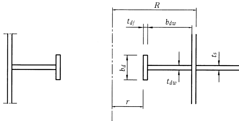
그림 3.14.5 원형기둥의 다이어그램
