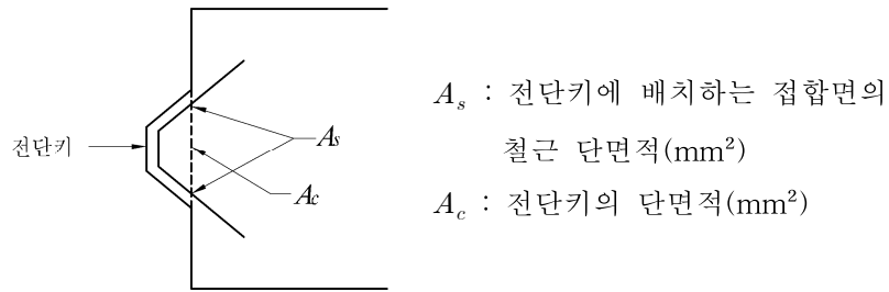
그림 4.15.7 전단키의 구조
