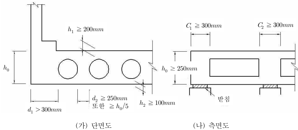
그림 4.8.3 속빈 슬래브교의 단면 최소치수
