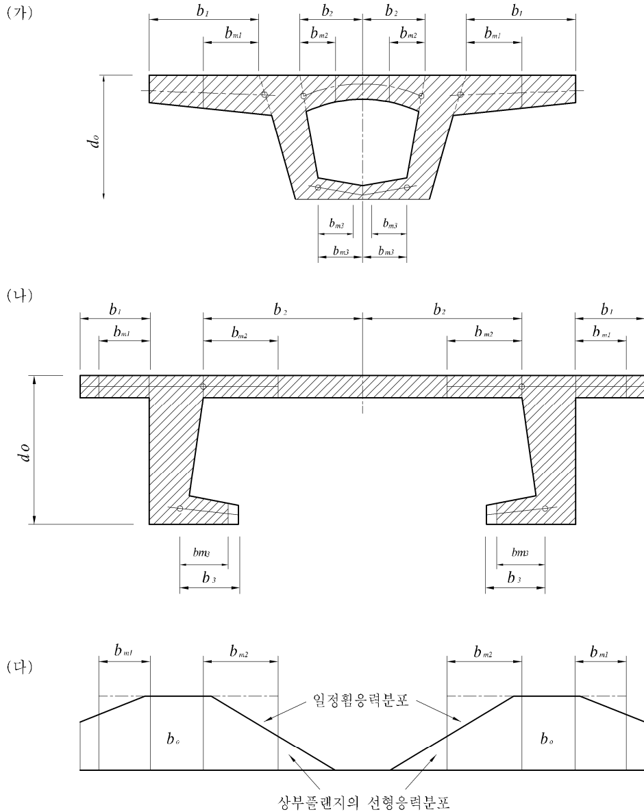
그림 4.15.9 휨과 전단해석을 위한 횡단면과 유효플랜지 폭
