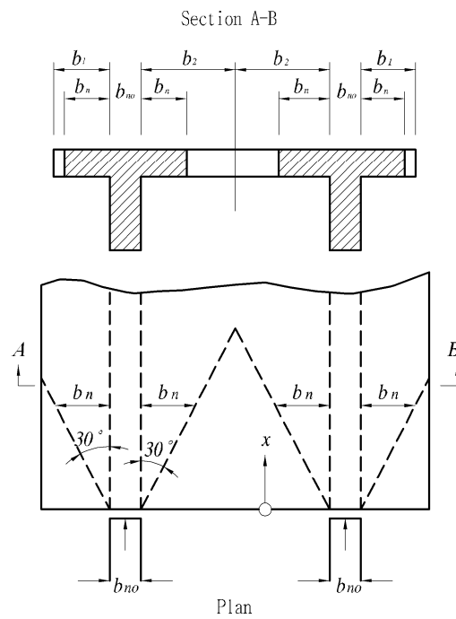
그림 4.15.12 수직력에 대한 유효플랜지폭( b_n )
