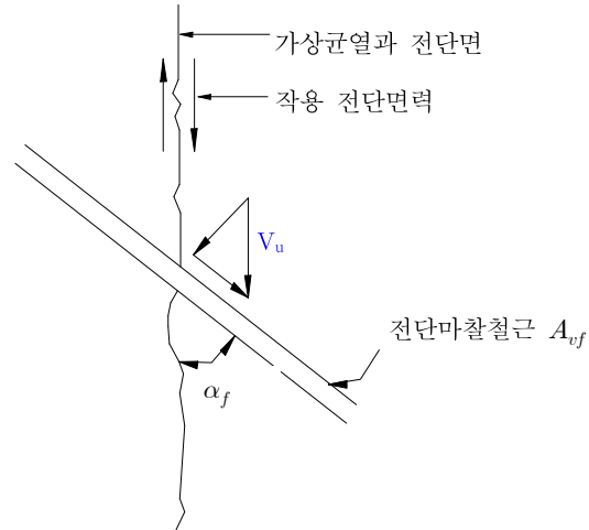
그림 4.4.3 균열과 전단마찰철근
