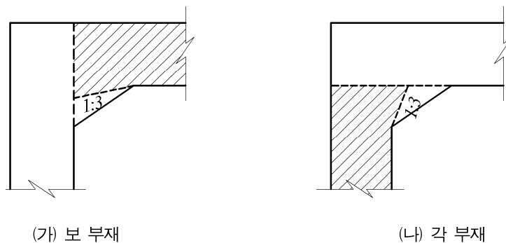
그림 5.4.2 헌치의 유효부분
