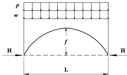
그림 3.11.1 면외좌굴의 조사에 사용되는 재하상태
