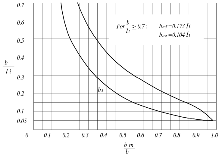
그림 4.15.11 유효플랜지폭 계수
