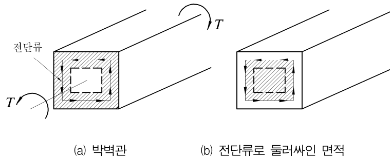
그림 4.4.5 박벽관
