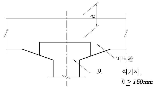
그림 4.14.1 보를 바닥판에 매립할 경우의 바닥판의 최소두께
