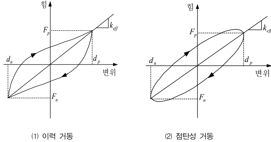
그림 6.9.1 지진격리받침의 유효강성 및 지진격리시스템의 등가감쇠비 산출
