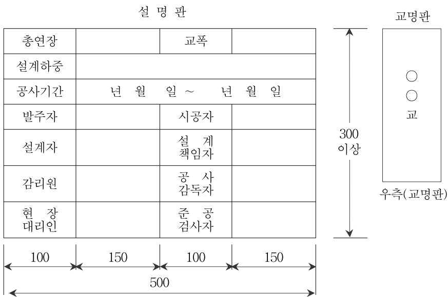
그림 2.5.1 교명판
