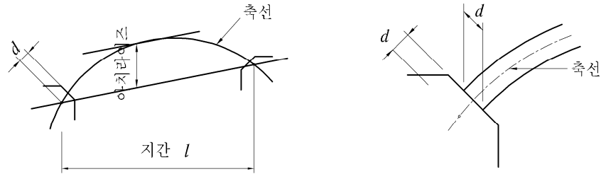
그림 4.13.3 고정아치인 경우의 기초고정도를 고려한 경간
