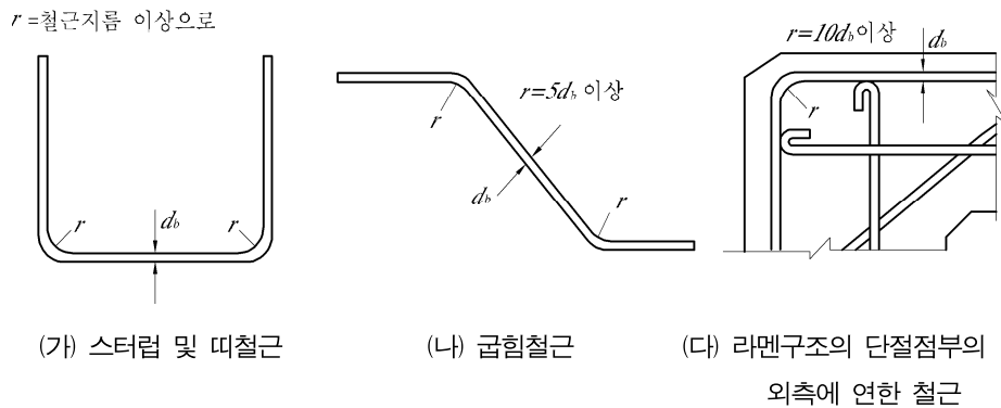
그림 4.3.2 철근의 구부림 내면반지름
