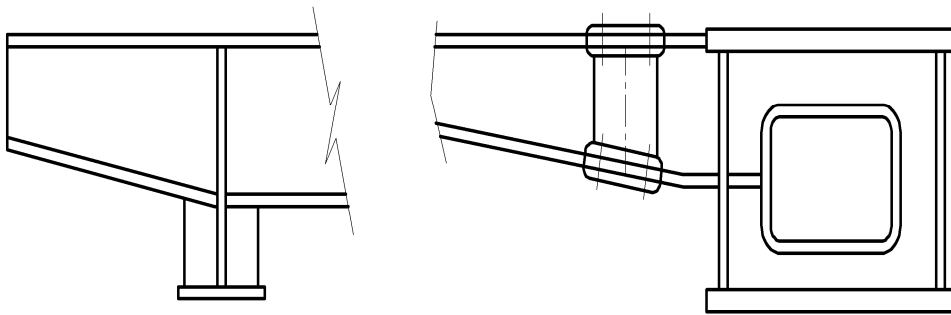
그림 3.7.4 바닥틀 브래킷의 연결방법의 예
