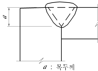
그림 3.5.2 부분용입 그루브용접의 두께
