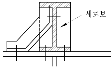
그림 3.7.3 세로보와 가로보의 연결방법의 예
