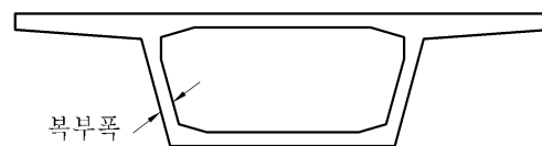
그림 4.10.2 전단응력의 계산에 쓰이는 복부의 폭
