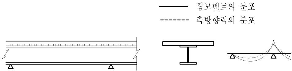
그림 3.9.1 전단연결재의 배치
