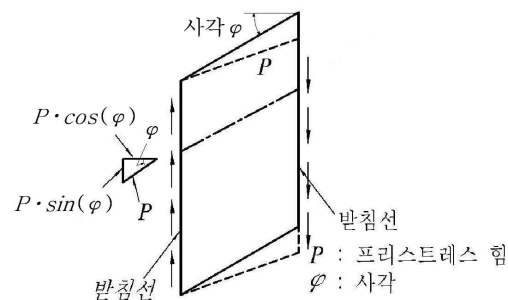
그림 4.8.9 프리스트레스 힘의 분포에 따른 슬래브의 변형
