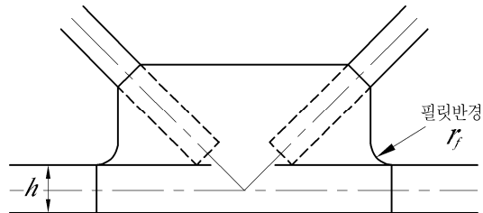
그림 3.10.5 필릿
