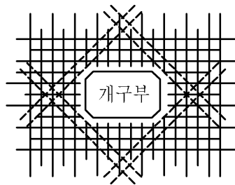
(나) 개구부 근처의 가외철근
