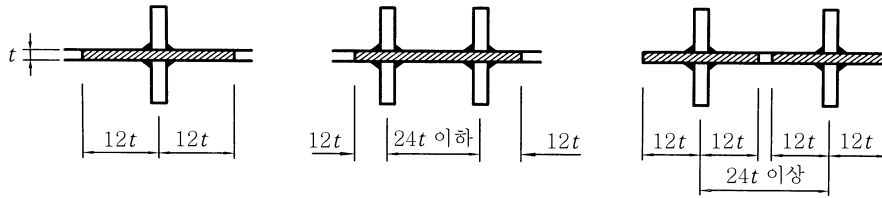
그림 3.8.7 하중집중점 보강재의 유효단면적
