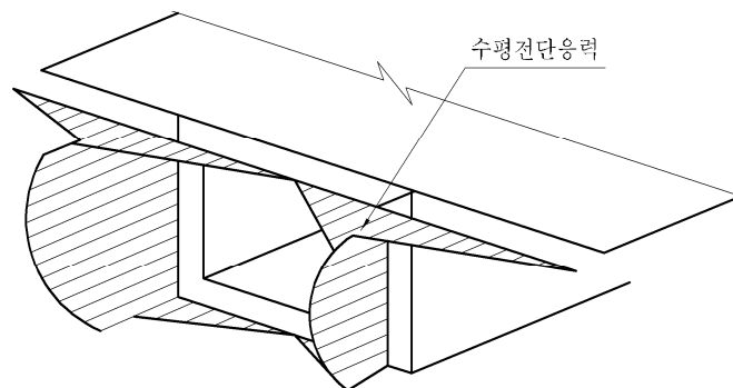
그림 4.10.3 플랜지에 생기는 수평전단응력의 분포
