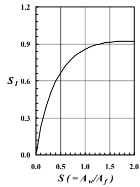
그림 3.14.3 전단지연의 추정도
