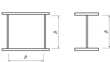
그림 3.4.1 판의 고정연 사이의 거리 b
