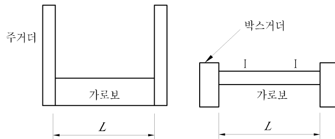
그림 3.7.2 가로보의 지간
