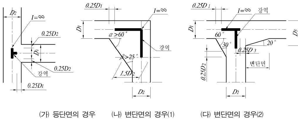
그림 4.12.3 라멘교 절점부에서의 강역
