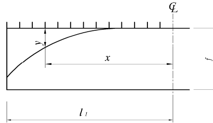
그림 4.13.2 아치축선의 좌표
