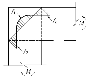
그림 4.12.9 내측인장 휨모멘트가 작용하는 경우의 응력분포
