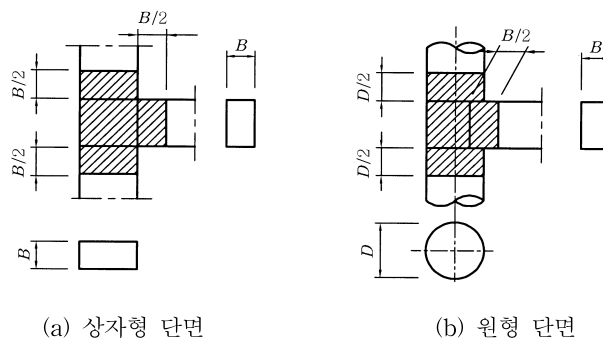
그림 3.14.10 모서리부 범위
