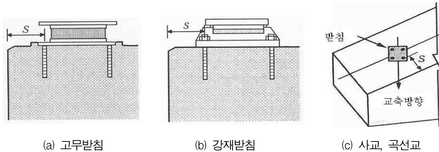
그림 5.4.1 연단거리, S
