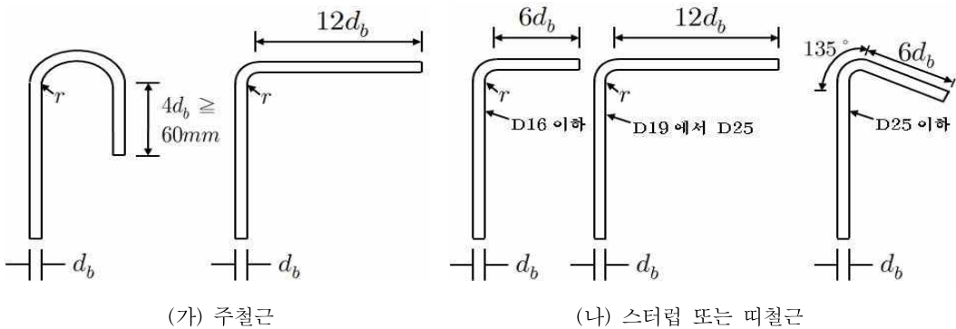
그림 4.3.1 표준갈고리의 형태
