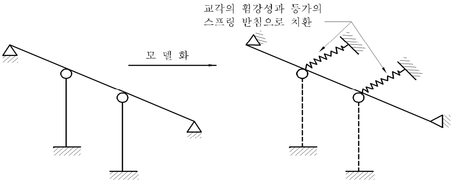
그림 4.11.3 교축직각방향의 검토 모델의 예
