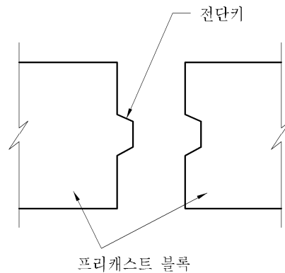
그림 4.15.6 전단키
