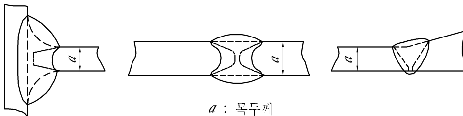
그림 3.5.1 전단면용입 그루브용접의 목두께
