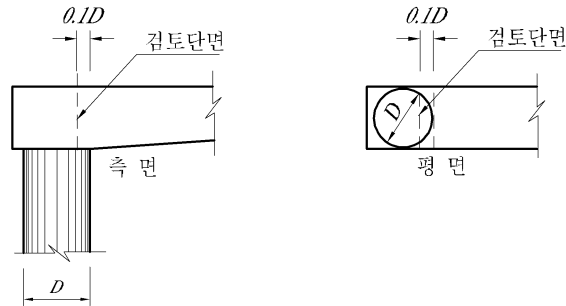
그림 4.12.6 기둥 단면이 원형인 경우의 설계 단면
