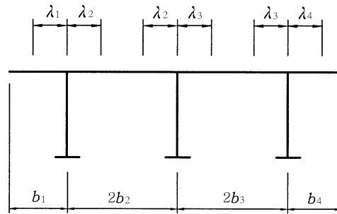
그림 3.8.3 플랜지의 유효폭
