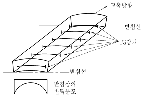
그림 4.8.7 받침선상의 반력 분포
