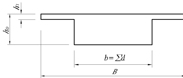
(나) 가상 T형단면
