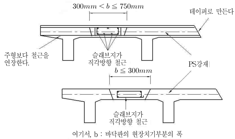
그림 4.9.2 바닥판을 현장타설하는 경우의 구조상세
