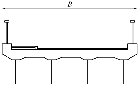
그림 2.1.2 교량 총폭 B
