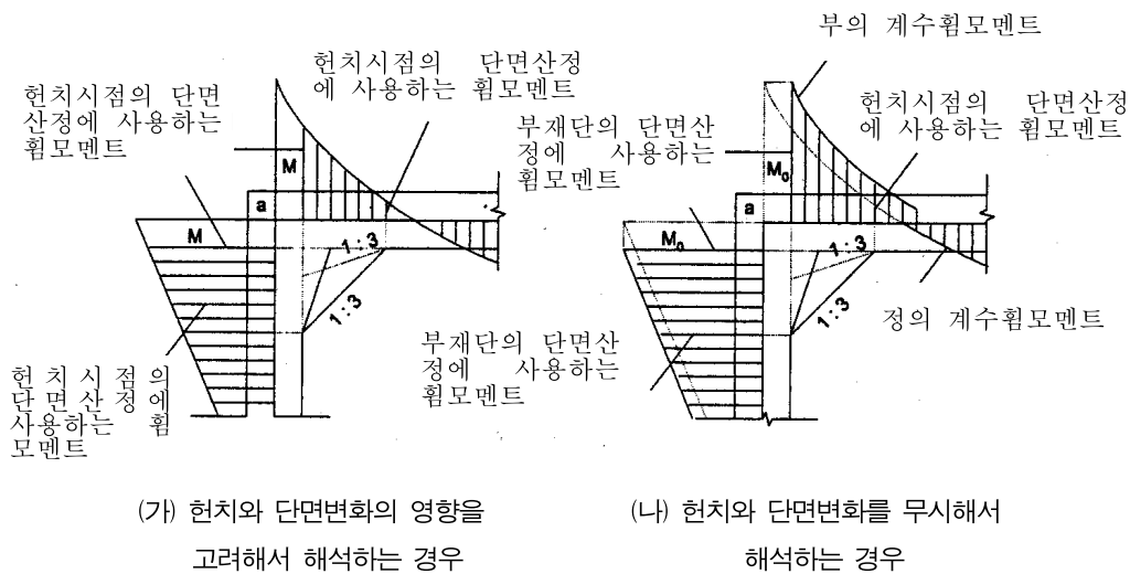
그림 5.4.3 라멘부재 절점부의 설계휨모멘트
