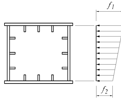
그림 3.4.5 보강된 판의 연응력
