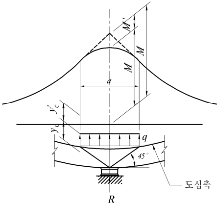
그림 4.11.4 중간받침점상의 설계휨모멘트
