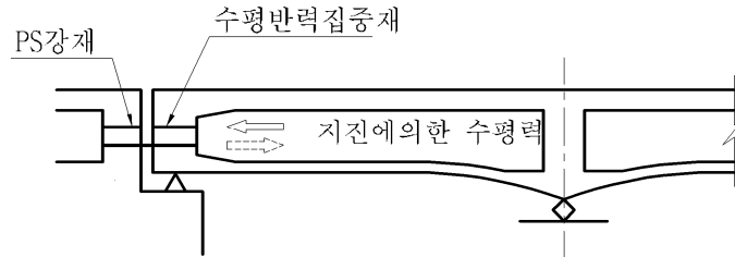
그림 4.11.7 단발침점의 격벽으로부터 직접 교대에 수평반력을 전달하는 경우
