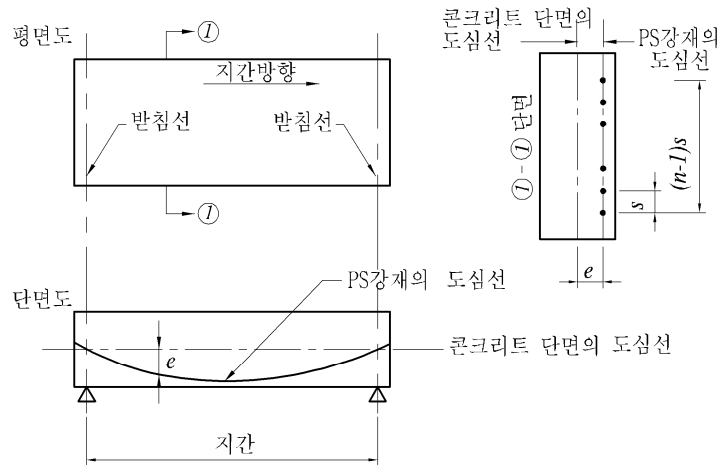
그림 4.8.6 PS강재의 배치
