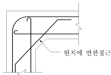
그림 4.3.3 현치에 의한 철근
