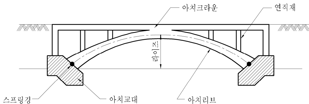
그림 4.13.1 아치교 각부의 명칭
