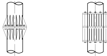
(a) 리브가 붙은 플랜지 연결 (b) 겹플랜지 연결
