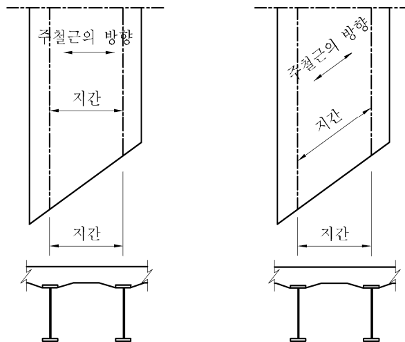
그림 3.6.3 사교의 바닥판의 지간
