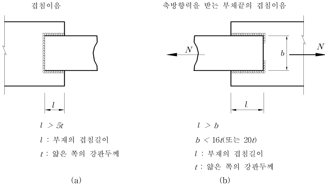
그림 3.5.4 겹침이음의 필릿용접
