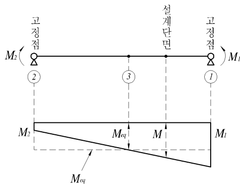
그림 3.3.2 양단 사이에서 휨모멘트가 직선적으로 변화하는 경우
