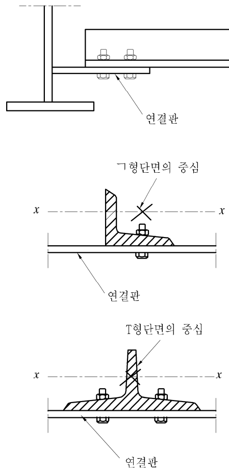
그림 3.4.8 ㄱ형 및 T형 단면을 가진 압축부재
