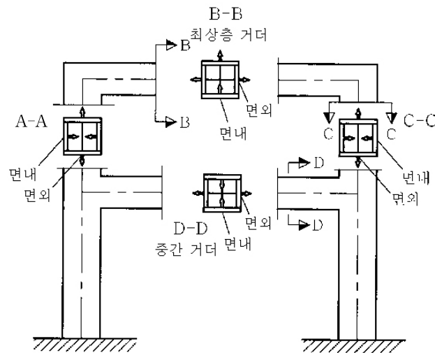
그림 3.14.9 판두께 변화의 방향
