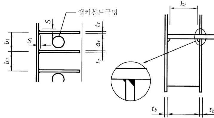
그림 3.14.6 리브의 설치
