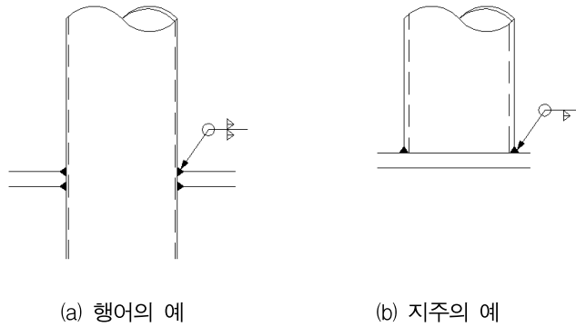
그림 3.13.8 단일 강관부재의 단부의 용접방법( d \leq l/25 )
