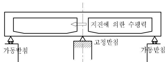
(나) 중간교각에 고정받침부를 설치하는 경우
