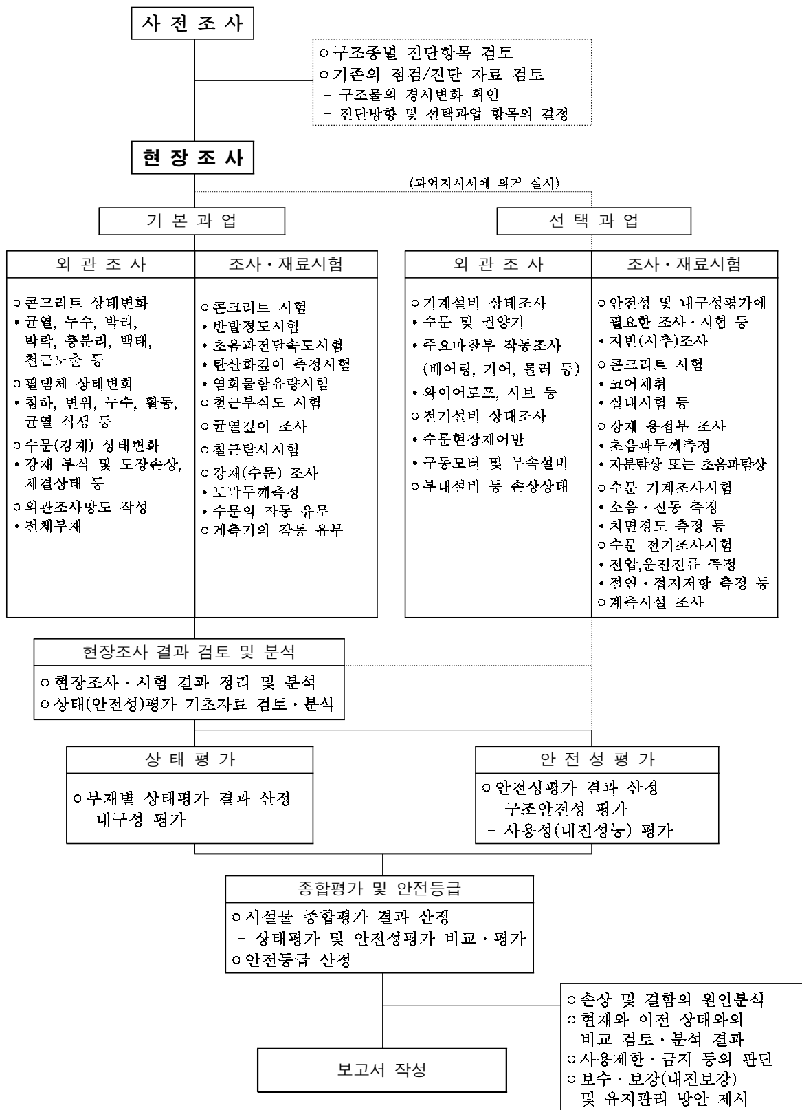
[그림 4.1] 정밀안전진단 흐름도
