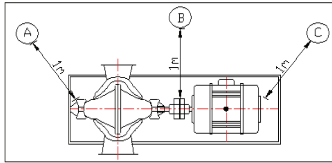
[그림 6.16] 펌프소음의 측정위치도
