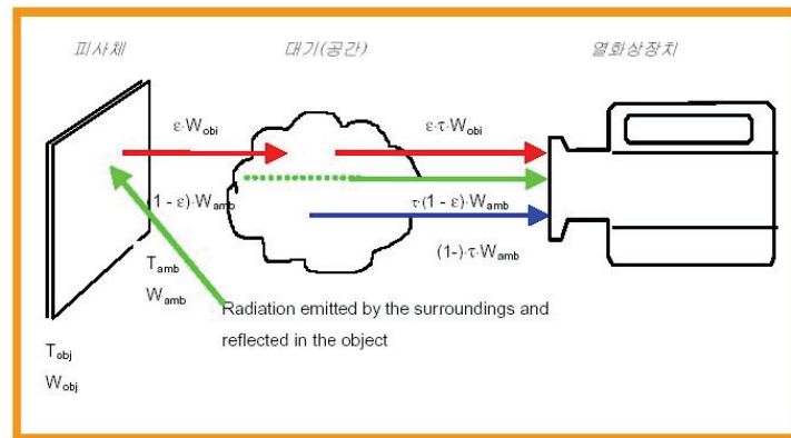
[그림 6.17] 적외선 열화상 카메라에 의한 온도측정
