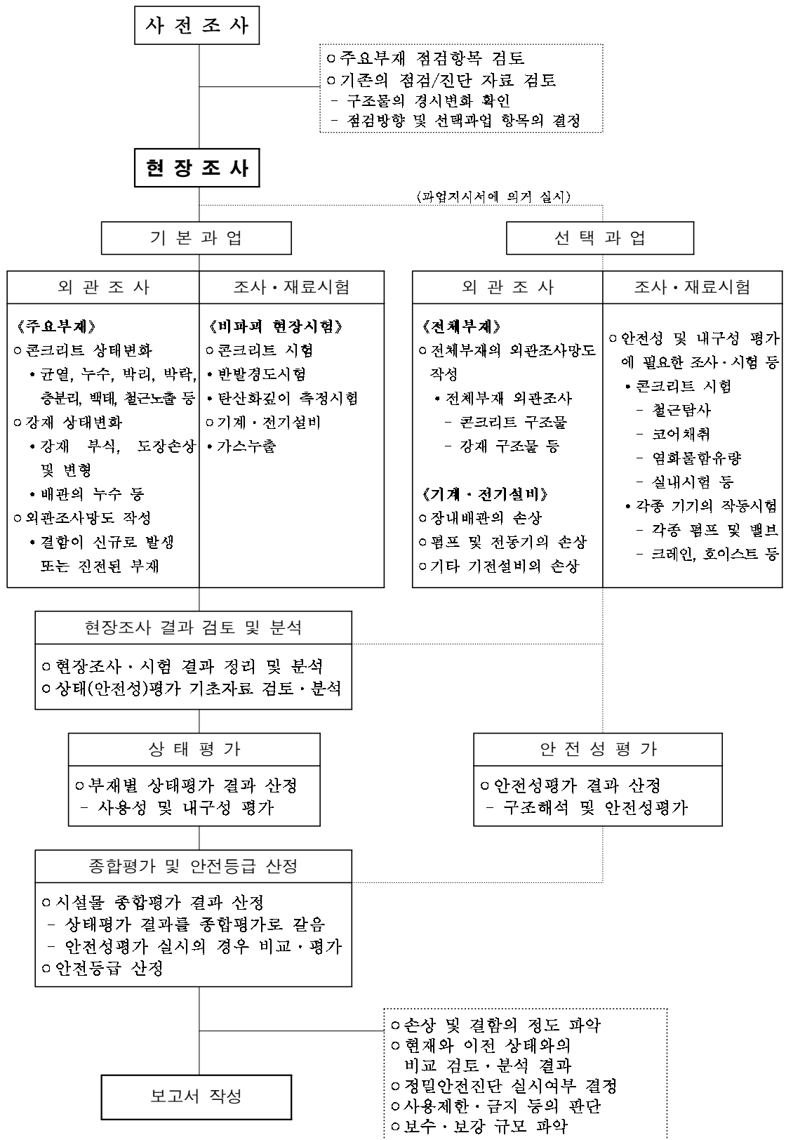
[그림 3.2] 정밀점검 및 긴급점검 흐름도
