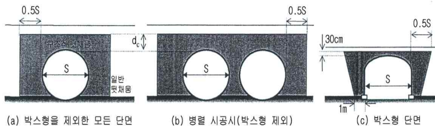
그림 5-2-12 흙쌓기부에 지중강판 구조물을 설치할 경우 구조적 뒤채움 영역
