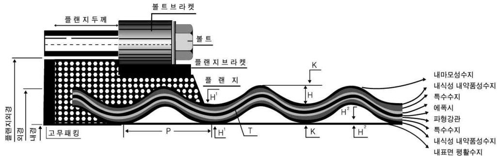
그림 5-2-6 수지파형강관 단면도(평활형)
