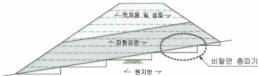
그림 5-2-15 종단경사가 있는 구조물의 뒤채움
