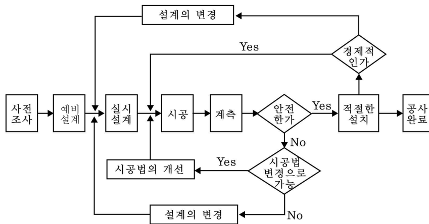
그림 7-10-1 계측관리 계획도
