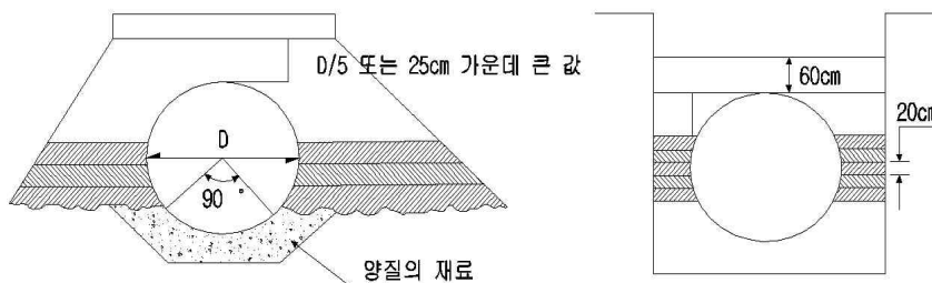
그림 5-2-9 흙쌓기와 뒤채움 기준
