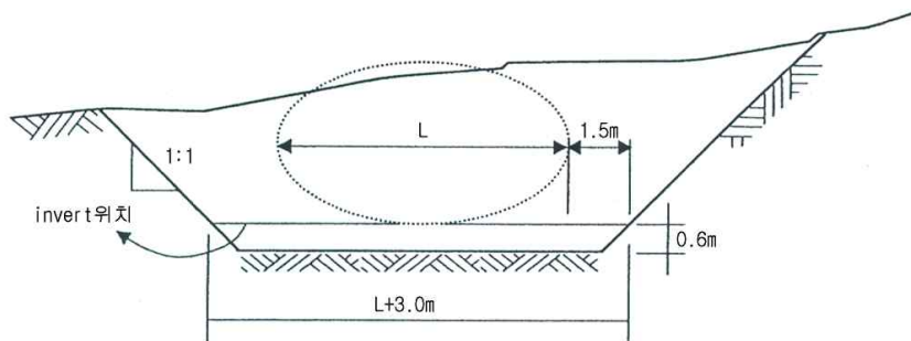
그림 5-2-13 기초지반을 굴착하여 설치하는 경우 구조적 뒤채움 영역
