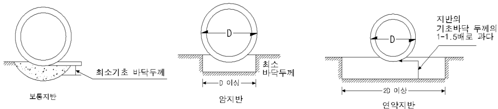
그림 5-2-8 지반에 따른 기초폭
