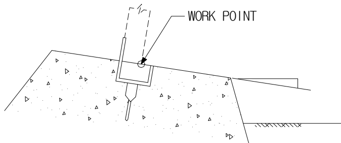
그림 5-2-16 베이스채널을 이용한 기초연결부
