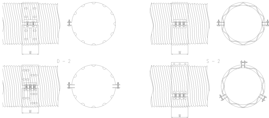
그림 5-2-3 커플링 밴드 형상
