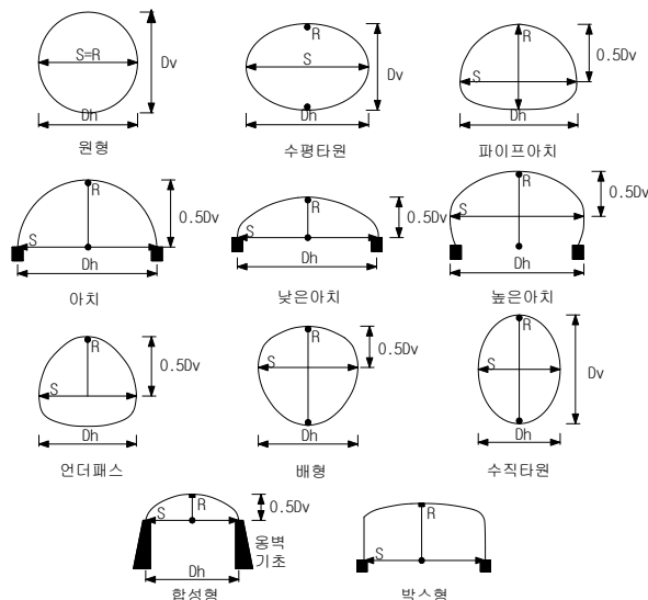
그림 5-2-17 파형강판구조물 적용단면 (S = 폭-span, R = 높이-rise)
