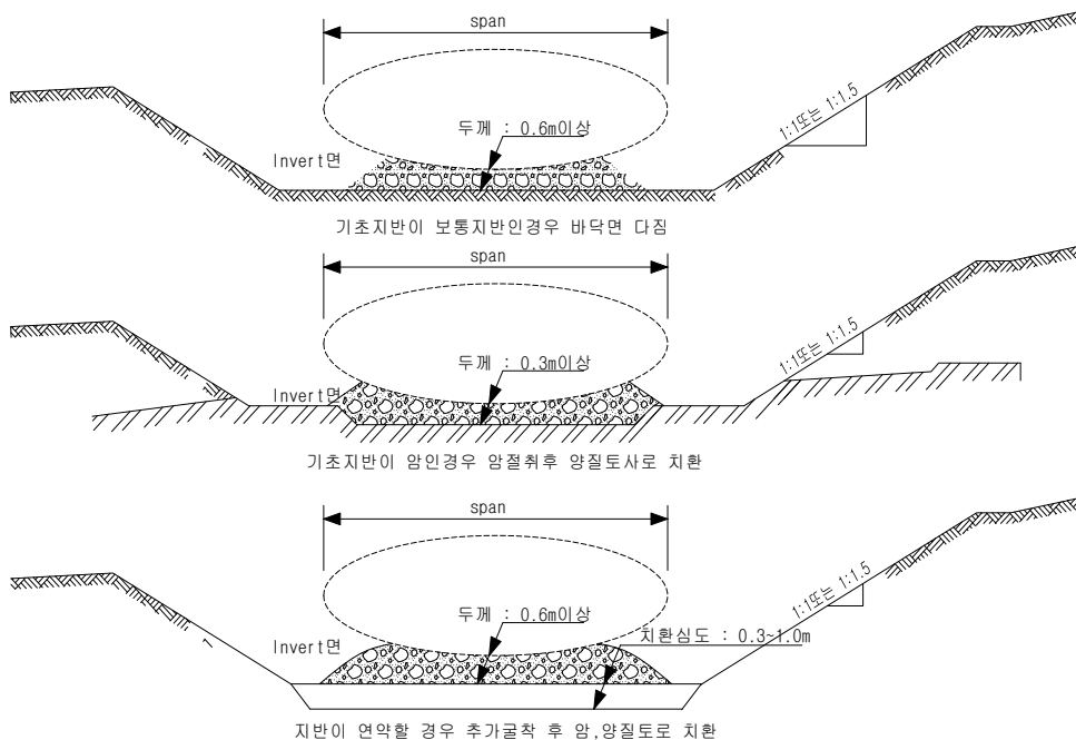
그림 5-2-10 기초지반 조건에 따른 처리방법 예
