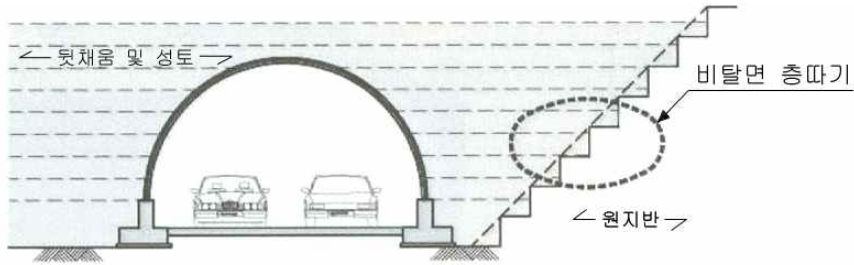
그림 5-2-14 흙쌓기·땅깎기부와 접속부 뒤채움
