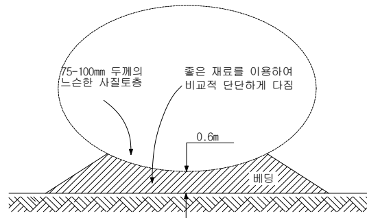
그림 5-2-11 베딩 시공
