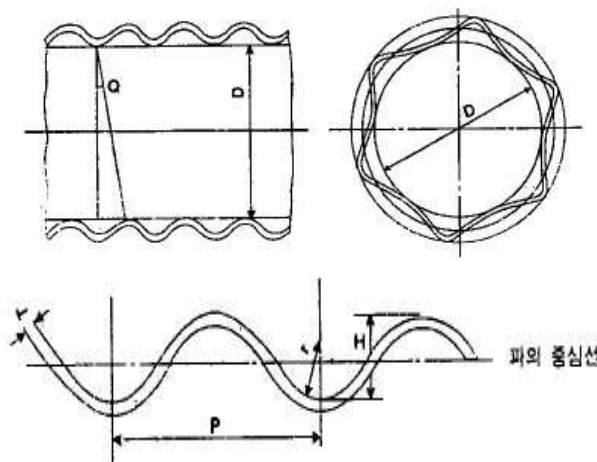
그림 5-2-4 수지파형강관의 단면 모양
