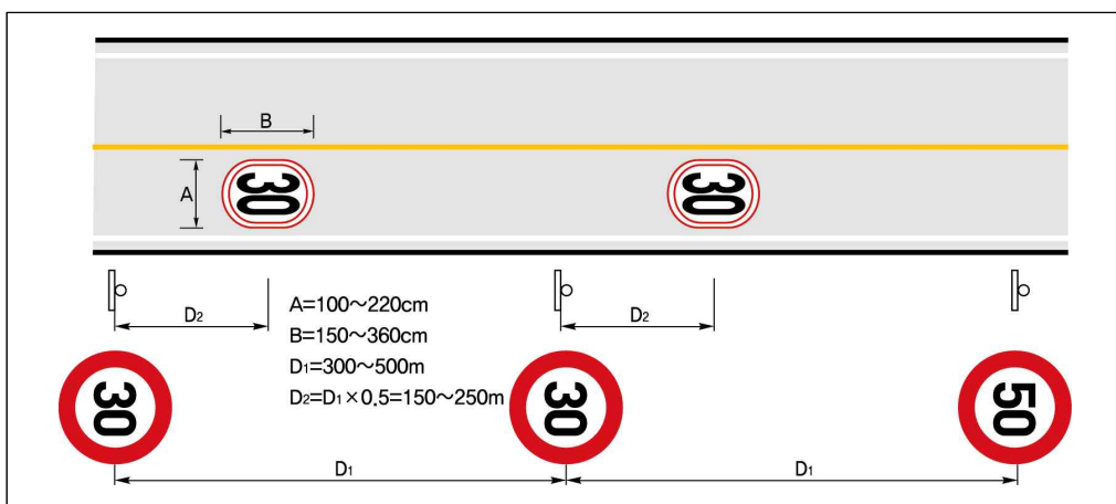
[그림 3-16] 어린이보호구역내 속도제한(518) 표시 설치 예시도
