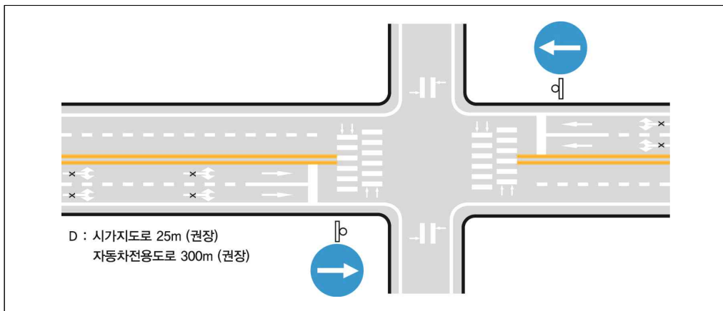
[그림 3-12] 좌우회전금지(513) 표시 설치 예시도
