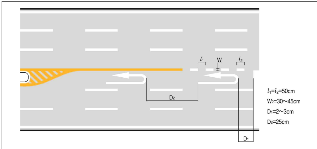
[그림 3-3] 유턴구역선(502) 표시 설치 예시도
