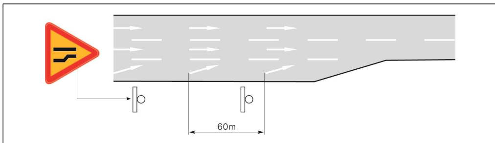
[그림 4-21] 차로변경표시 설치 사례도
