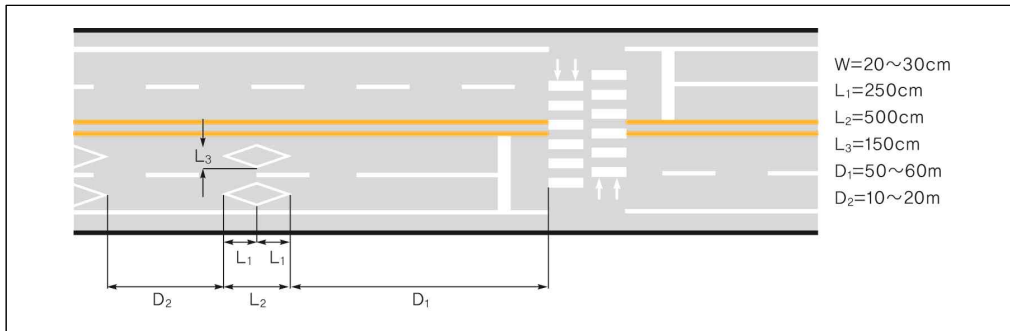
[그림 4-10] 횡단보도예고(529) 표시 설치 예시도
