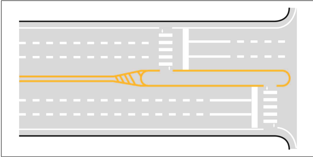
[그림 4-16] 스테거드 횡단보도 설치 예시도
