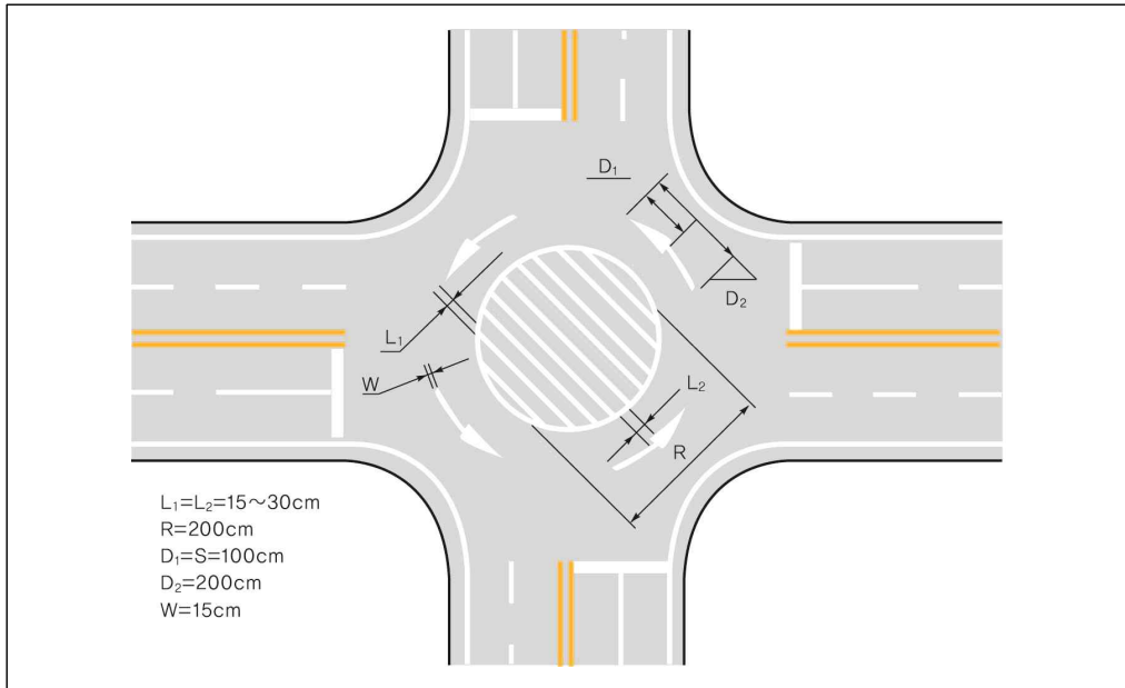
[그림 4-7] 유도(526) 표시 설치 예시도(1)
