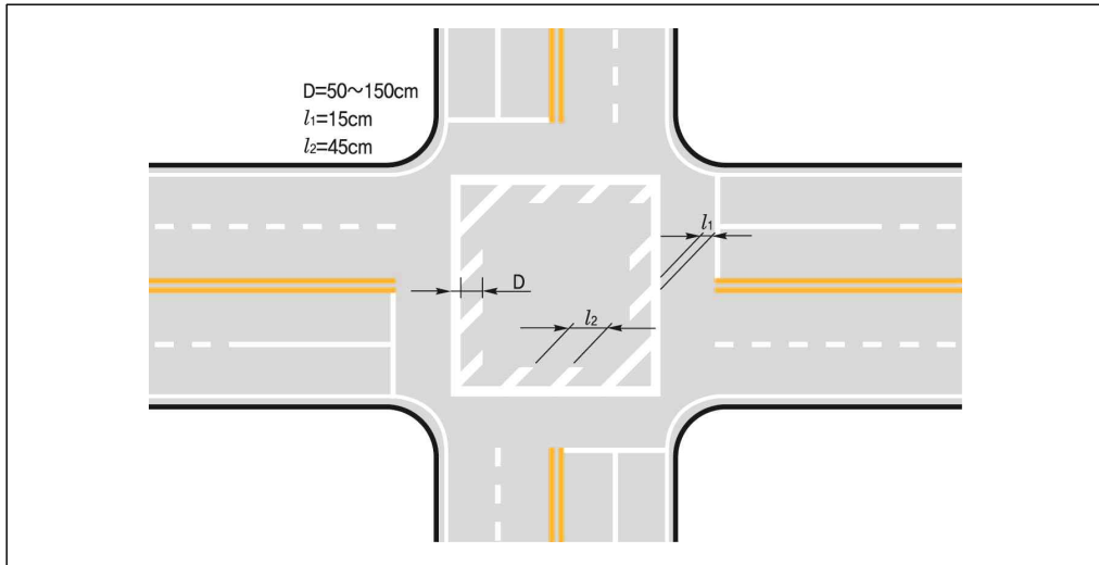
[그림 3-23] 정차금지대(524) 표시 설치 예시도
