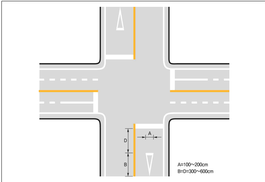
[그림 3-19] 교차로에서 양보표시(522) 표시 설치 예시도
