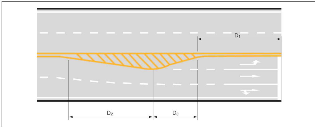
[그림 4-24] 좌회전 전용차로 설치 예시도
