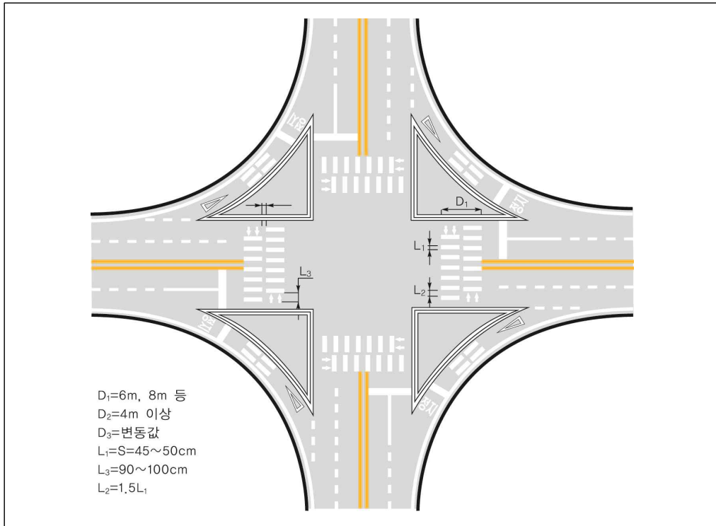
[그림 4-14] 도류화 횡단보도(532) 표시 설치 예시도
