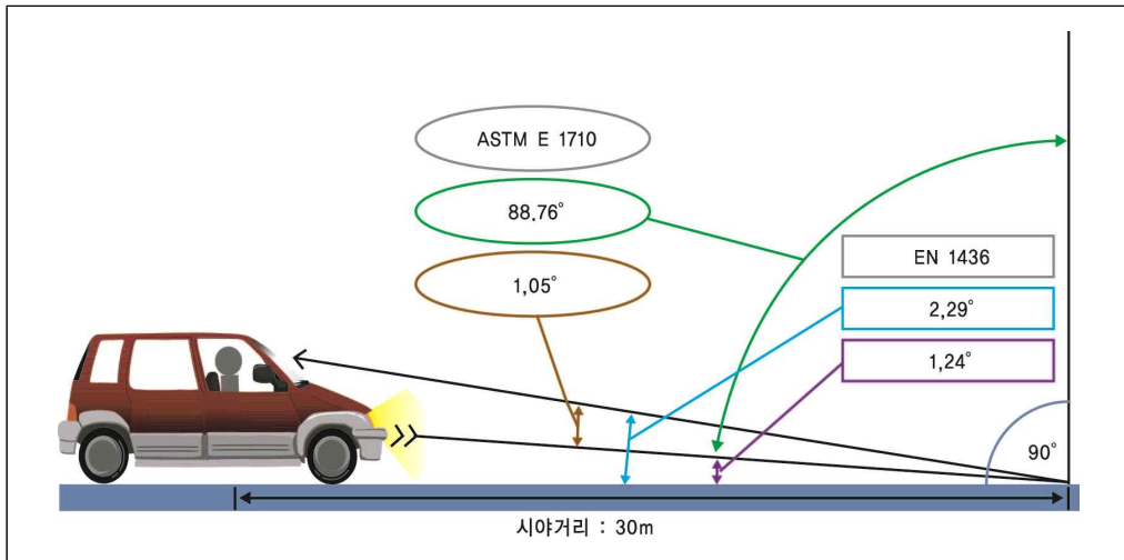
[그림 2-3] 입사각과 관찰각
