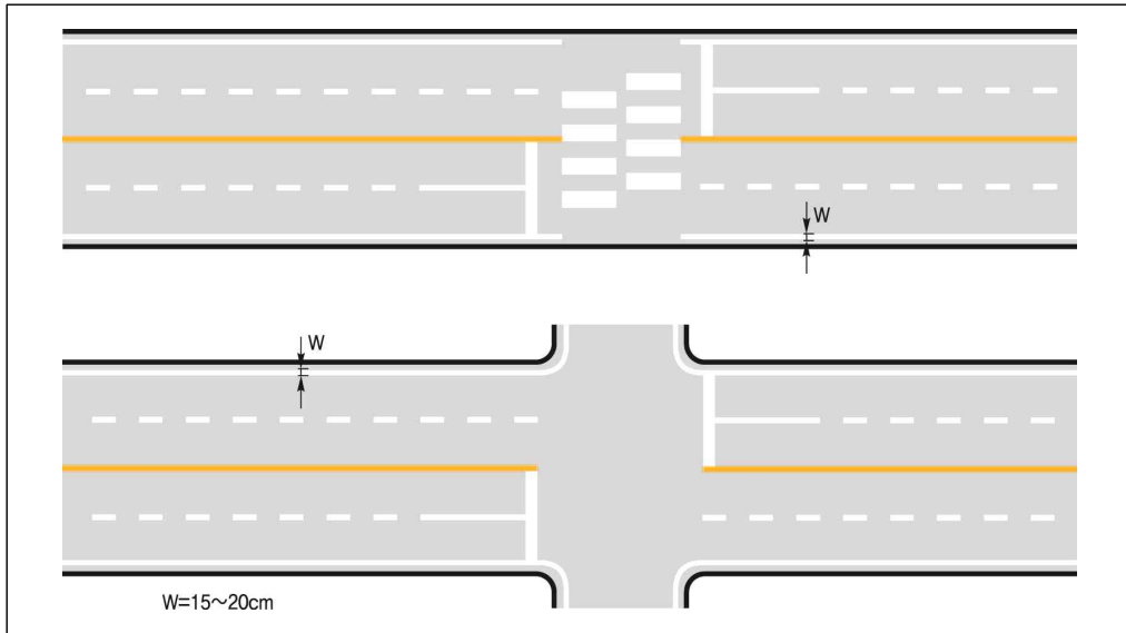
[그림 3-6] 길가장자리구역선(505) 표시 설치 예시도
