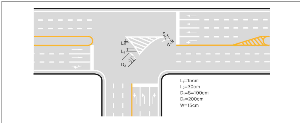
[그림 4-9] 유도(528) 표시 설치 예시도(3)
