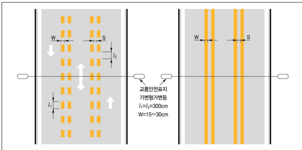
[그림 3-2] 가변차선 표시 설치 예시도
