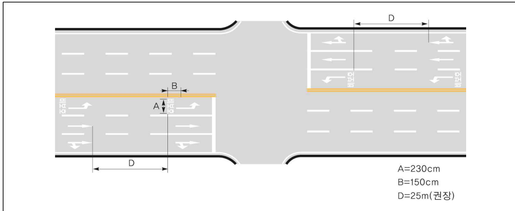
[그림 4-20] 비보호좌회전(542) 표시 설치 예시도
