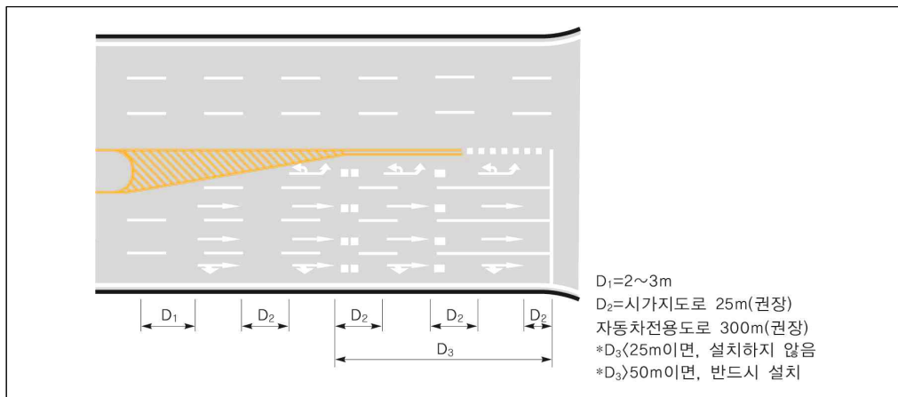
[그림 4-19] 진행방향(537, 538, 539, 538-2, 540, 541) 표시 설치 예시도
