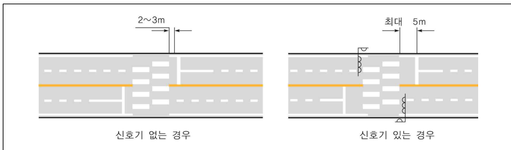
[그림 4-12] 단일로상 횡단보도에서 정지선의 위치
