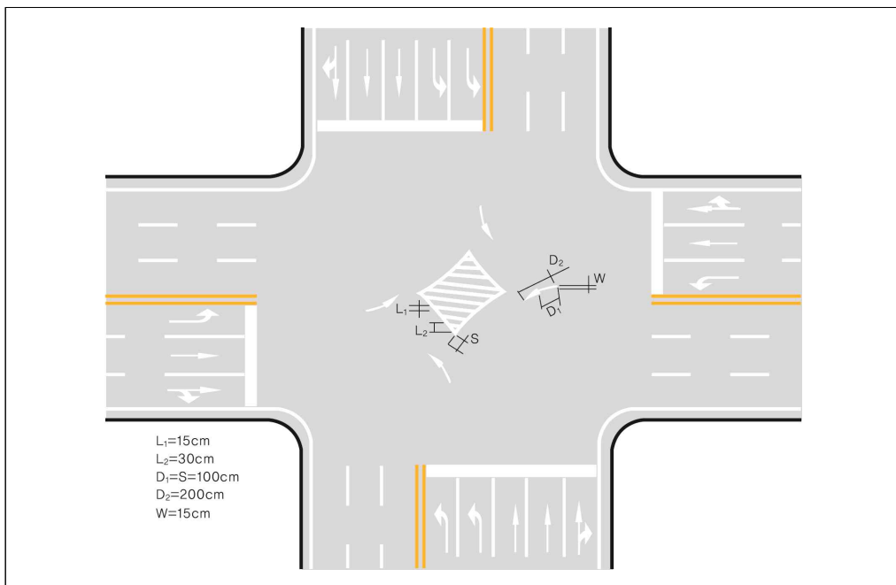
[그림 4-8] 유도(527) 표시 설치 예시도(2)
