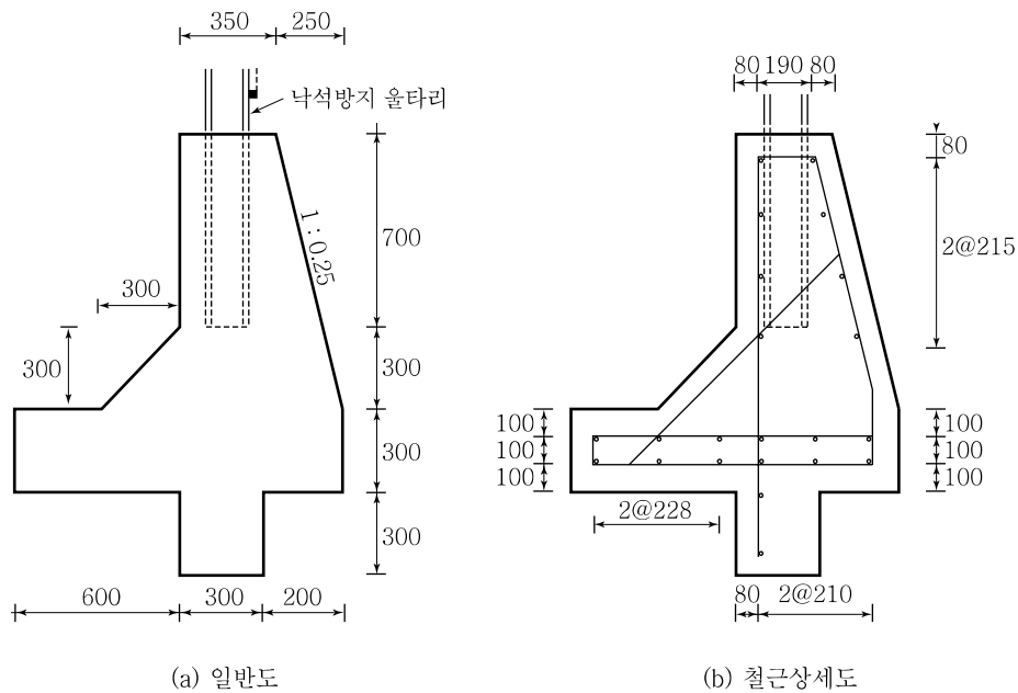
해설그림 22.2 C 형식 옹벽의 단면(H 150×75 지주의 경우)
