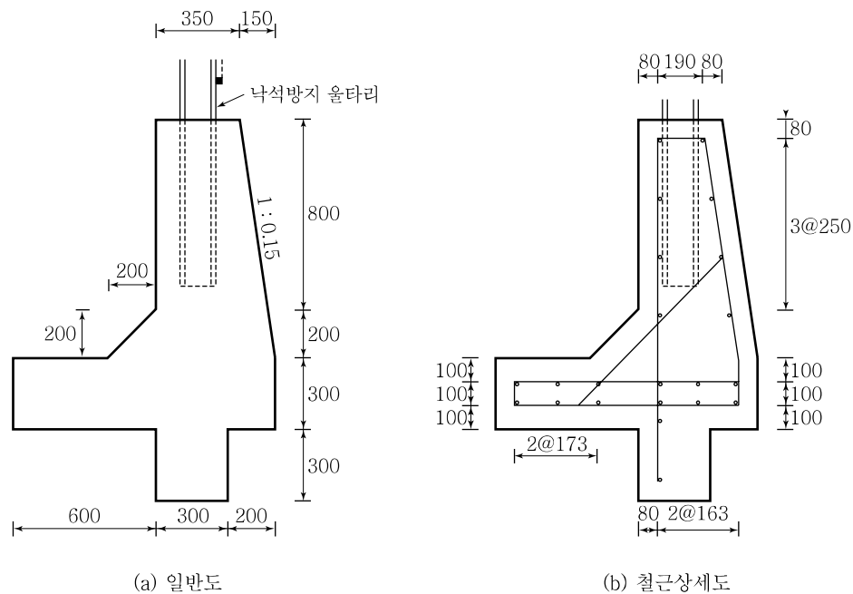
해설그림 22.1 A, B 형식 옹벽의 단면(H 150×75 지주의 경우)
