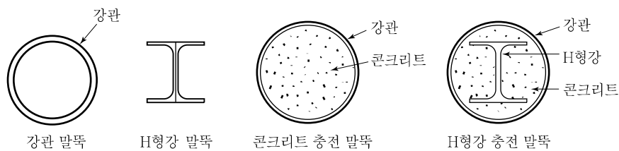
해설그림 9.1 억지말뚝의 재료와 단면 종류
