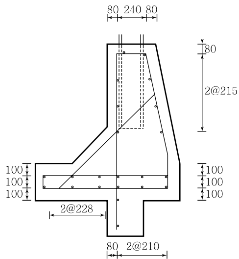
(b) 철근상세도
