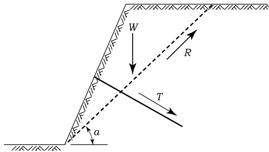
해설그림 7.8 단일 켤레파괴에 대한 안정계산
