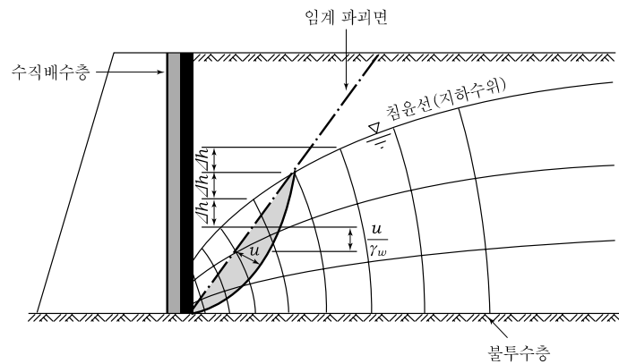
(a) 뒤채움 내부에 지하수가 있는 경우 파괴면에서 작용하는 수압
