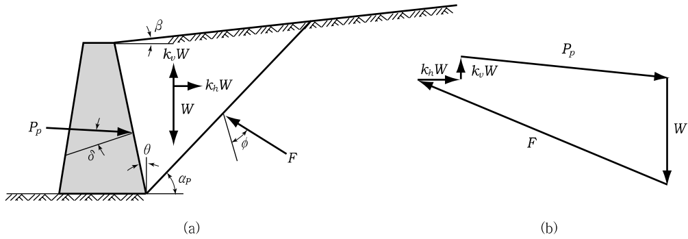
해설그림 10.22 Mononbe-Okabe방법에서 수동췌기에 작용하는 힘
