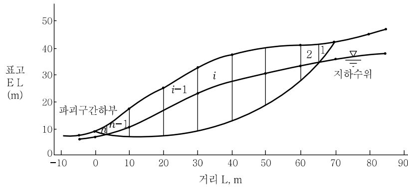
해설그림 9.11 안정해석을 위한 파괴토체 분할도
