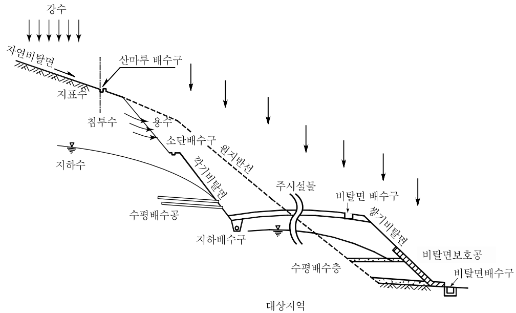
해설그림 18.1 비탈면 지표수 배수시설
