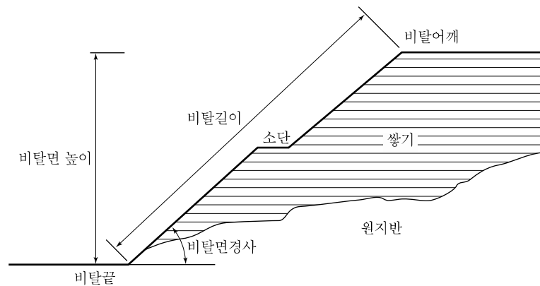
그림 1.9 쌓기비탈면의 단면예
