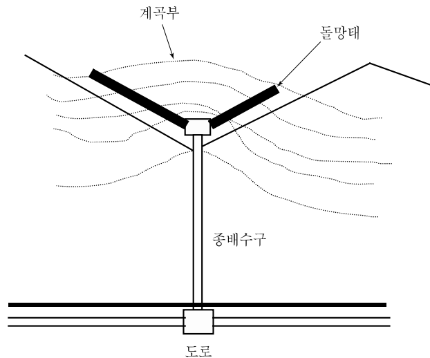
해설그림 18.5 비탈면 계곡부의 배수시설
