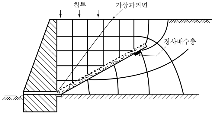
해설그림 10.10 경사배수층을 둔 경우 임계파괴면에서 작용하는 수압
