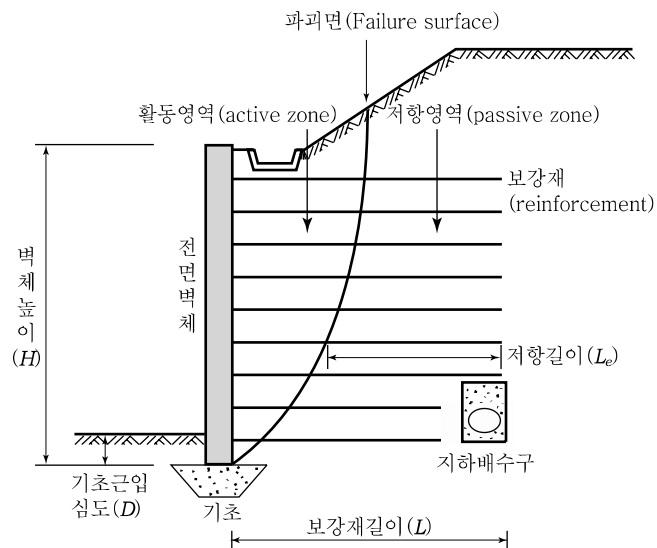
그림 1.7 보강토옹벽의 단면
