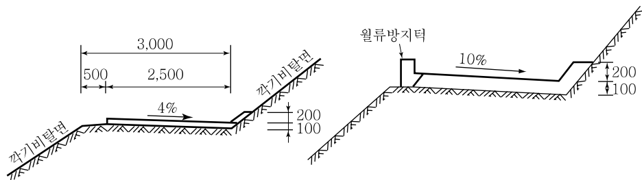
해설그림 18.6 깎기비탈면의 소단배수구 단면 (배수경사 4% 또는 10%)
