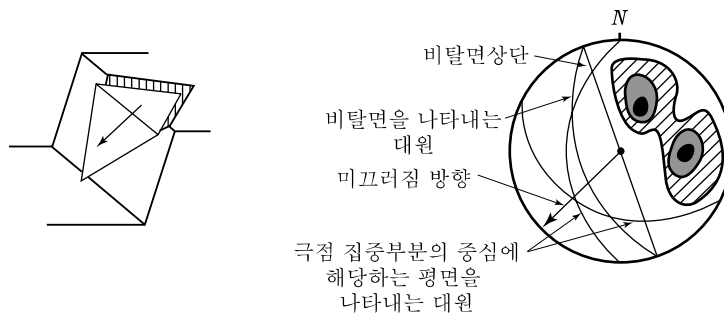
(c) 교차하는 두 불연속면 위에서의 썩기파괴
