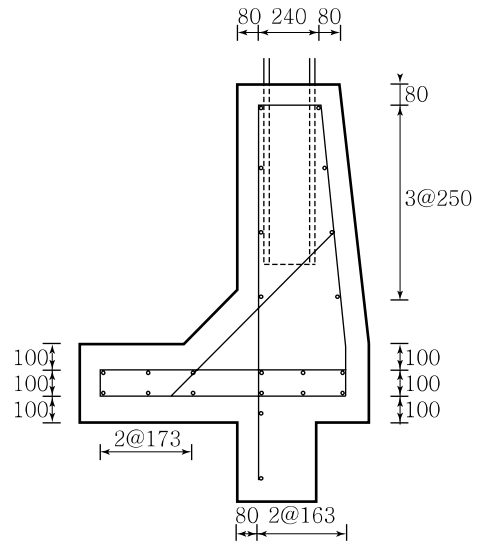
(b) 철근상세도
