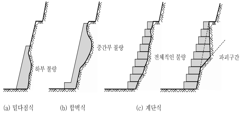
그림 1.1 기대기옹벽의 종류
