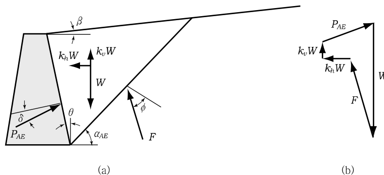
해설그림 10.20 Mononobe-Okabe방법에서 주동췌기에 작용하는 힘
