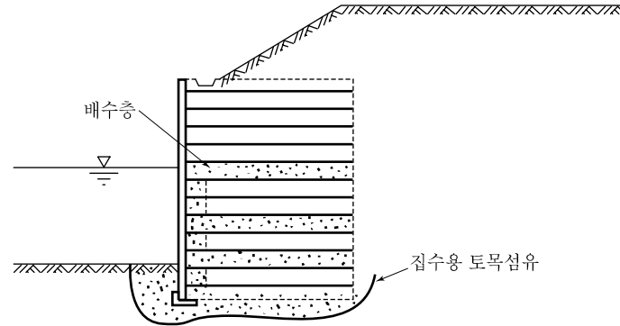
(b) 침수지역 보강토 옹벽의 배수대책 해설그림 11.12 보강토 옹벽의 배수시설 적용예
