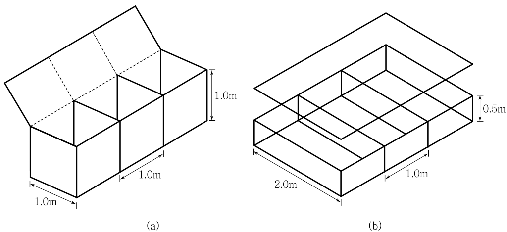
그림 1.4 돌망태의 형태
