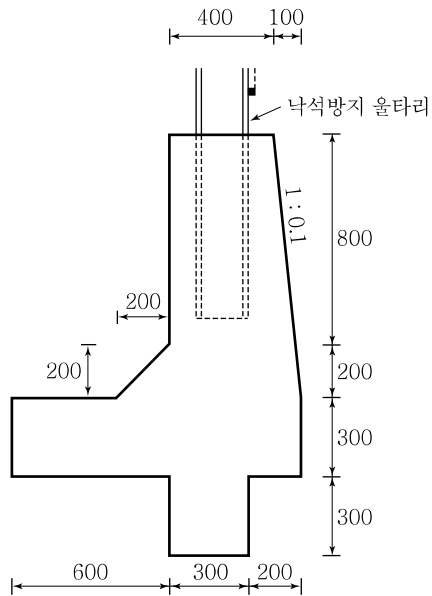
(a) 일반도
