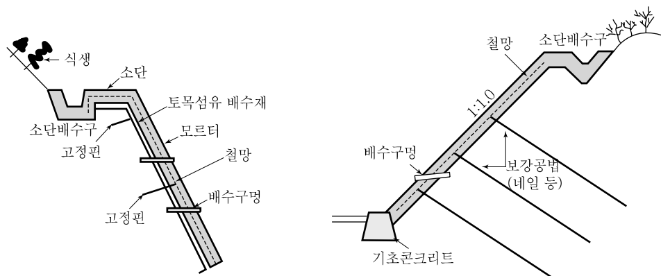
해설그림 16.1 콘크리트 뿔어붙이기 예
