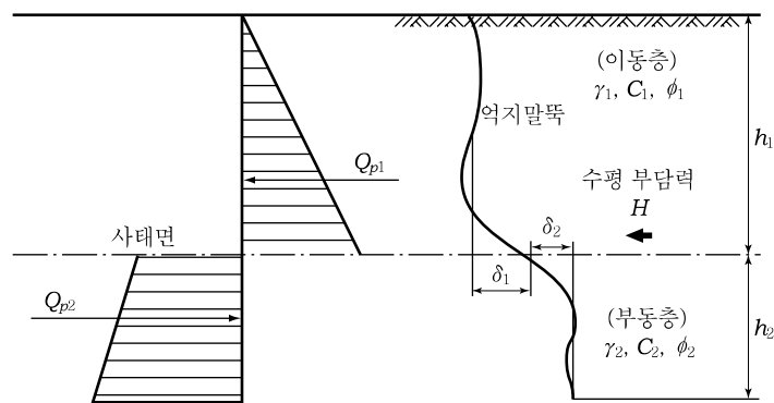
해설그림 9.10 억지말뚝에 작용하는 수동토압
