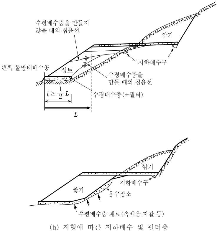
해설그림 4.5 쌓기비탈면의 주요배수시설들
