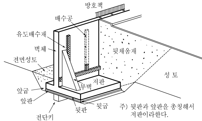
그림 1.8 옹벽의 단면에
