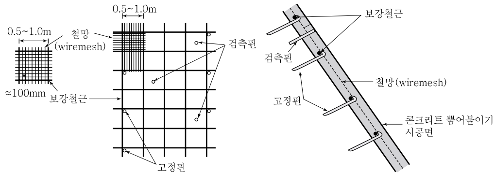
해설그림 16.2 콘크리트 뿔어붙이기 철망
