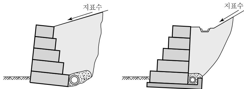
(a) 옹벽배면의 땀암거와 유공관
