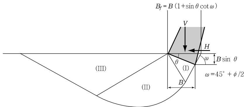
해설그림 10.18 경사진 기초의 소성영역과 환산기초폭
