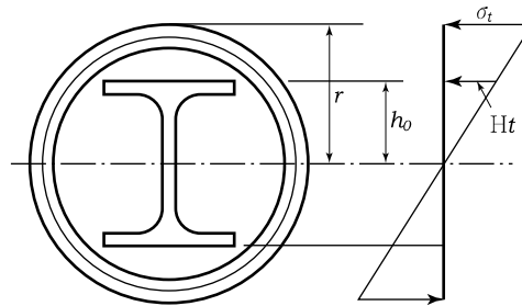
해설그림 9.3 H형강 삽입 말뚝
