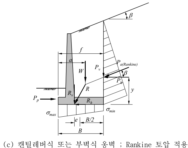
해설그림 10.4 토압의 작용 방법
