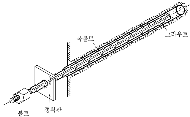
그림 1.6 록볼트의 형태
