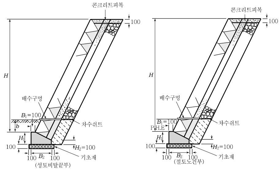
해설그림 14.4 돌(블록)쌓기 공법의 단면 및 배수시설(단위: mm)
