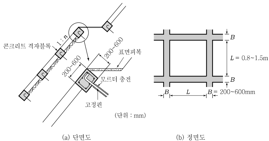
해설그림 15.1 격자블록공법
