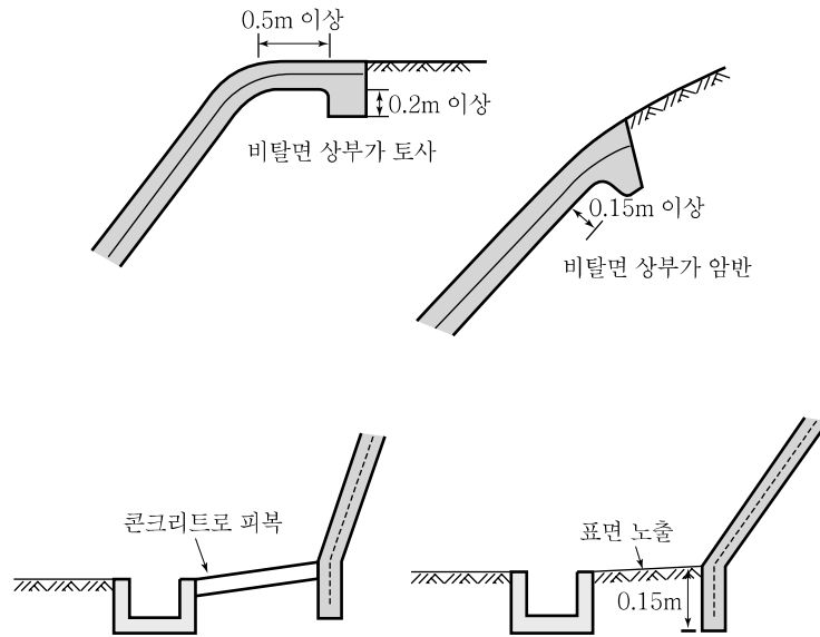
해설그림 16.3 비탈어깨와 비탈끝의 배수처리
