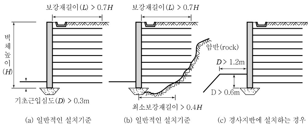
해설그림 11.3 보강토 옹벽의 설치기준
