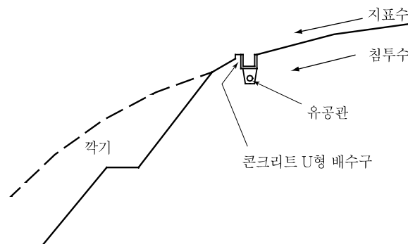
해설그림 19.3 비탈어깨의 지하배수구
