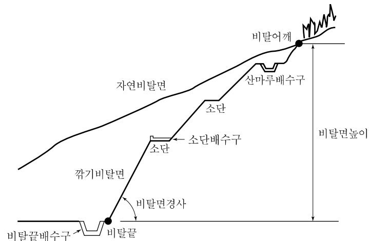
그림 1.2 깎기비탈면의 단면예
