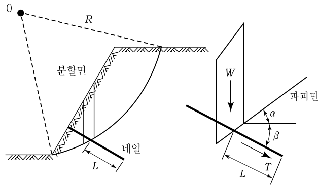
해설그림 7.6 원호활동면에 대한 안정계산
