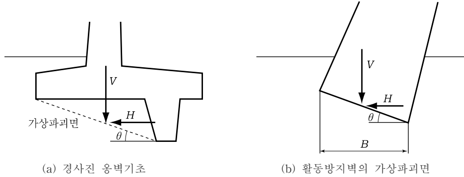
해설그림 10.17 활동저항을 위한 경사진 옹벽기초
