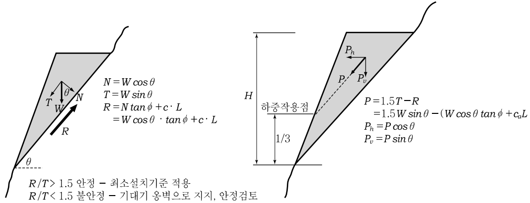
해설그림 13.5 파괴썰기에 의한 작용하중 계산
