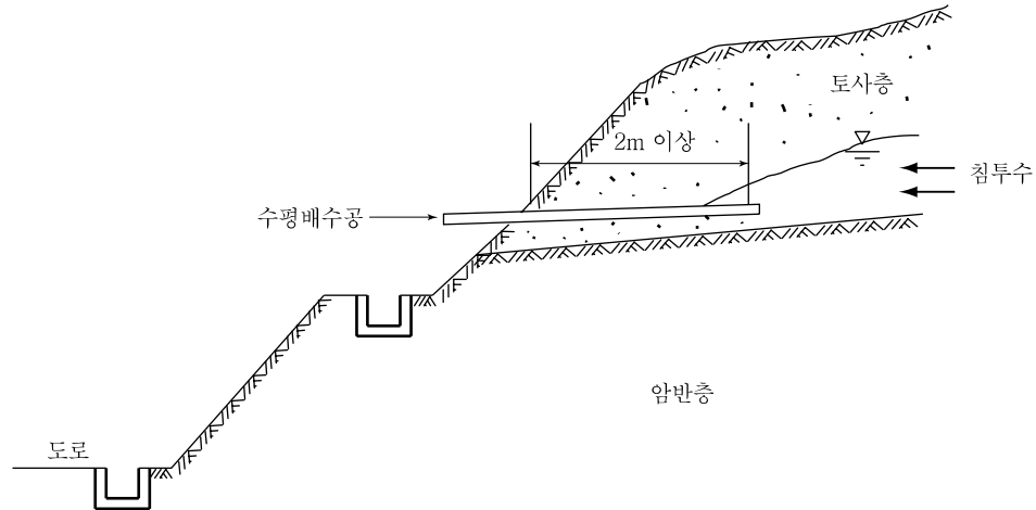
해설그림 19.7 수평 배수공
