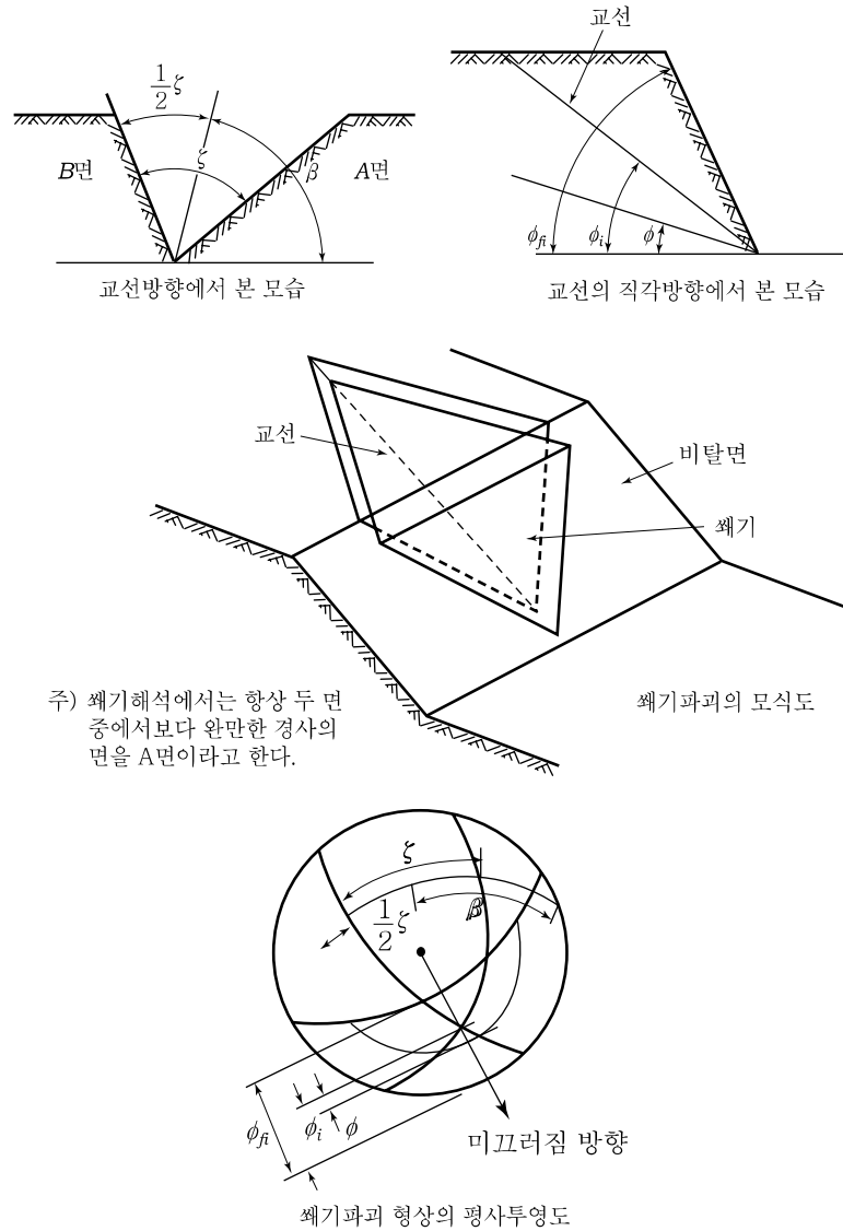
해설그림 5.4 썩기파괴의 기하학적 형상
