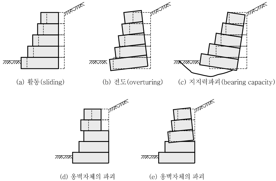
해설그림 12.4 돌망태 옹벽의 파괴형태
