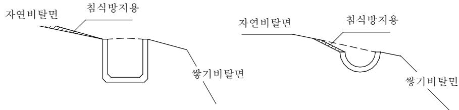
해설그림 18.4 프리캐스트제품에 의한 비탈어깨배수구
