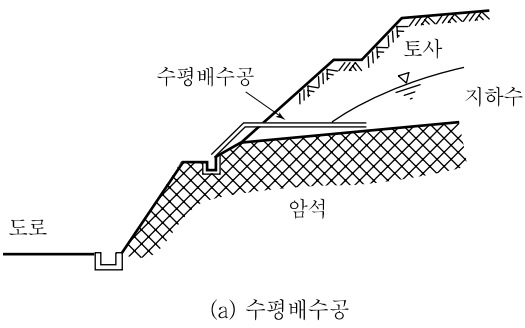
해설그림 5.6 깎기비탈면에서의 배수공법
