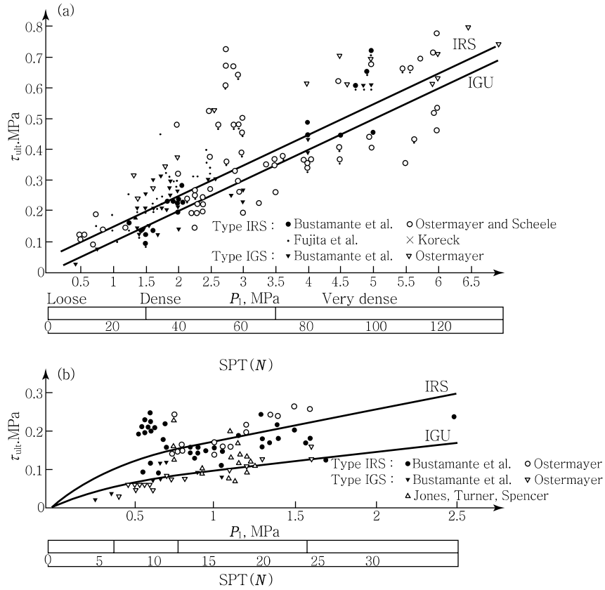
해설그림 7.2 한계압에 따른 네일의 단위주면마찰저항력
