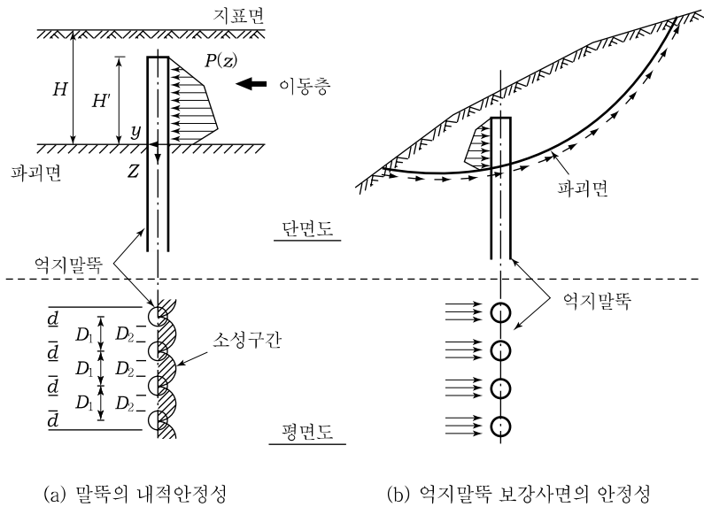
해설그림 9.6 억지말뚝의 비탈면 안정해석 개념도
