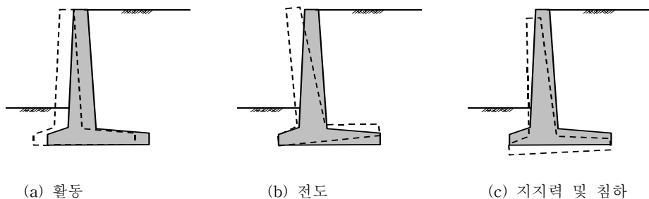
해설그림 10.13 옹벽의 안정성 검토
