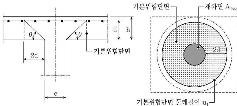
그림 5.7.9 뚫림전단 검증모델
