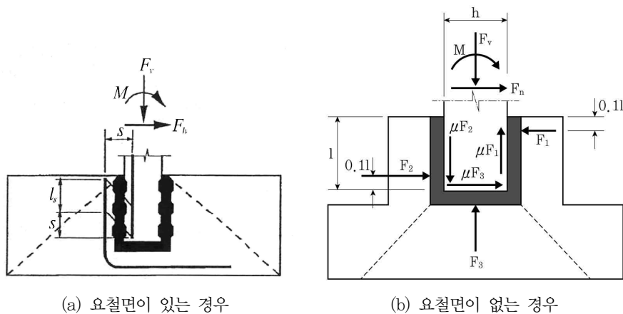
그림 5.13.7 포켓기초
