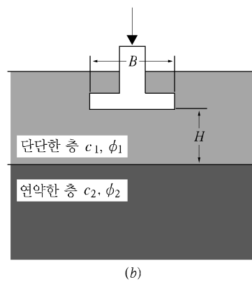
그림 7.6.7 2층으로 구성된 지반
