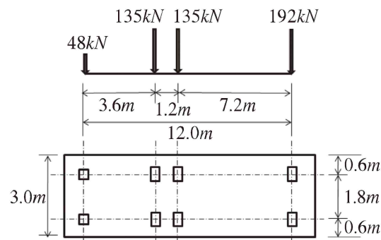
그림 3.6.1 표준트럭하중
