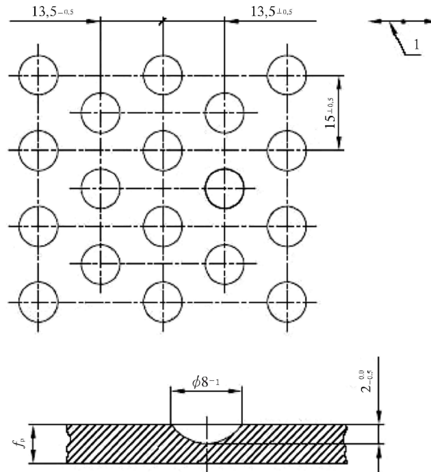
그림 9.5.10 댐플의 형상과 패턴
