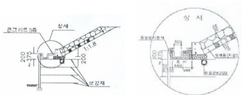
<그림3. 판넬식 보강토 옹벽과 성토시설물 중복구간 처리방안>
