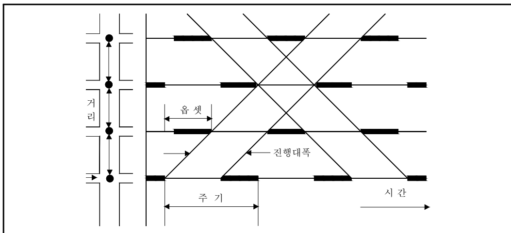
<그림 4.3> 이상적인 조건의 시공도
