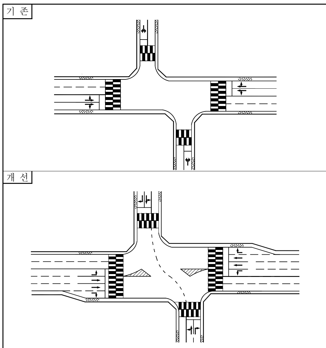
<그림 6.3> 엇갈림 교차로의 개선
