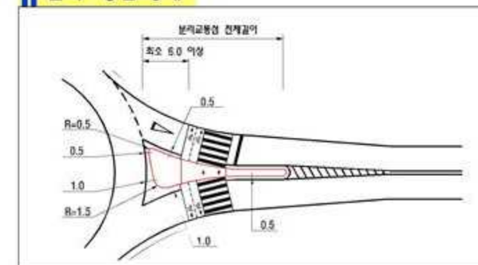
■ 분리교통섬 상세
