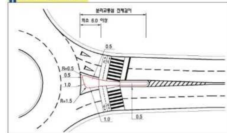
■ 분리교통섬 상세
