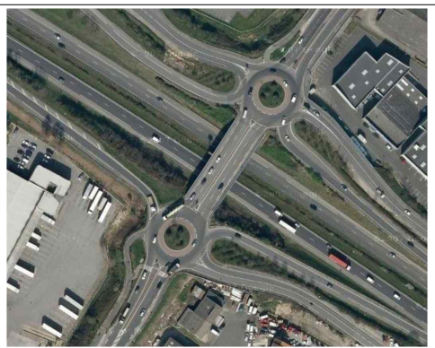
쌍구형 입체 회전교차로(프랑스)
