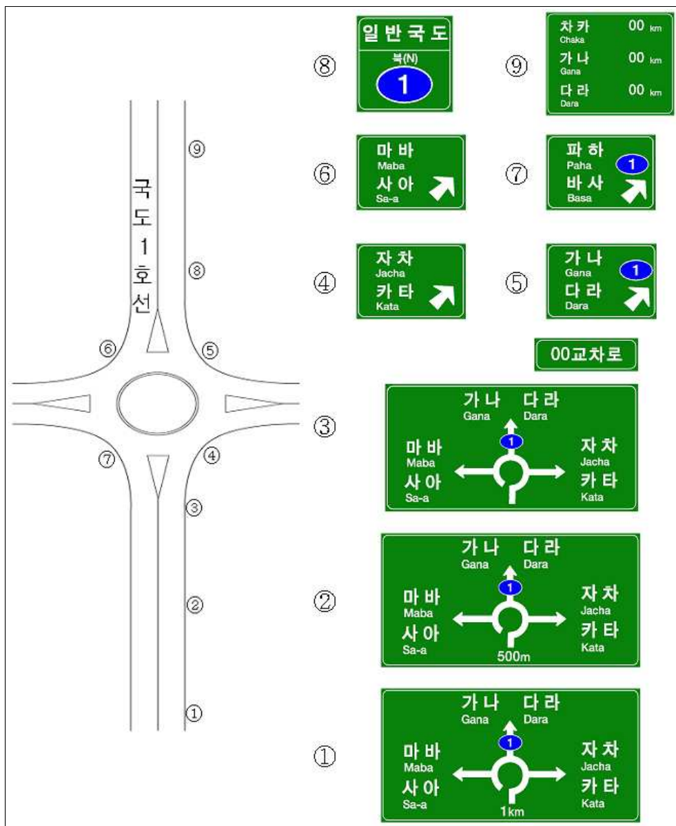
<그림 4.33> 도로안내표지 설치 예
