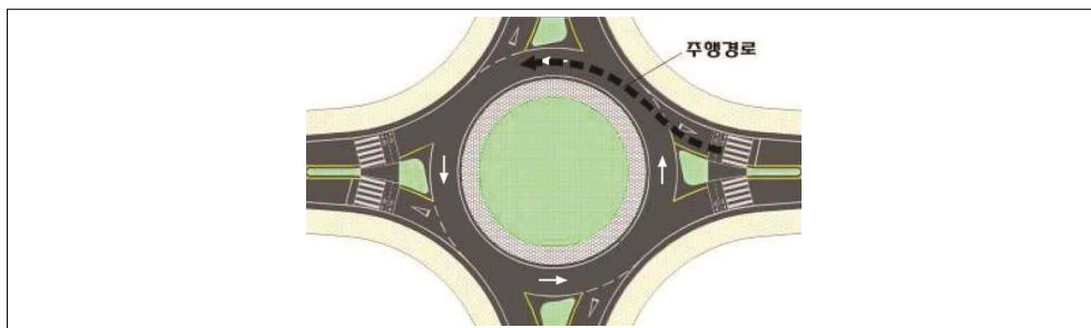
<그림 4.2> 진입로 기하구조를 통한 자동차 주행경로 곡선화
