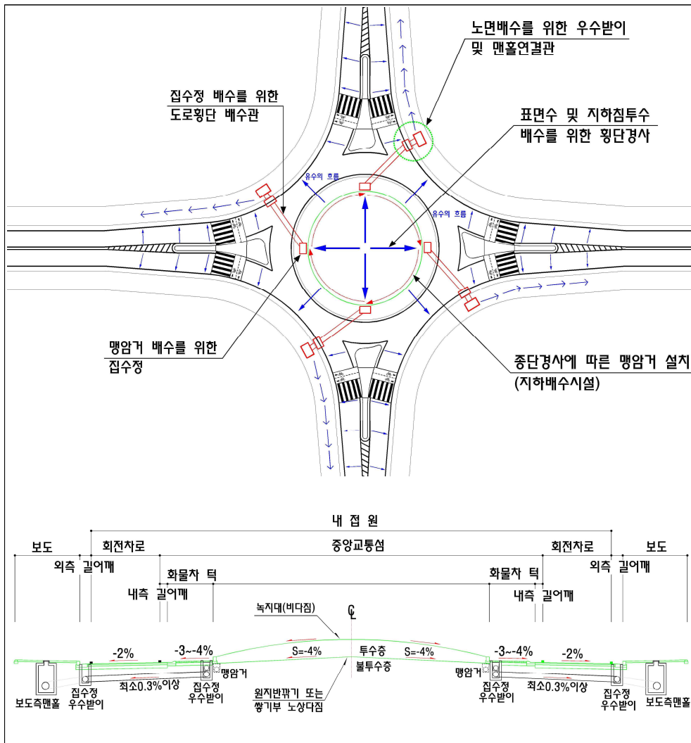
<그림 4.42> 배수시설 설치 예
