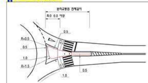
|| 분리교통섬 상세
