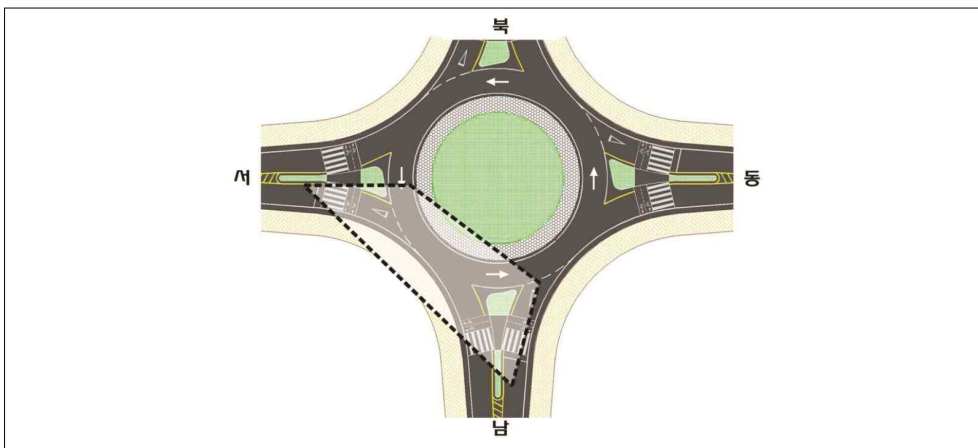
<그림 4.6> 진입부 자동차 시거 확보 필요 구간
