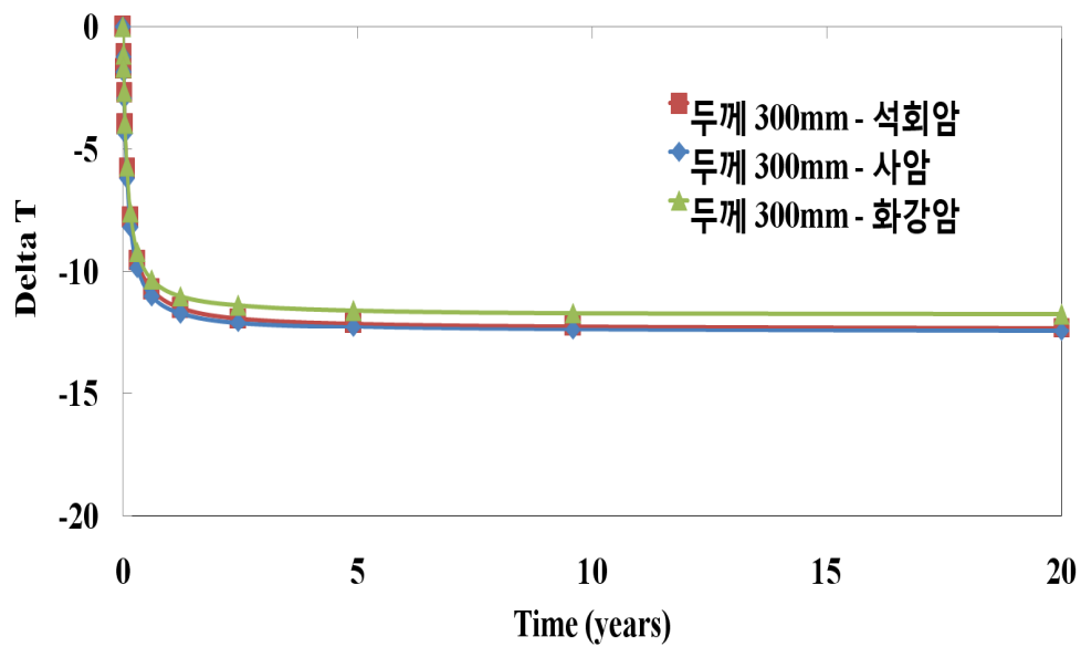
(c) 암종별 응력감소가 고려된 부등건조수축 예측량3(V/S= 300mm)
