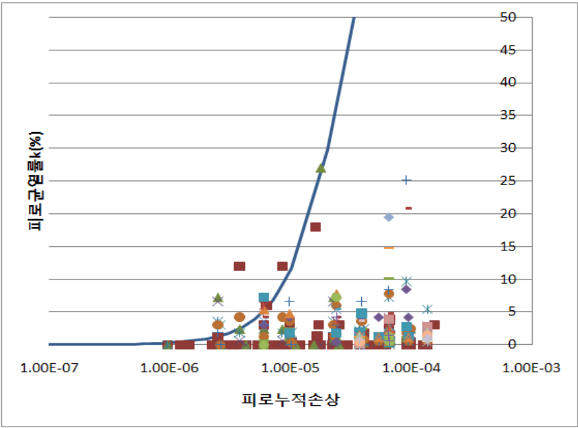
<그림 11.48> 피로누적손상 vs 피로균열율
