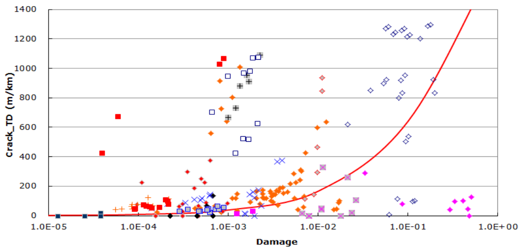
<그림 11.47> 하향균열에 대한 전이함수
