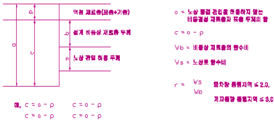
<그림 4.13> 노상동결 관입허용법에 의한 설계 비동결성 재료층 두께결정 도표
