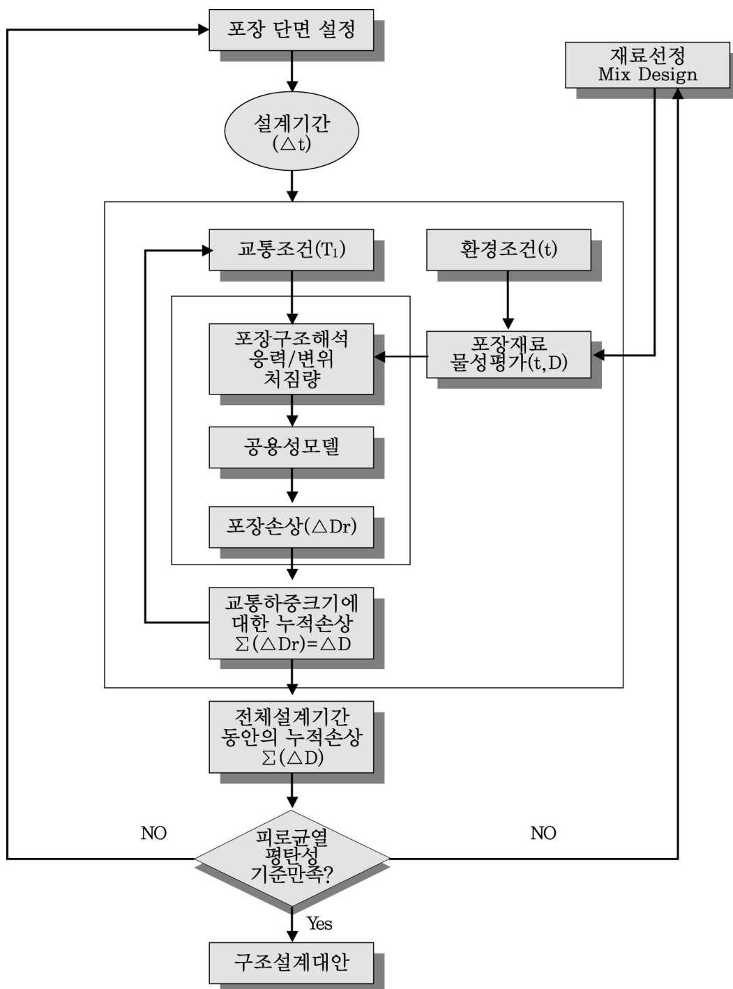
<그림 1.1> 시멘트 콘크리트 포장의 역학적-경험적 설계 절차
