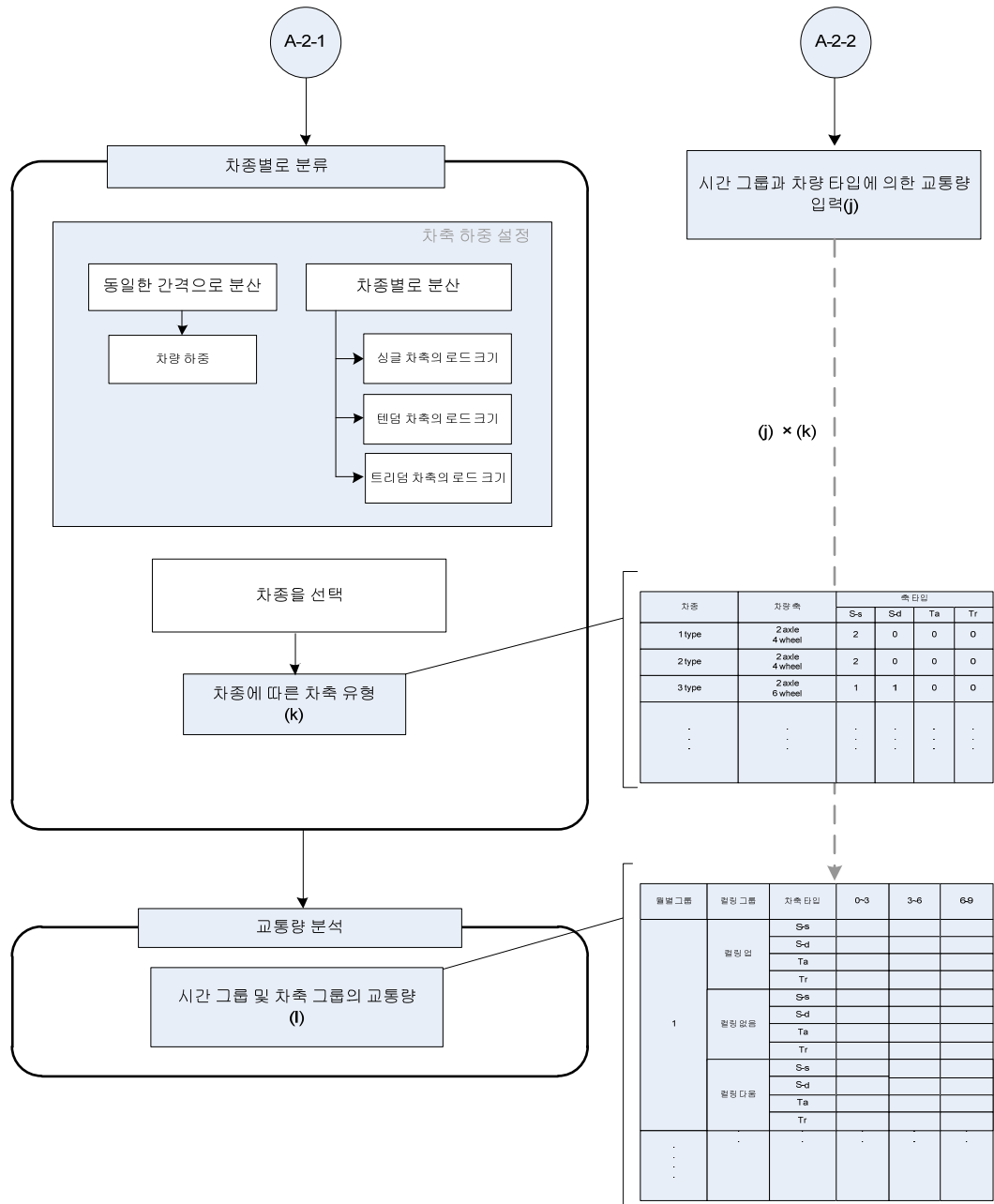
<그림 1.14> 도로포장 구조 설계 교통하중 로직 (2)
