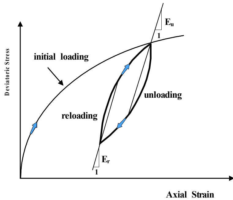
<그림 3.1> 삼축압축시험에서 결정되는 전형적인 응력-변형률 곡선
