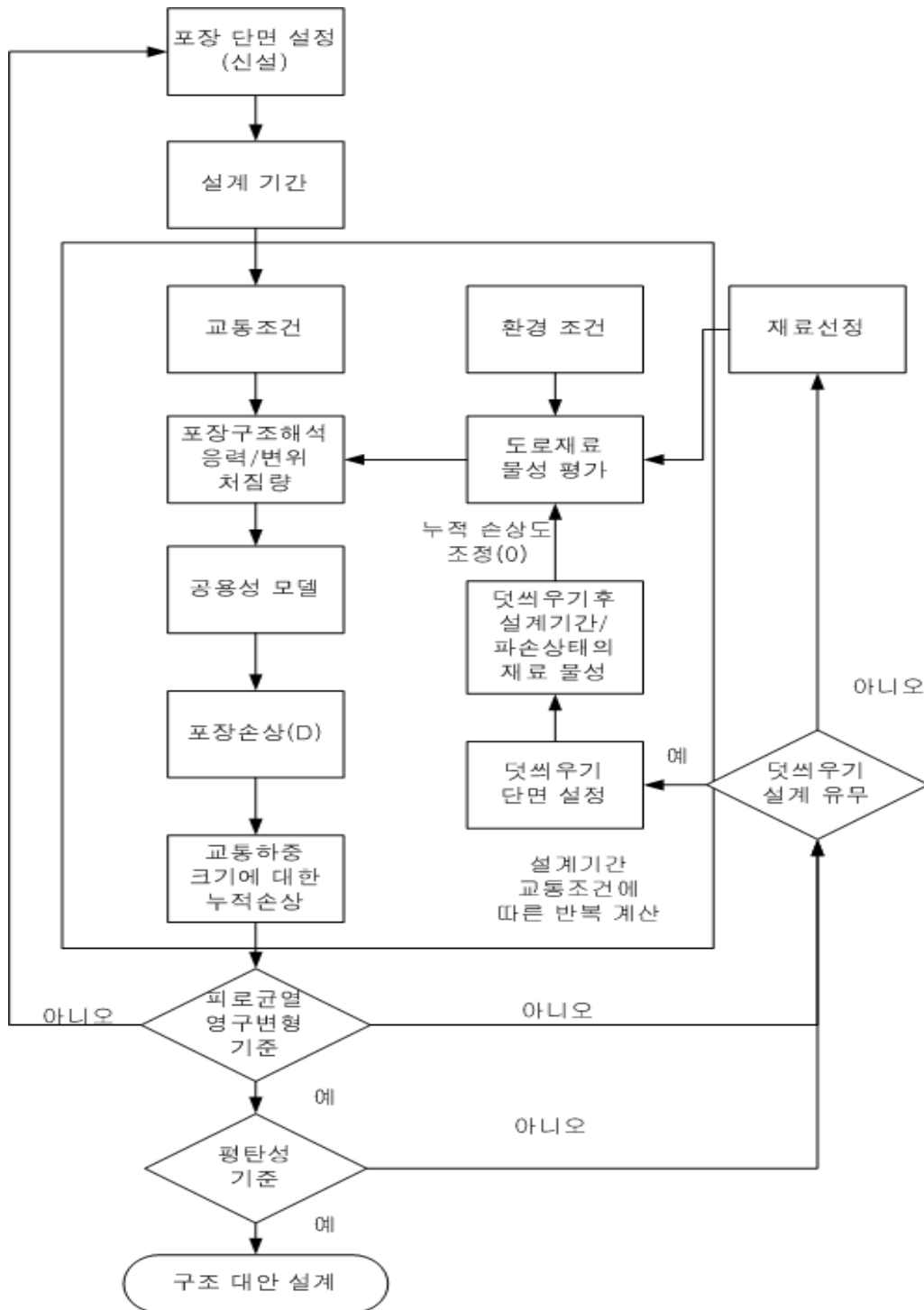
<그림 12.9> 덧씌우기 설계 포함된 신설 포장 설계 흐름도
