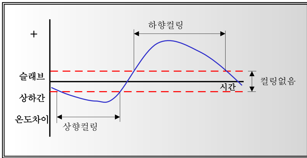
<그림 10.10> 24시간 동안의 컬링 사이클
