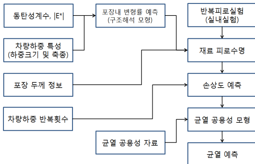
&lt;그림 11.13&gt; 균열 예측 순서도
