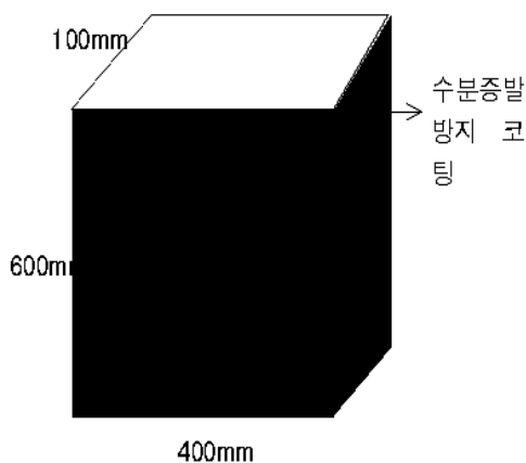
<그림 9.8> 도로포장용 시편
