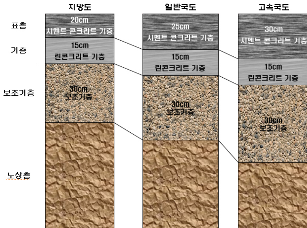
<그림 2.2> 시멘트 콘크리트 포장의 기본 설계 단면
