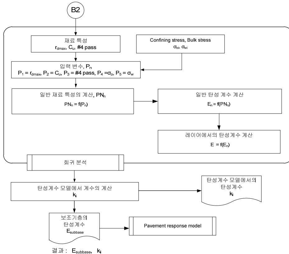
&lt;그림 4.4&gt; 보조기층 탄성계수 결정 로직
