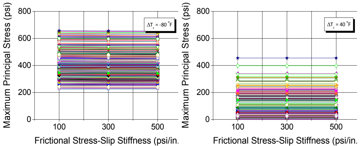
&lt;그림 16.10&gt; 슬래브와 하부층의 마찰력의 영향
