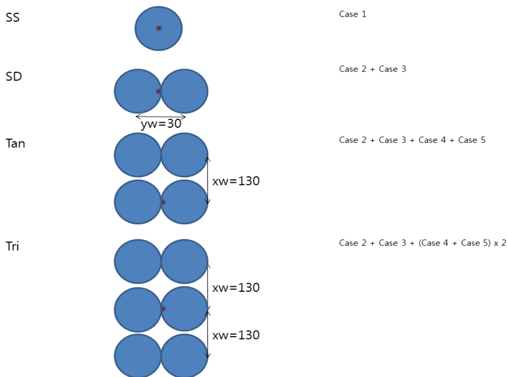
<그림 10.2> KICTMLE에서 고려하는 하중조건과 중첩방법
