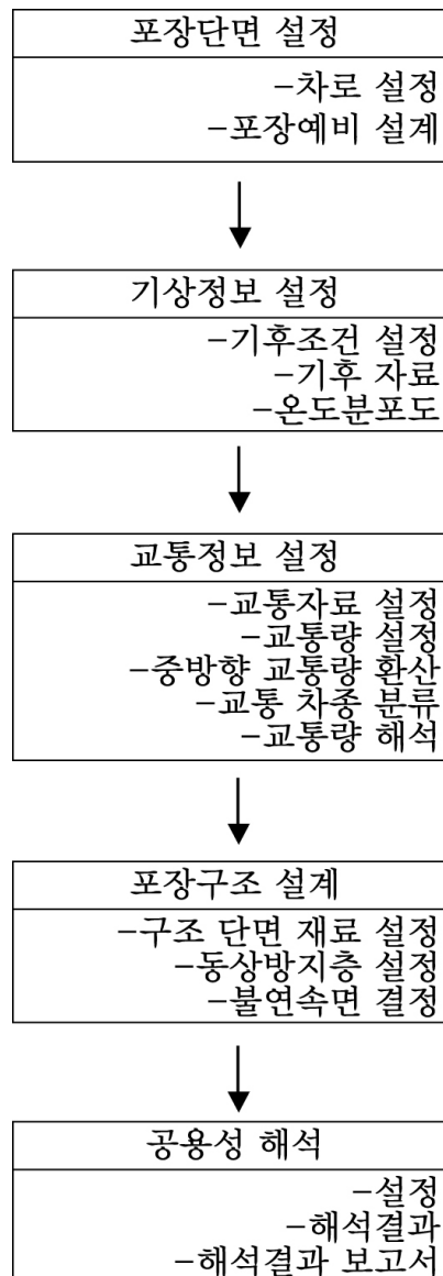
<그림 15.1> 설계흐름도
