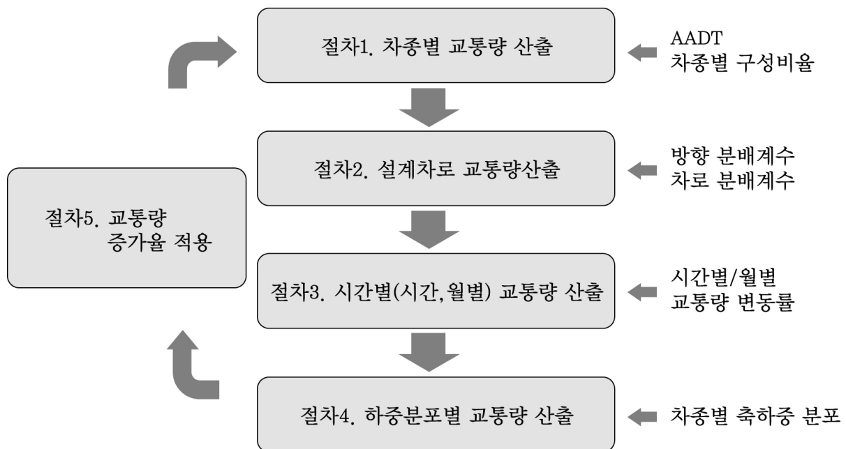
<그림 3.1> 포장설계 시 교통량 산출 절차
