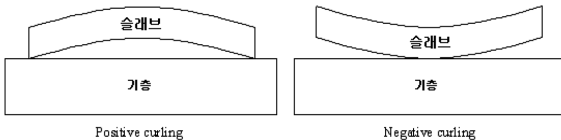
<그림 2.1> 컬링(Curling)에 의한 슬래브의 거동
