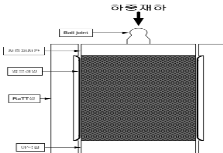
<그림 11.18> RaTT(Rapid Triaxial Testing system) 셀
