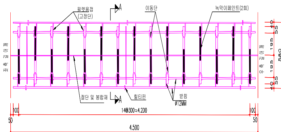
(a) 다웰바 설치 도면
