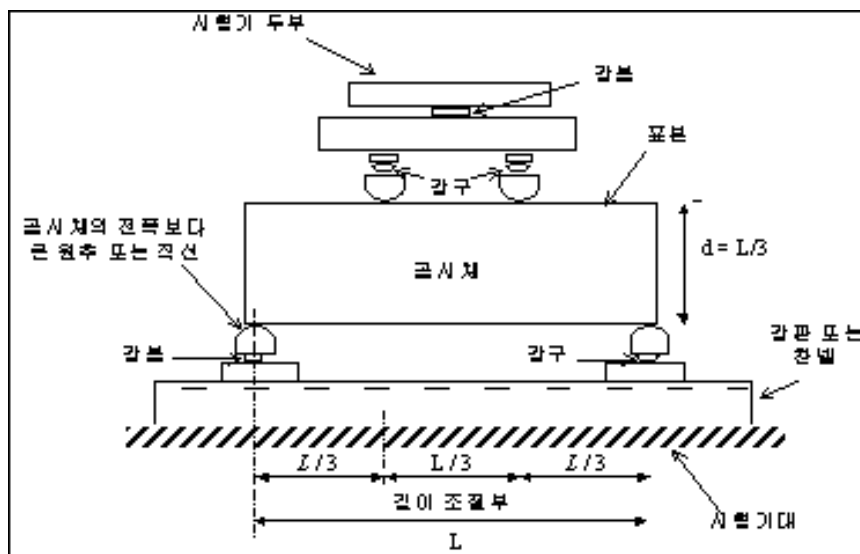
<그림 7.7> 휨강도 시험방법 (단순보의 3등분점 하중법)
