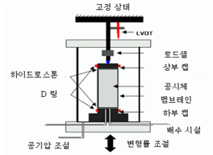
<그림 4.1> 회복탄성계수 측정 장비
