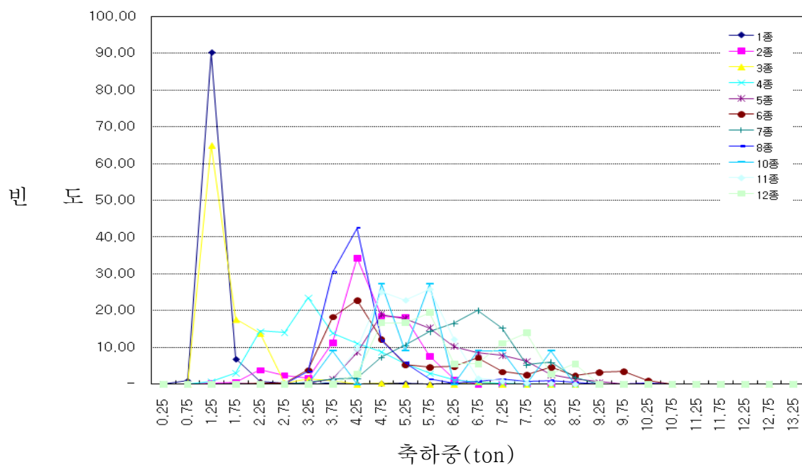
<그림 3.2> 차종별 단축(Single Axle) 축하중 분포의 예
