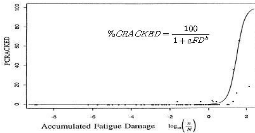
<그림 11.45> 일반적 균열발생률과 누적 피로손상과의 관계
