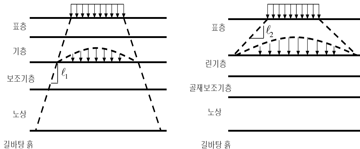
<그림 2.2> 국내 포장 대표 단면 및 응력 분포도
