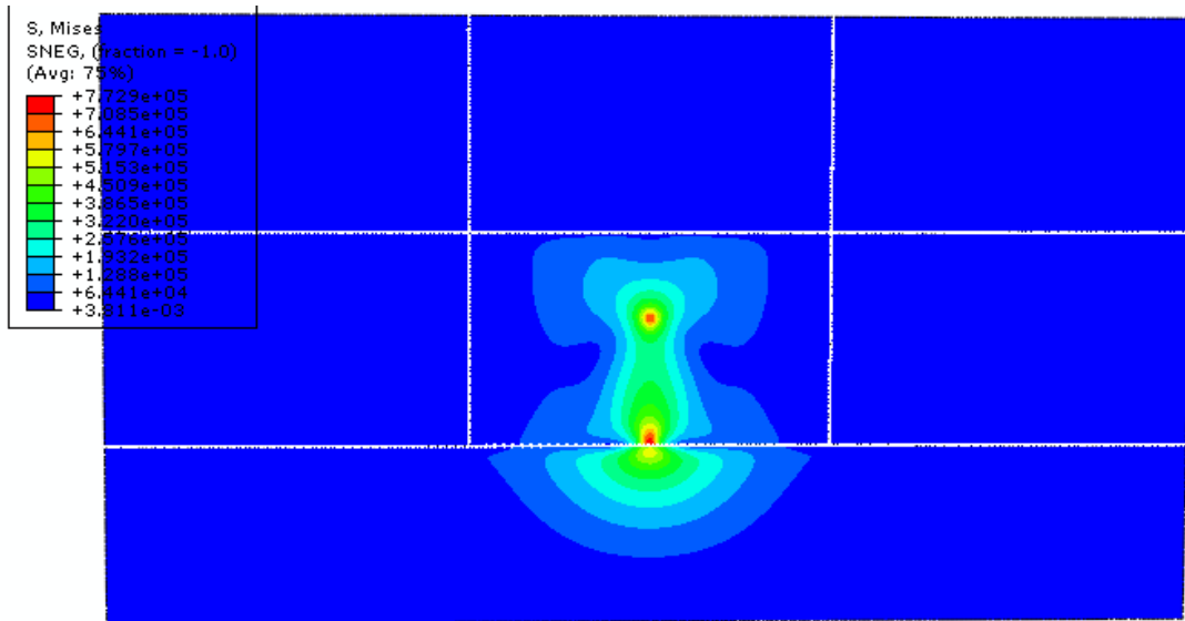
<그림 10.15> 길어깨의 하중 전달율이 50% 일 경우의 응력 분포도
