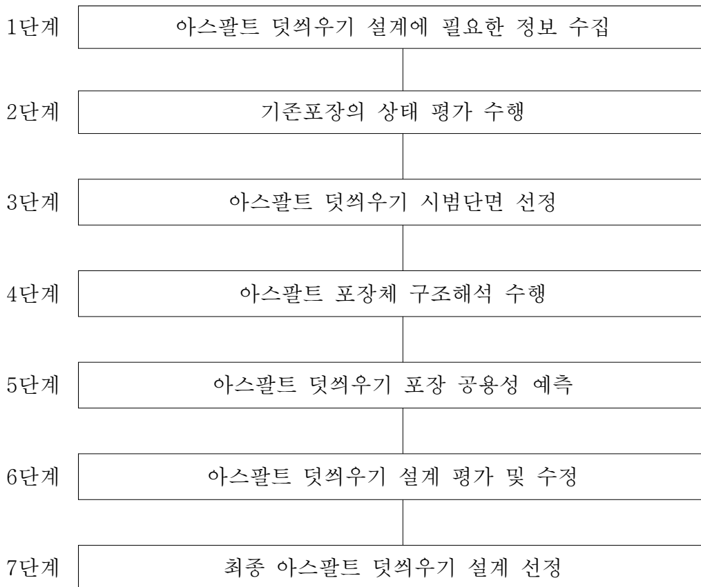
<그림 8.1> 아스팔트 포장 상부 아스팔트 덧씌우기 포장설계 절차
