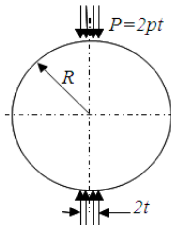
&lt;그림 7.8&gt; 쪼갬인장강도 실험
