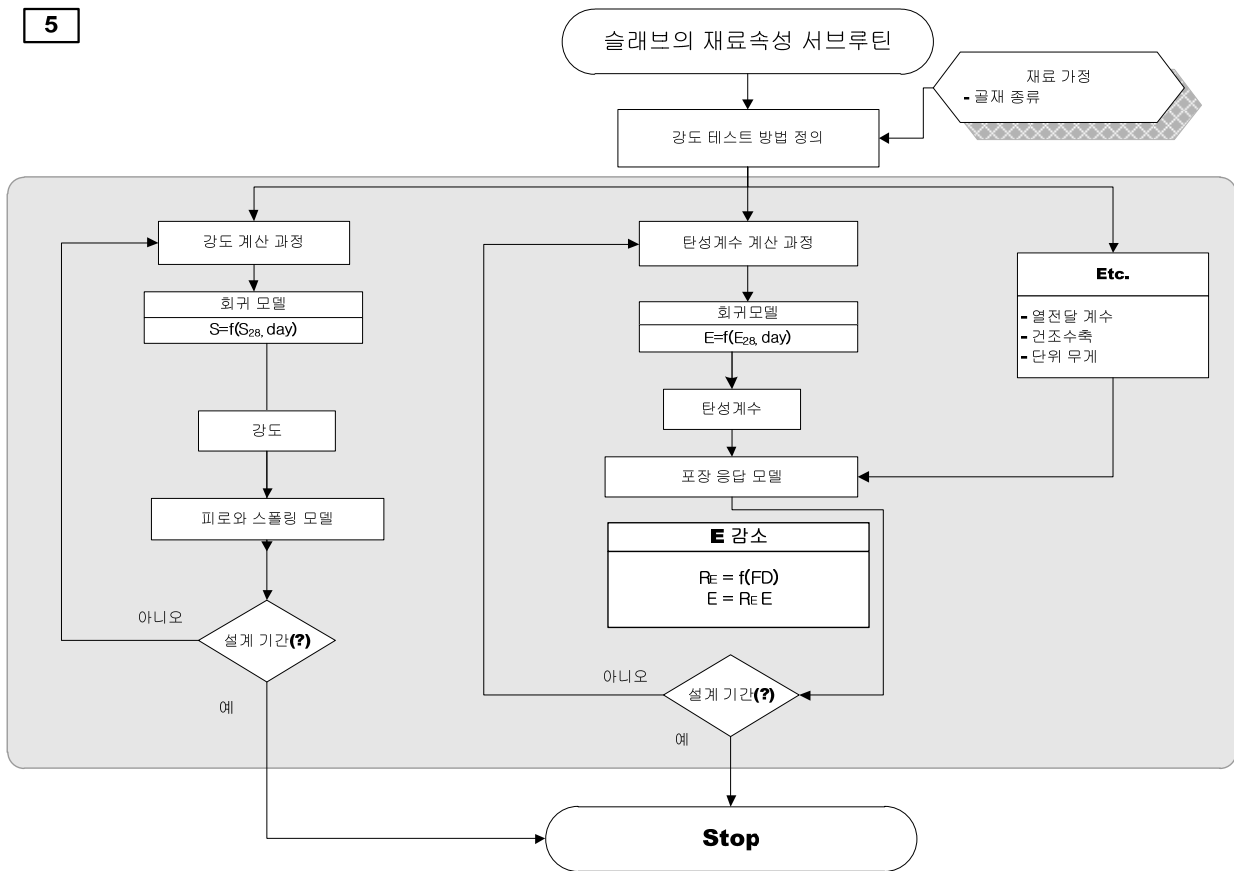
<그림 7.1> 콘크리트 재료물성 산정로직
