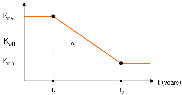
&lt;그림 4.10&gt; 복합지지력 저하 함수
