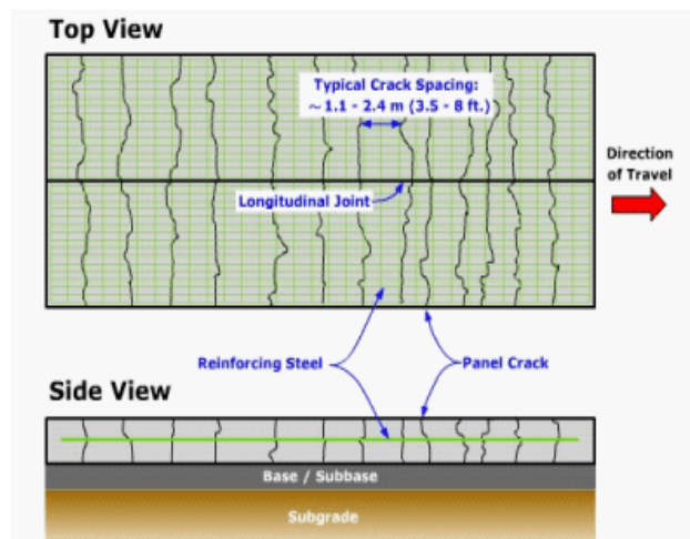
(c) 연속 철근 콘크리트 포장
