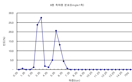
(e) 8종 Single1 축 하중분포(11종 구분)
