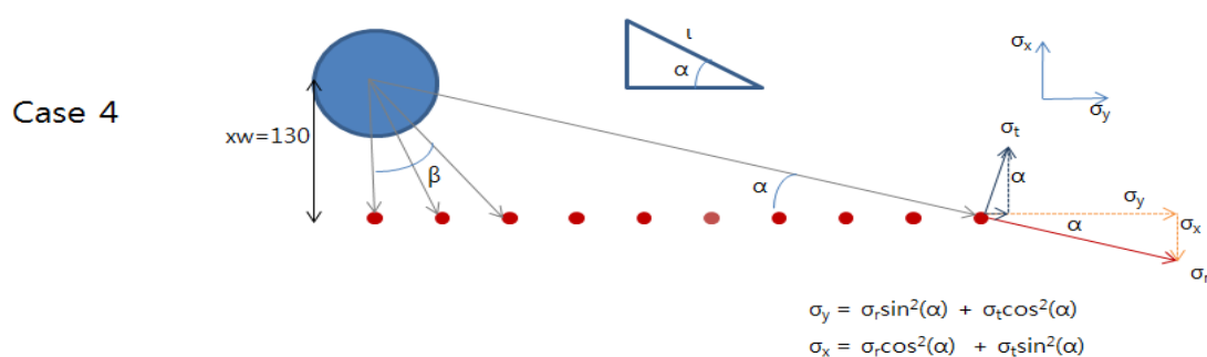
<그림 10.4> Case 4에서의 x, y 방향 응력 결정방법
