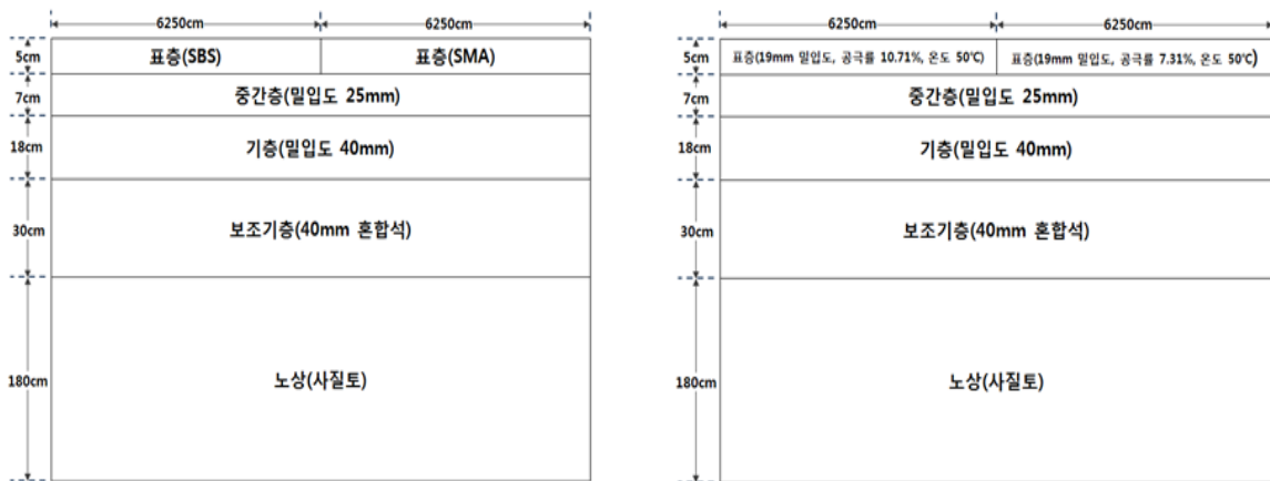
<그림 11.34> 가속실험에 사용된 개질(좌) 및 밀입도 혼합물의 포장 단면
