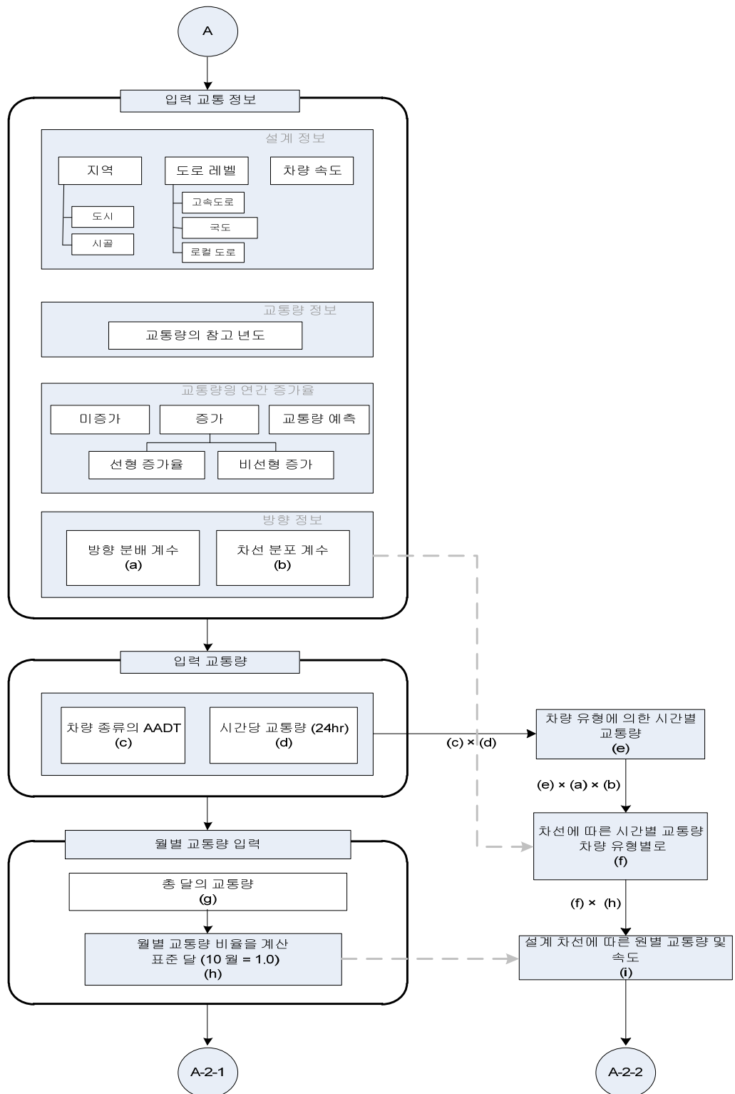
<그림 1.13> 도로포장 구조 설계 교통하중 로직 (1)
