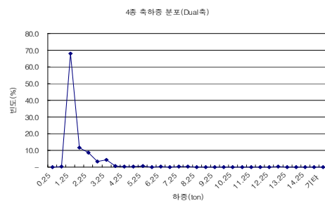
(b) 4종 Dual 축 하중분포(11종 구분)
