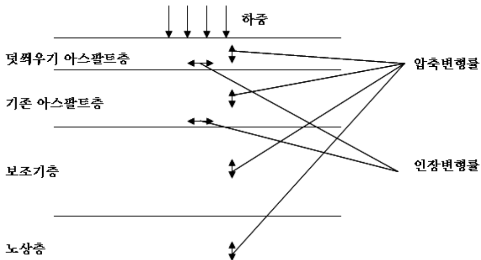
&lt;그림 12.6&gt; 아스팔트 덧씌우기 포장 구조해석
