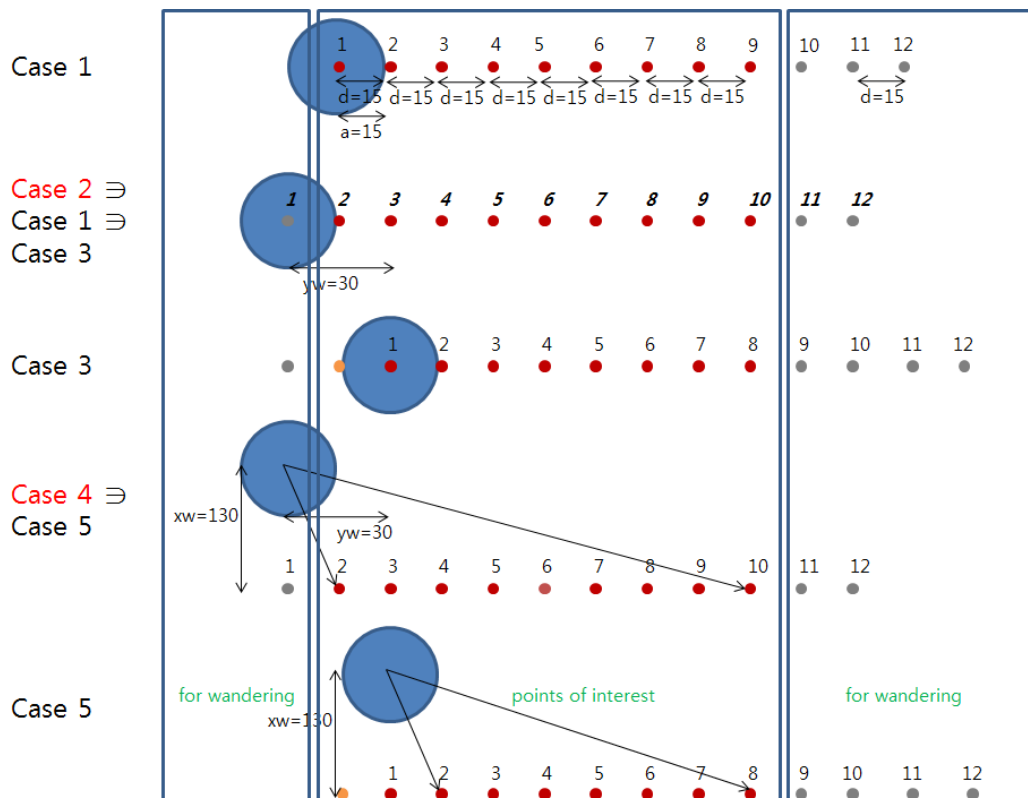
<그림 10.3> 단축단륜(SS) 조건에서의 하중조건과 측점의 위치
