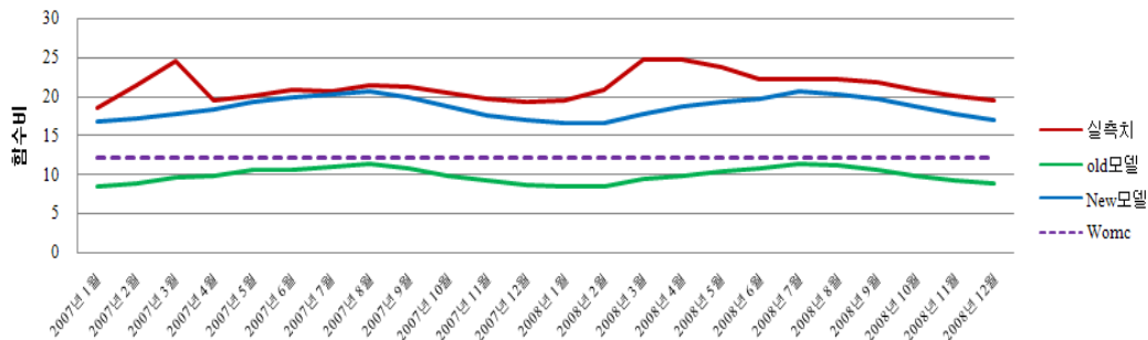
&lt;그림 2.10&gt; 실측값과 모형값 함수비 비교
