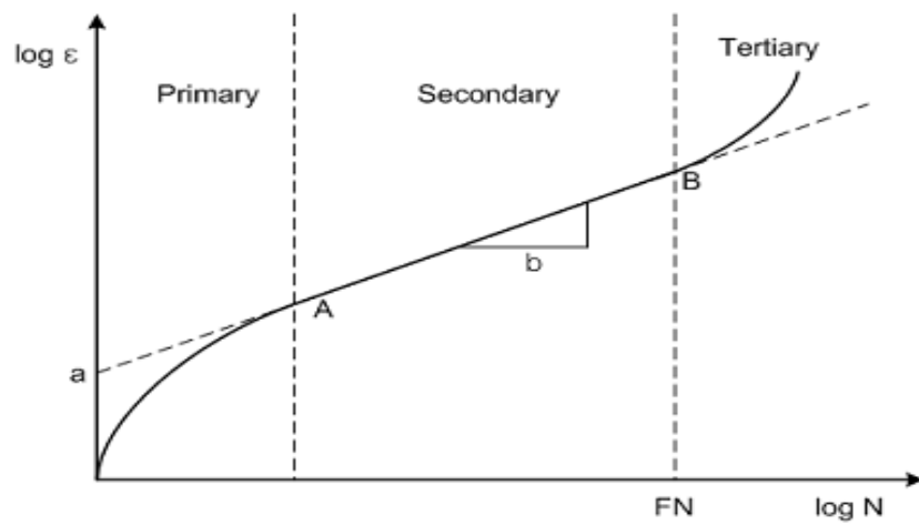
<그림 11.16> 영구 변형률과 하중재하 회수의 전형적 관계
