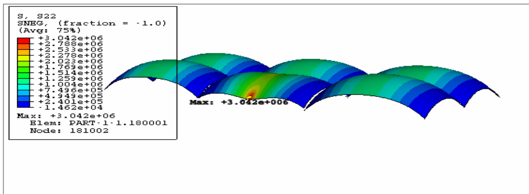
&lt;그림 10.12&gt; 상향균열을 유발하는 온도 및 차륜하중에 기인한 응력선도
