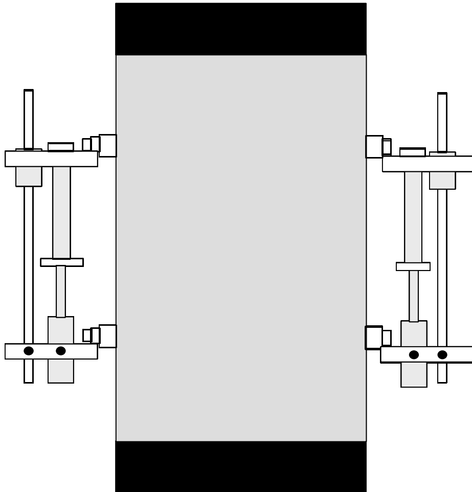
<그림 6.2> LVDT 설치 방법
