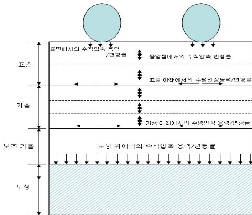
<그림 10.7> 아스팔트 포장의 구조해석결과
