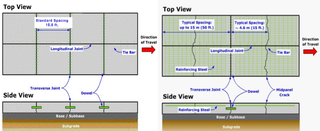
(a) 무근 줄눈 콘크리트 포장
