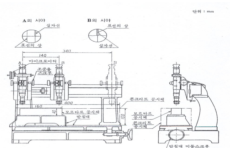
<그림 9.2> 콤퍼레이터 방법의 측정기
