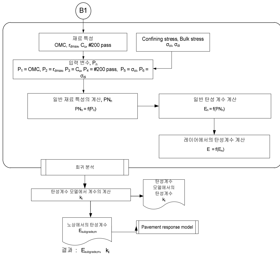
<그림 4.3> 노상 탄성계수 결정 로직
