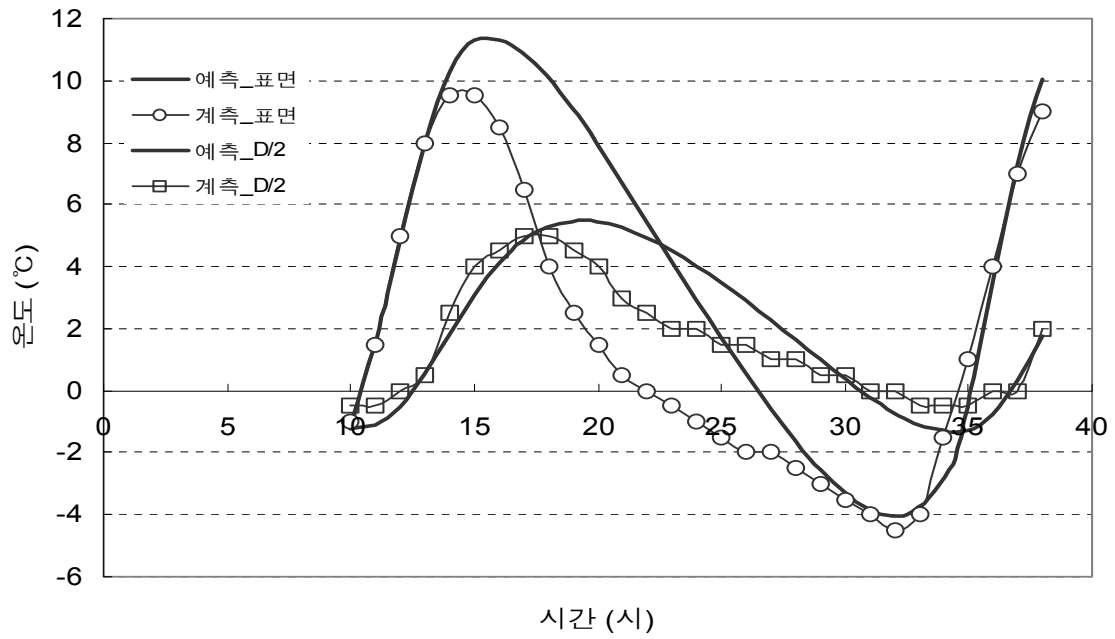
<그림 2.8> 충주지역의 온도예측 결과(겨울)
