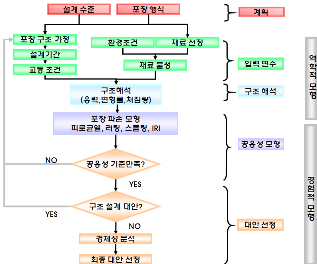
<그림 1.2> 역학적-경험적 설계 기본모형
