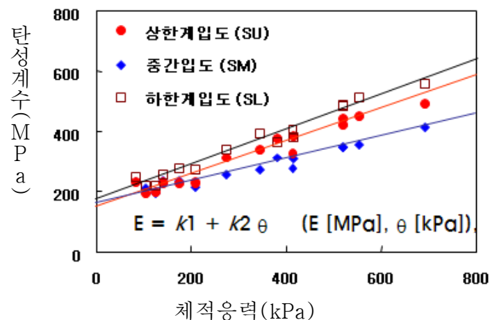
<그림 3.4> 쇄석기층의 일반적인 탄성계수
