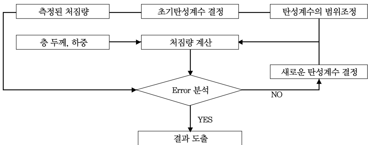
<그림 8.5> 포장층 탄성계수 역산 절차
