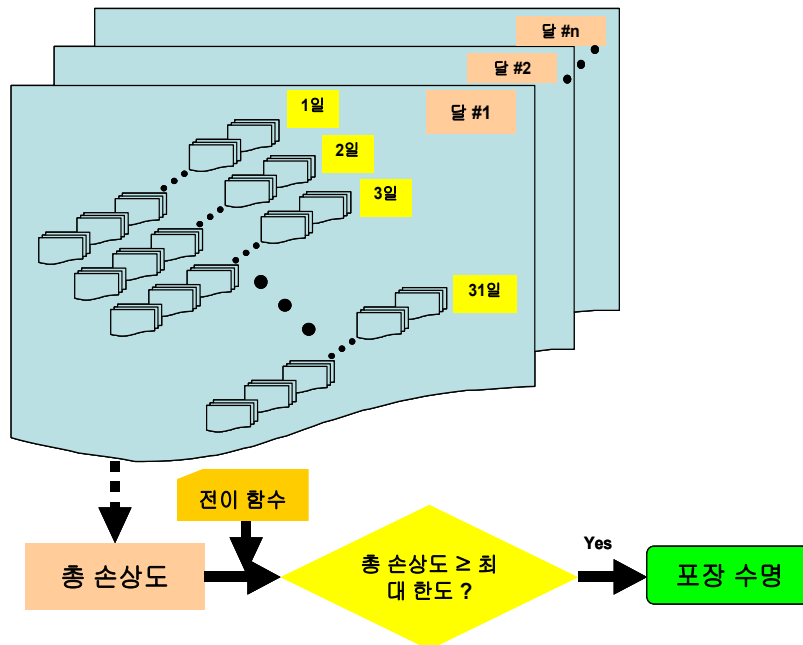
&lt;그림 11.9&gt; 전체 누적 손상 계산
