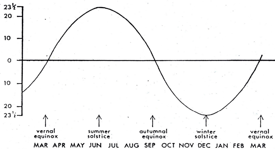
<그림 2.5> 계절에 따른 declination angle
