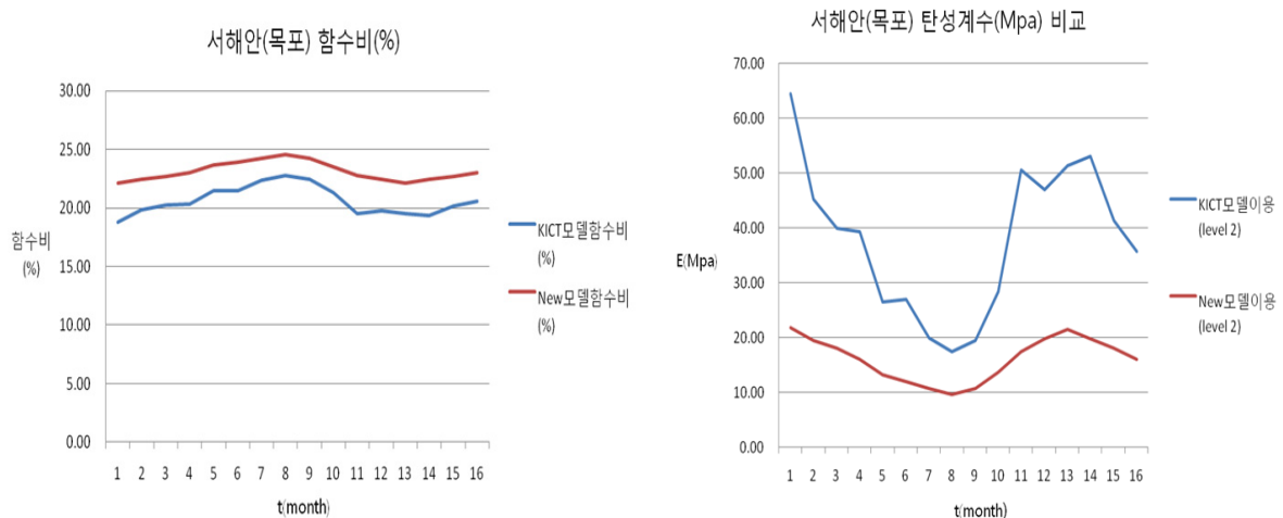
&lt;그림 2.12&gt; 함수비 변화에 따른 탄성계수 변화 비교(서해안)
