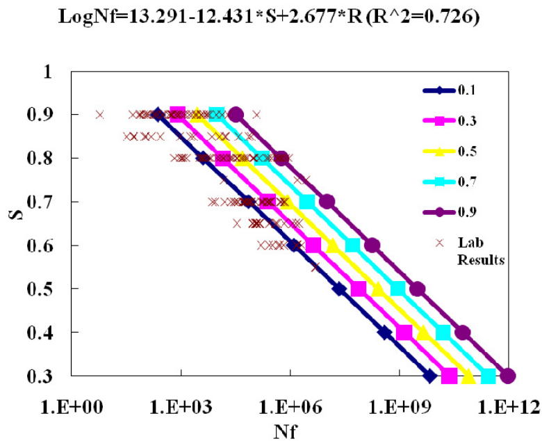
<그림 11.26> 개발 모형의 R에 대한 민감도
