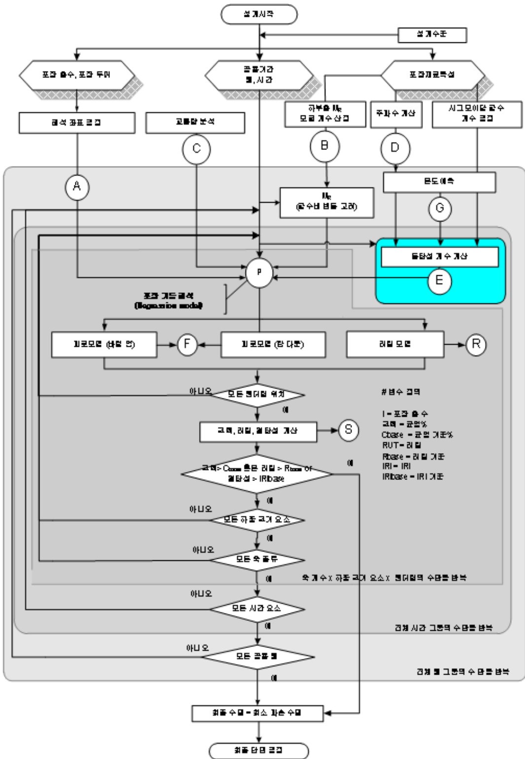
<그림 1.3> 아스팔트 포장 설계 로직
