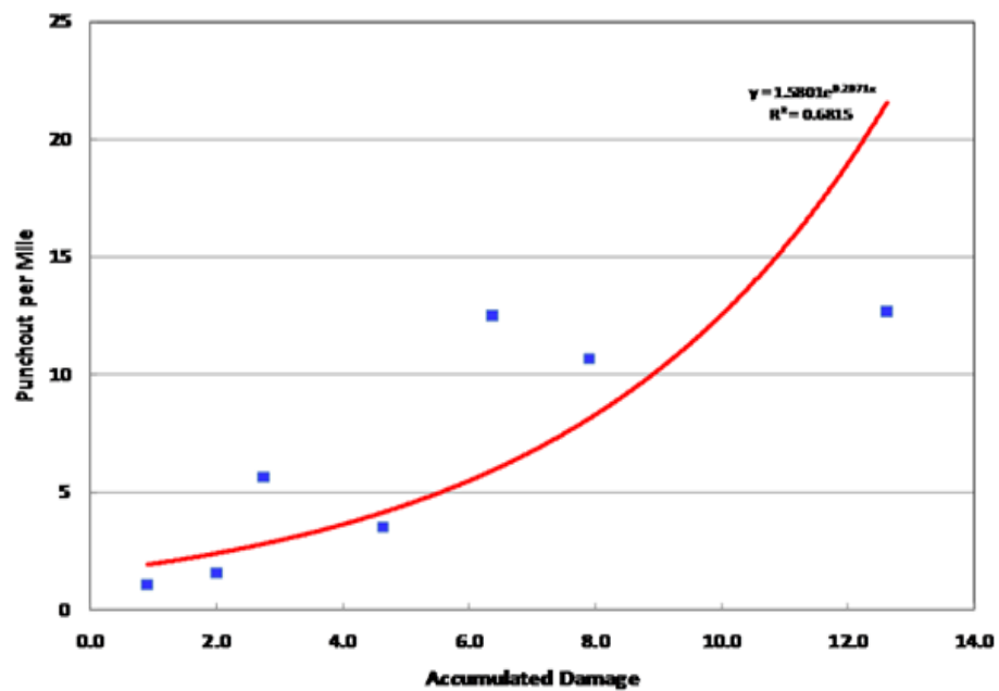
<그림 8.3> 전이함수를 이용한 파손율과 편치아웃과의 상관관계
