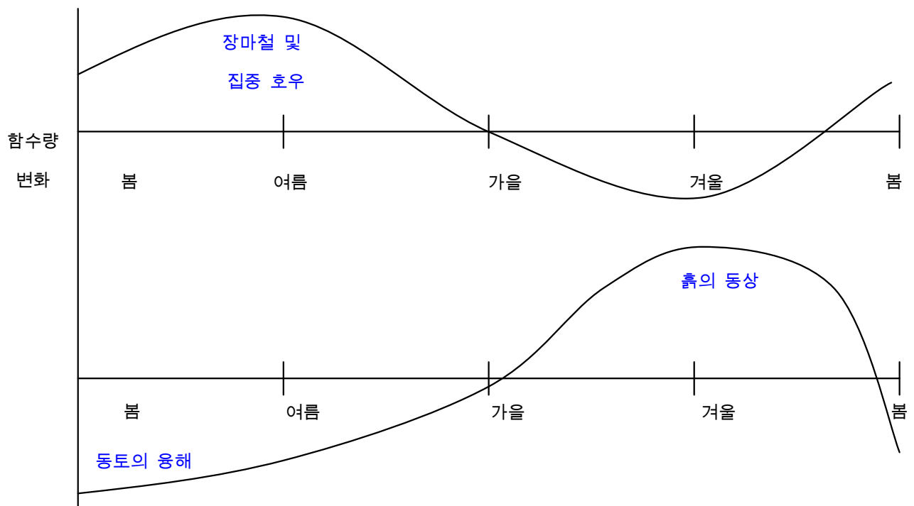
<그림 2.2> 계절 변화에 따른 노상의 함수비 및 탄성계수 변화
