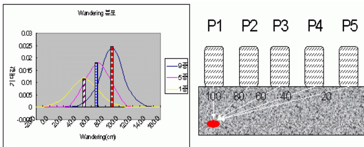
<그림 1.10> 차종에 따른 Wandering 분포 및 중첩효과
