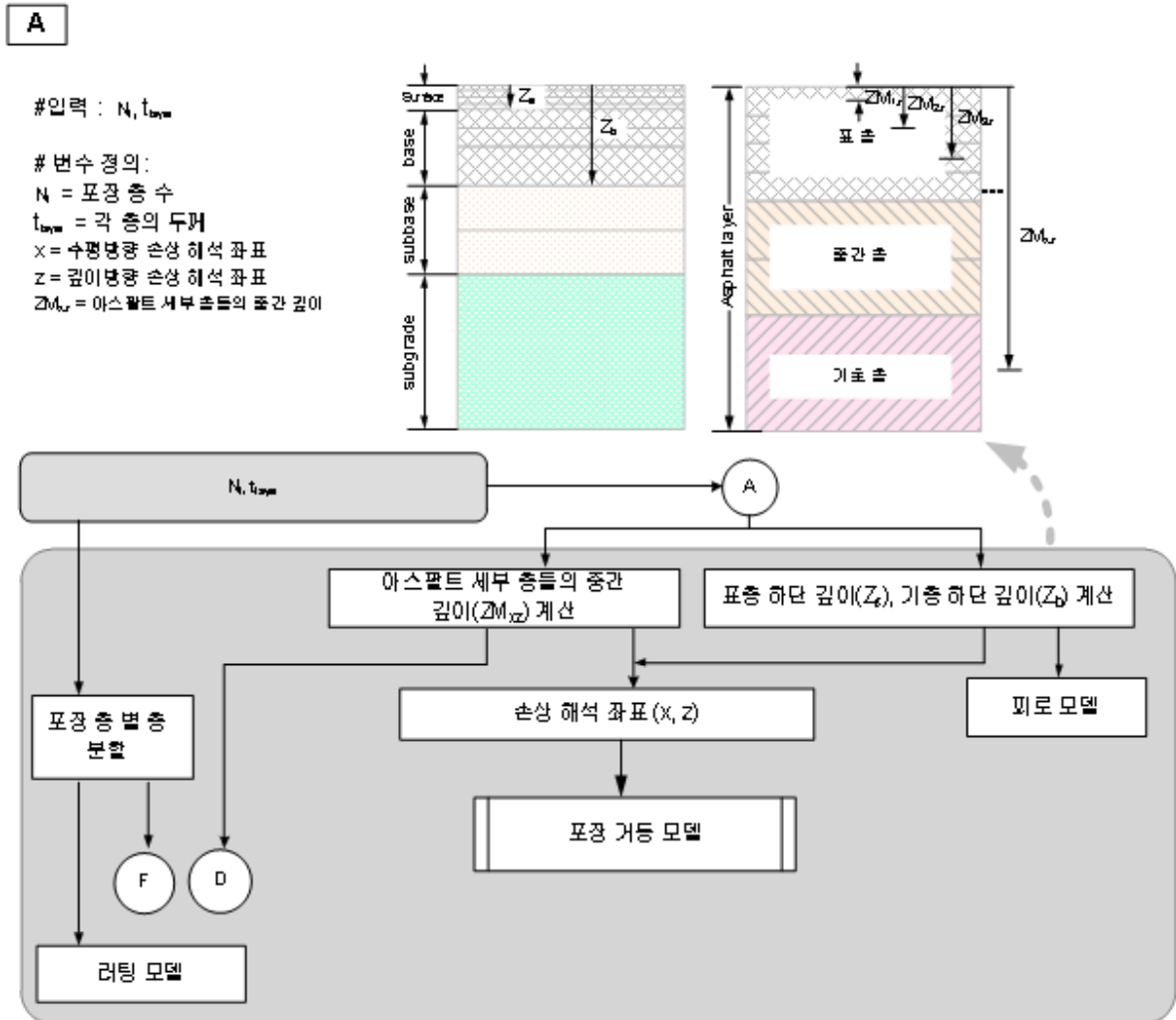
<그림 1.4> 각 층의 분할
