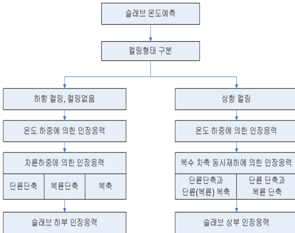
&lt;그림 10.8&gt; 콘크리트포장 구조해석 개념도
