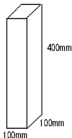
<그림 9.7> 표준시편
