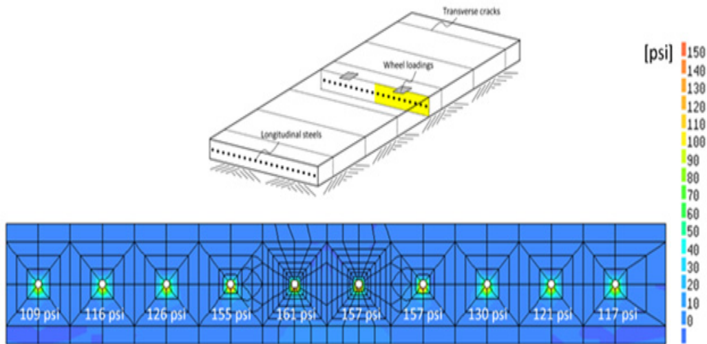
<그림 8.1> 연속철근 콘크리트 포장의 구조해석
