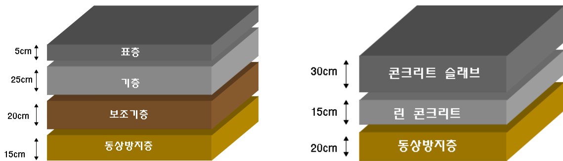
(a) 아스팔트 포장 단면
