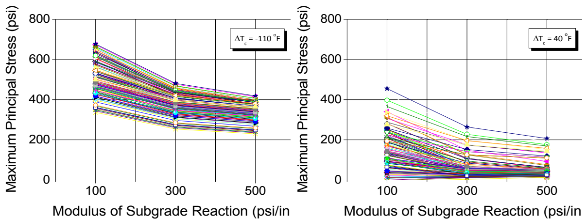
&lt;그림 16.6&gt; 하부 복합지지력의 영향
