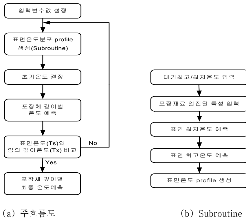
<그림 2.4> 온도예측모형 개발 흐름도
