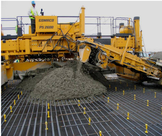
(a) 연속철근 콘크리트 포장 시공
