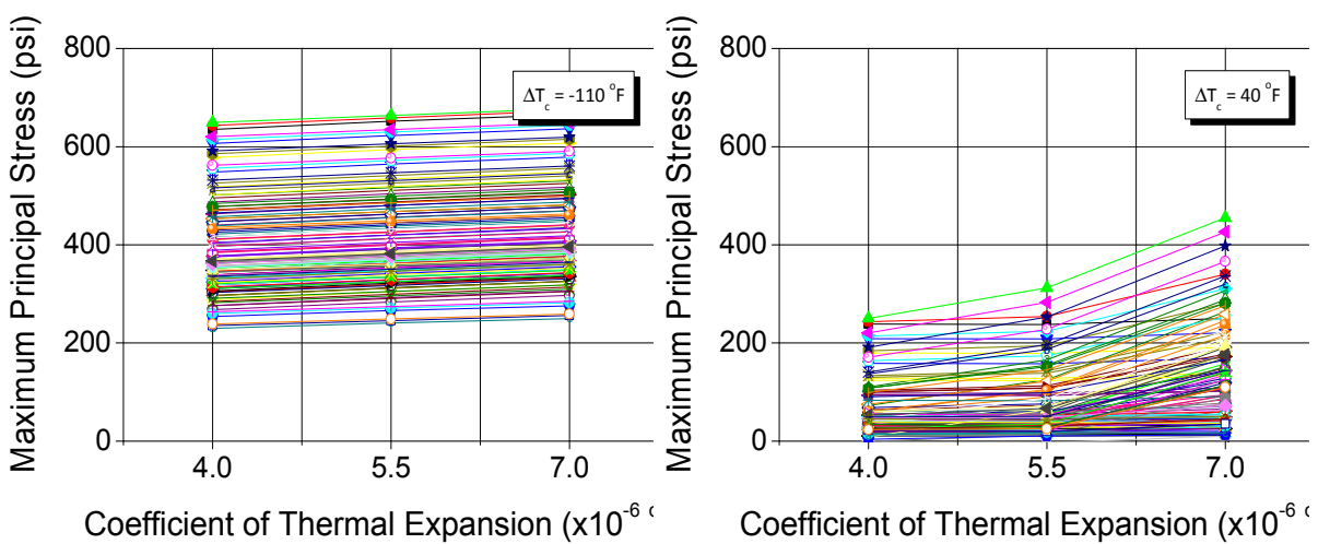
&lt;그림 16.8&gt; 열팽창계수의 영향
