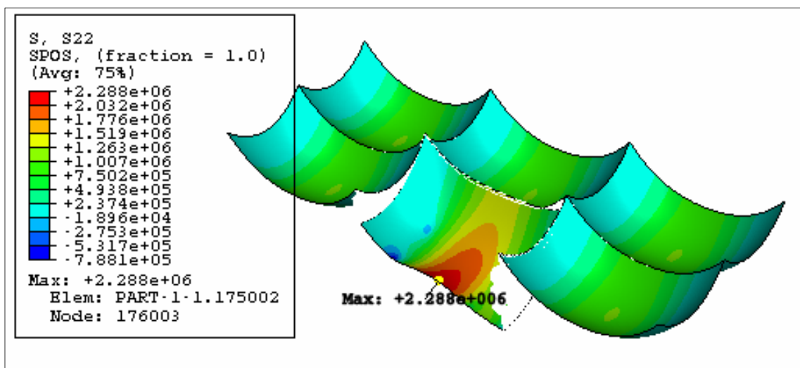
<그림 10.14> 하향균열을 유발하는 온도 및 차륜하중에 기인한 응력선도
