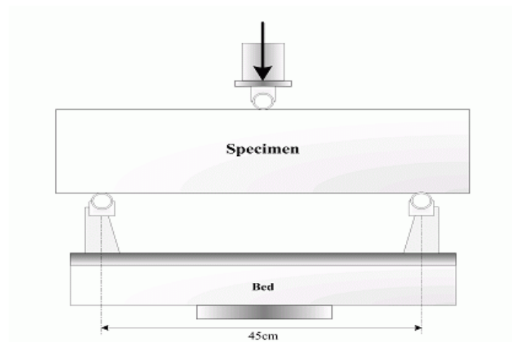
<그림 11.22> 휨인장 피로시험 개념도
