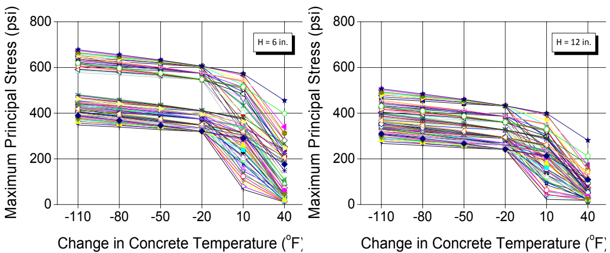
&lt;그림 16.7&gt; 콘크리트 온도 변화에 따른 영향
