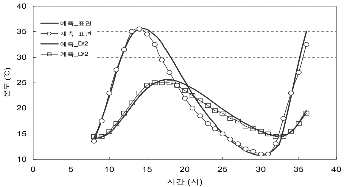
<그림 2.9> 충주지역의 온도예측 결과(봄)
