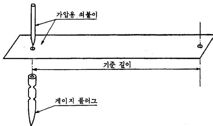
<그림 9.9> 가압용 쇠붙이
