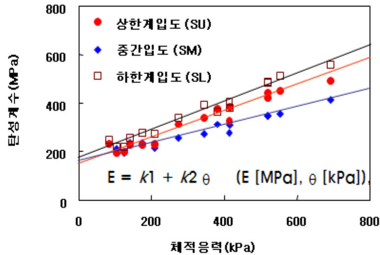
<그림 4.8> 채석기층의 일반적인 탄성계수
