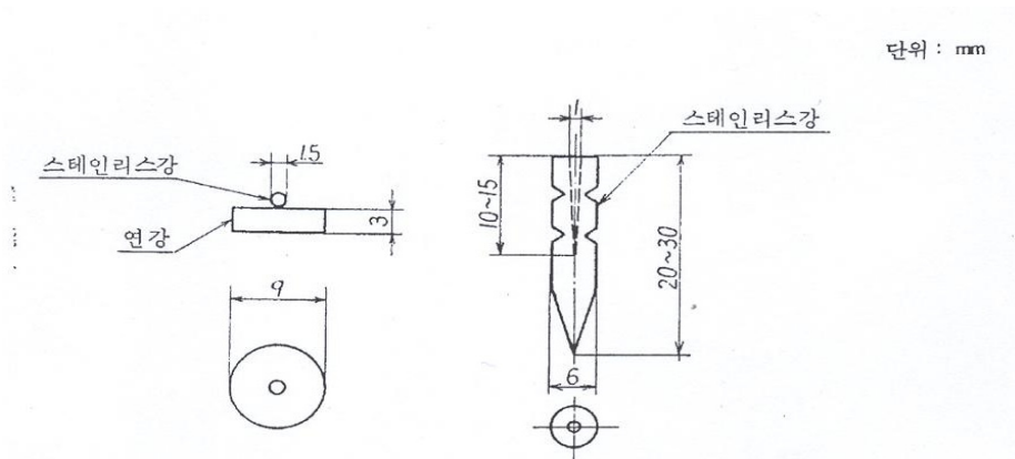
<그림 9.3> 콘택트 게이지 방법에 의한 게이지 플러그
