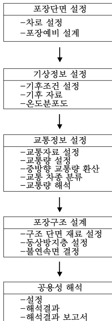
<그림 14.1> 설계흐름도
