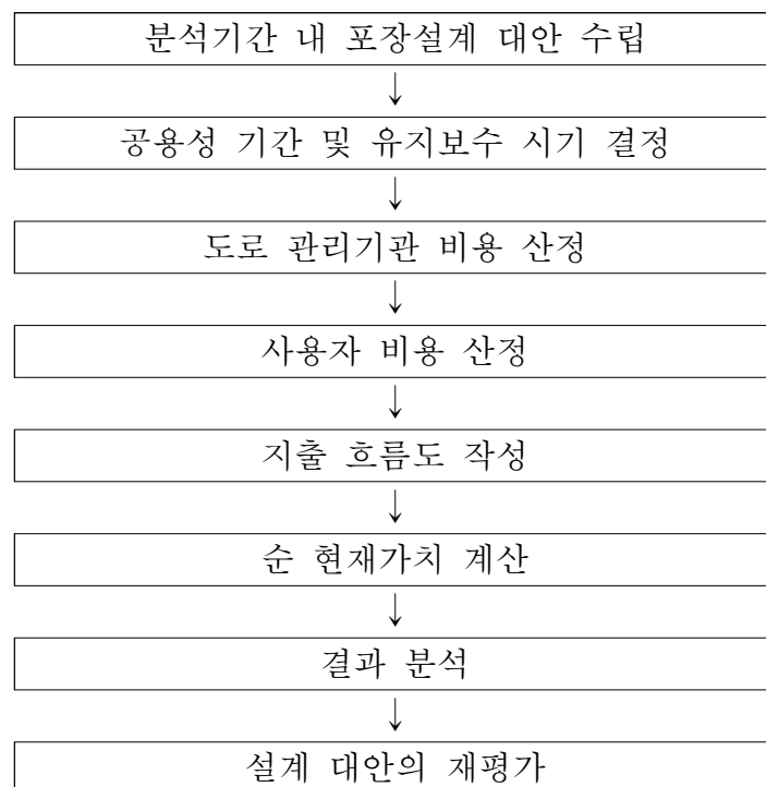
<그림 13.2> FHWA에서 제안하는 8단계 분석절차
