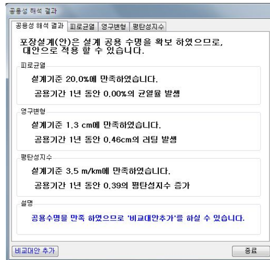
<그림 14.13> 공용성 해석 결과
