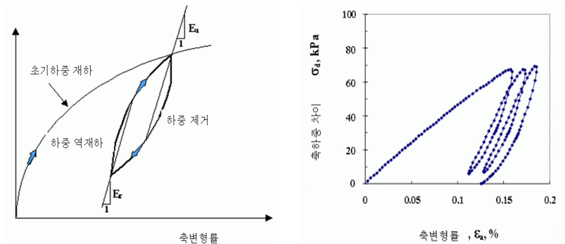
<그림 4.2> 회복탄성계수 시험에서의 탄성계수 결정
