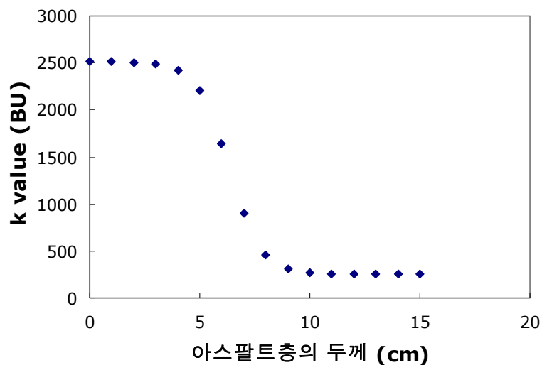
<그림 11.14> 상향균열의 두께 영향 변수 k의 변화
