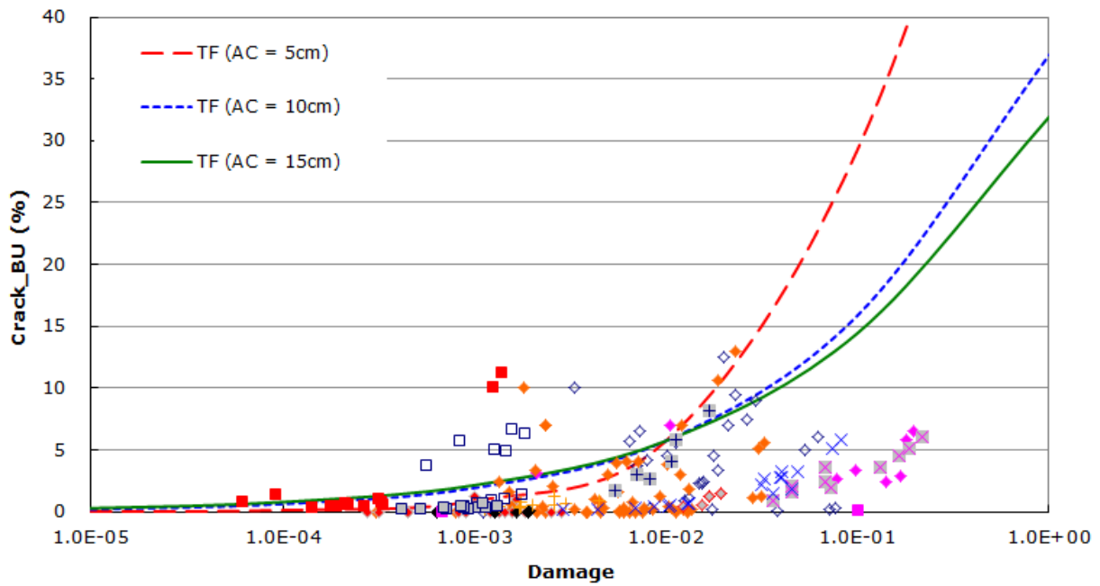
<그림 11.46> 상향균열에 대한 전이함수
