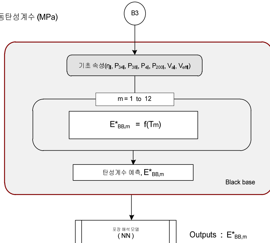
&lt;그림 4.5&gt; 아스팔트 안정처리기층(블랙 베이스) 탄성계수 결정 로직
