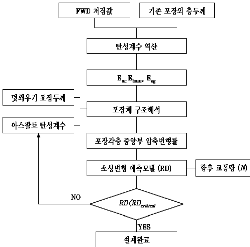
<그림 12.8> 아스팔트 콘크리트 덧씌우기 포장 설계에서 영구변형 예측 흐름도
