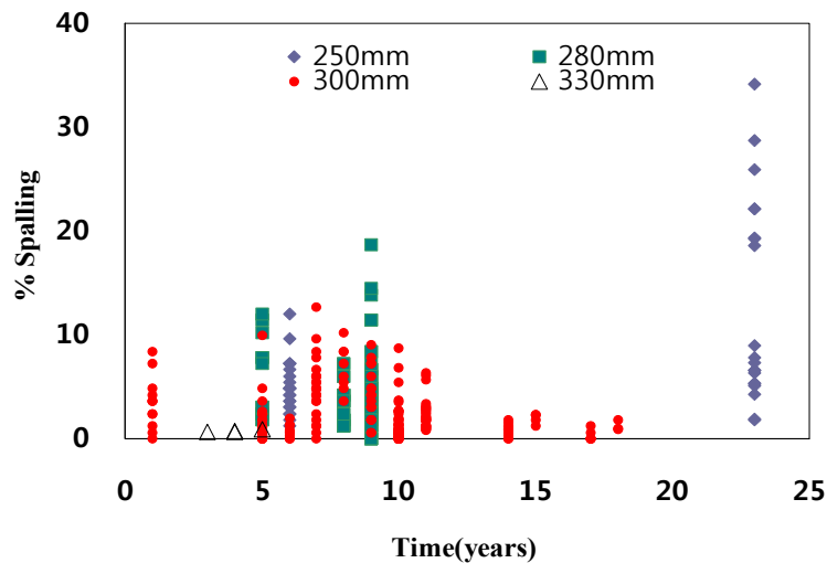
<그림 11.42> 재령에 따른 국내 시멘트 콘크리트 포장의 슬래브 두께별 스폴링 현황
