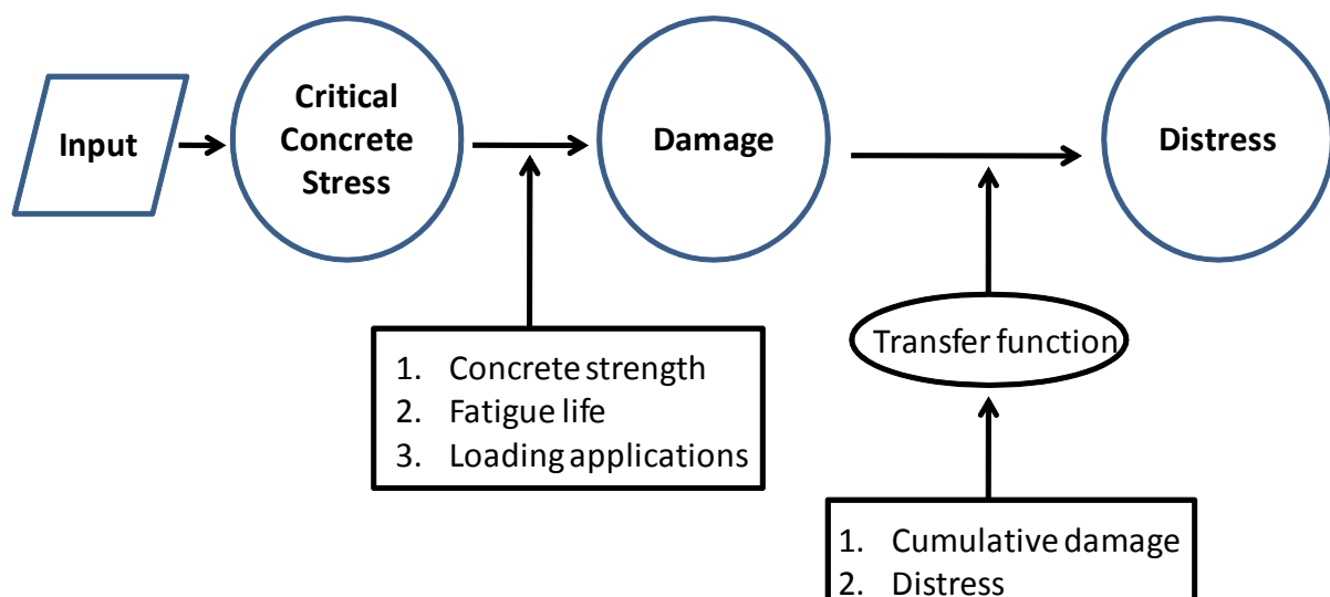
<그림 16.1> 역학적 경험적 연속철근 콘크리트 포장 설계의 아키텍처
