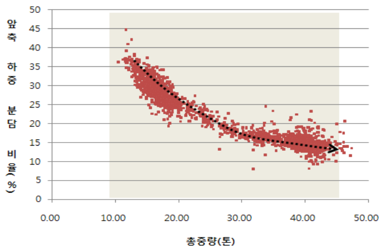
(b) 10종 트레일러 트럭의 앞축 하중 분담율
