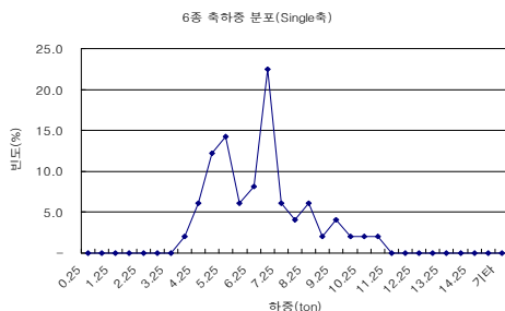
(c) 6종 Single 축 하중분포(11종 구분)
