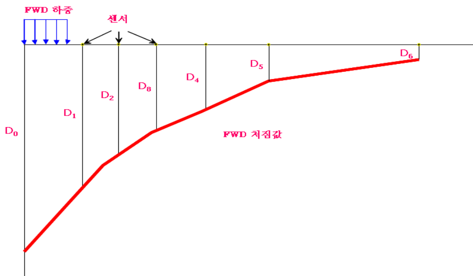
&lt;그림 12.3&gt; 포장 처짐량 측정
