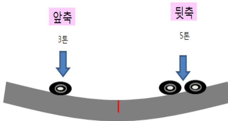
<그림 1.6> 시멘트 콘크리트 포장의 상향 컬링시 하향 균열 예측 위한 구조해석 형태
