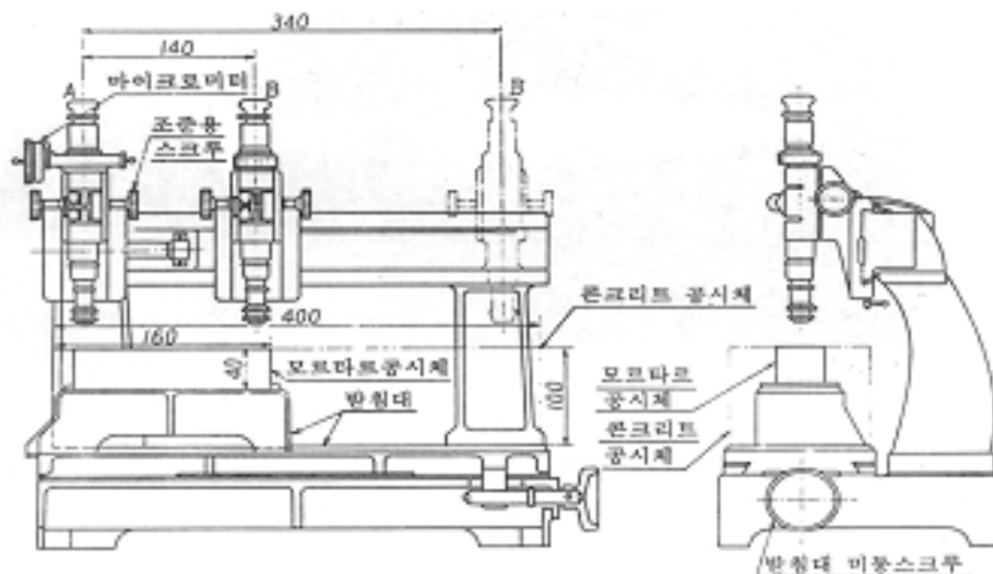
<그림 7.9> 콤퍼레이터 방법의 측정기
