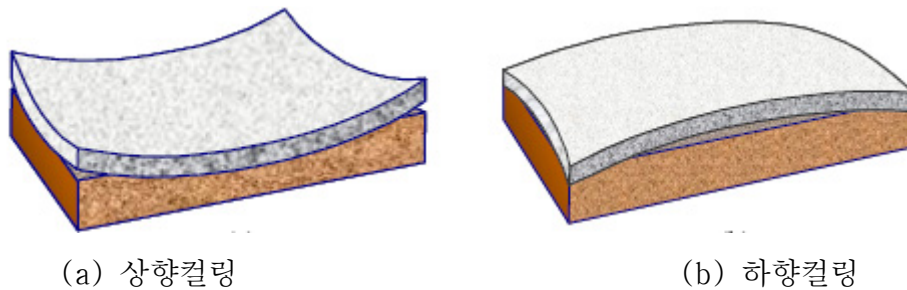
&lt;그림 10.9&gt; 슬래브 상하부 간의 온도 차이에 의한 컬링형태
