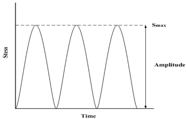
<그림 11.24> 최소응력( S_{min} )이 고려되지 않은 하중재하
