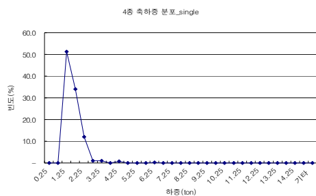
(a) 4종 Single 축 하중분포(11종 구분)
