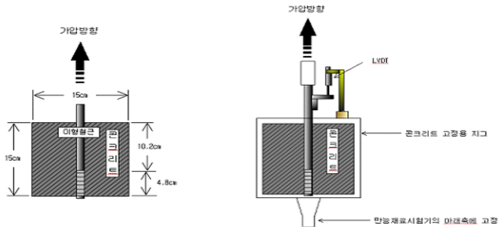
<그림 7.14> Tie-Bar의 콘크리트내 매립모습과 지그 및 LVDT 설치개념도
