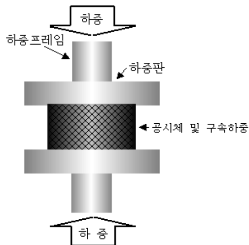
&lt;그림 5.7&gt; 구속반복하중 크리프 시험
