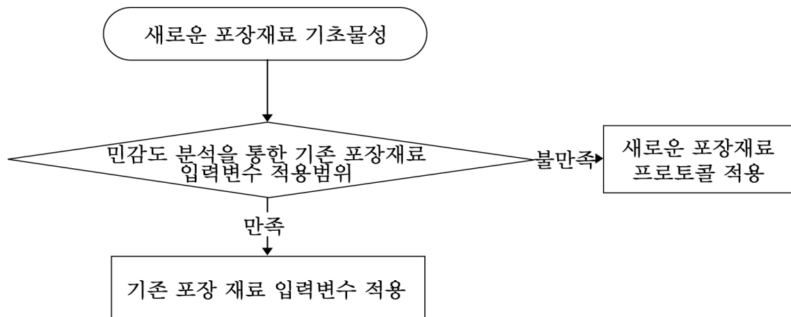
<그림 3.3> 새로운 시멘트 콘크리트 재료의 도입절차
