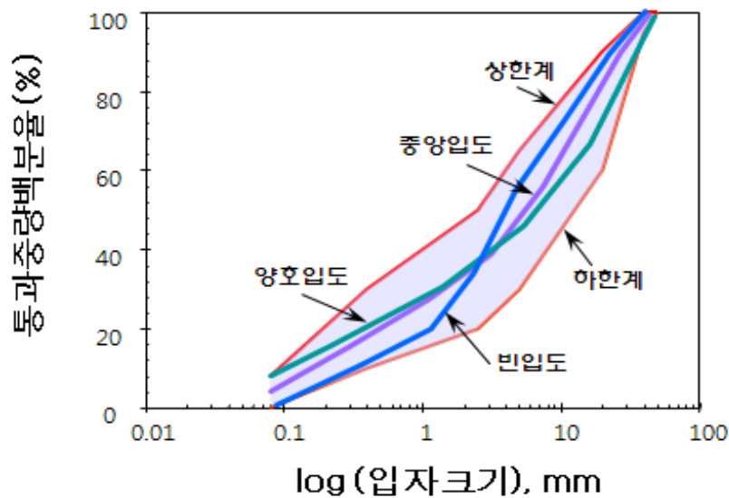
<그림 4.7> 쇄석기층 입도분포
