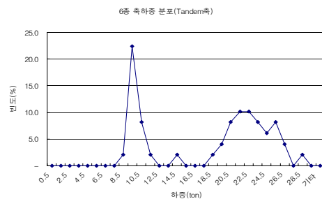
(d) 6종 Tandem 축 하중분포(11종 구분)
