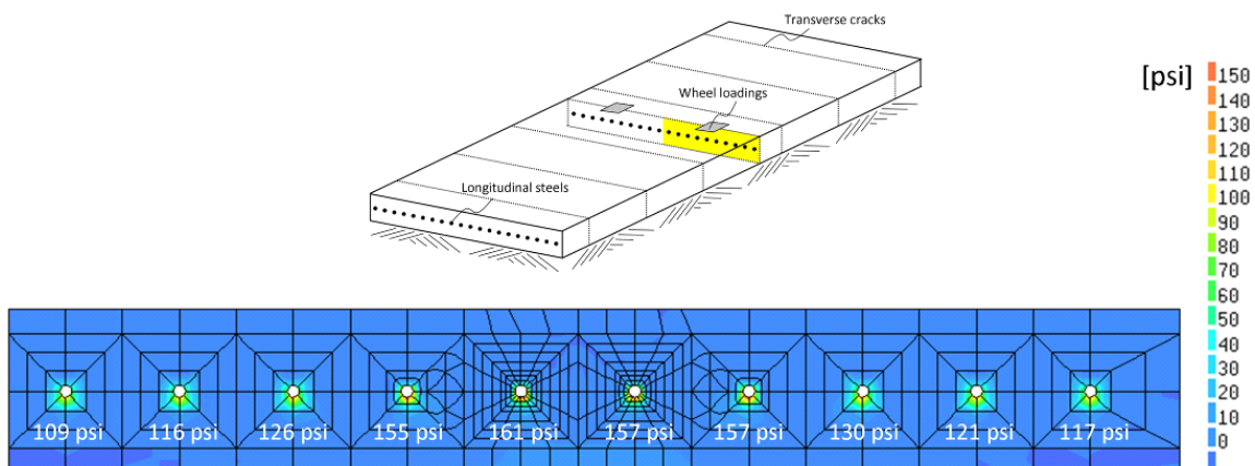
<그림 16.3> 구조해석 모형
