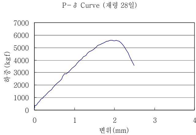
<그림 7.15> 재령 28일의 P-δ Curve
