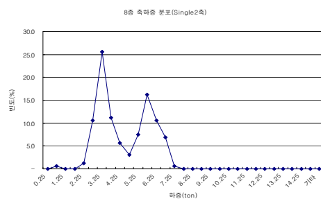
(f) 8종 Single2 축 하중분포(11종 구분)
