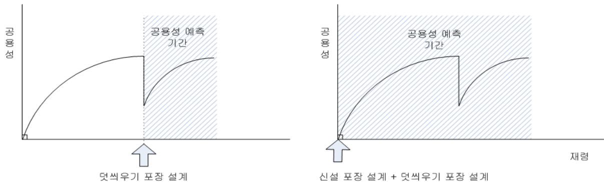
<그림 12.1> 기존 포장의 덧씌우기 설계 시점(좌) 및 단계건설에 필요한 덧씌우기 설계 시점(우)
