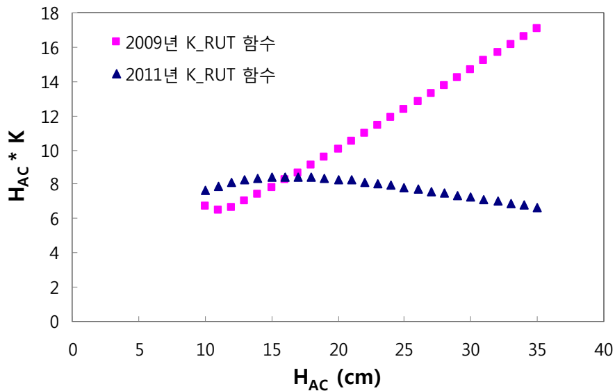
<그림 11.20> 아스팔트 층 두께에 따른 K 값의 변화
