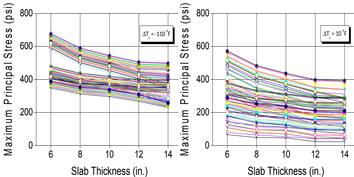
<그림 16.4> 슬래브 두께의 영향
