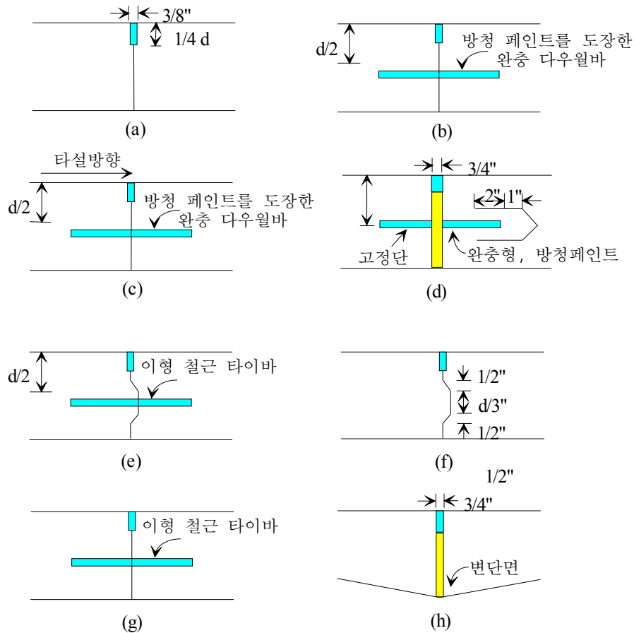
<그림 7.16> 다양한 불연속면 처리 형태
