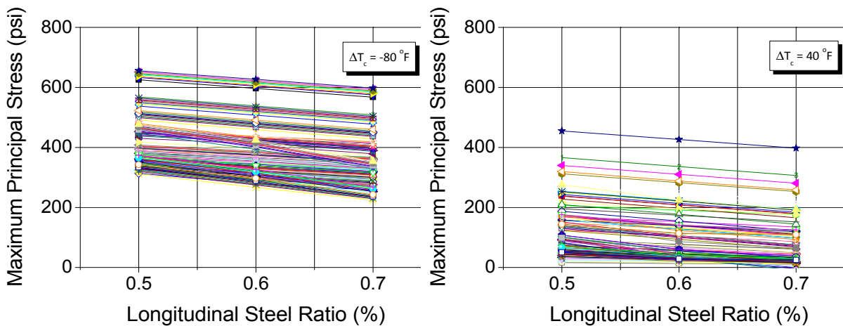
<그림 16.5> 종방향 철근비의 영향
