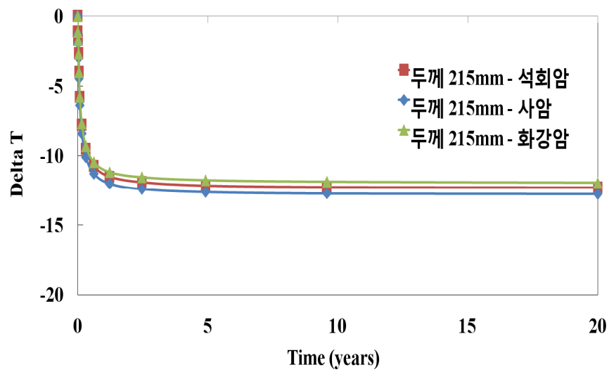
(a) 암종별 응력감소가 고려된 부등건조수축 예측량1(V/S= 215mm)
