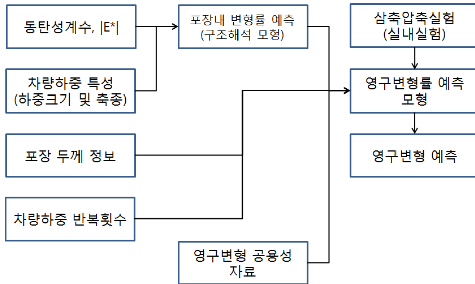
<그림 11.19> 영구변형 예측 순서도
