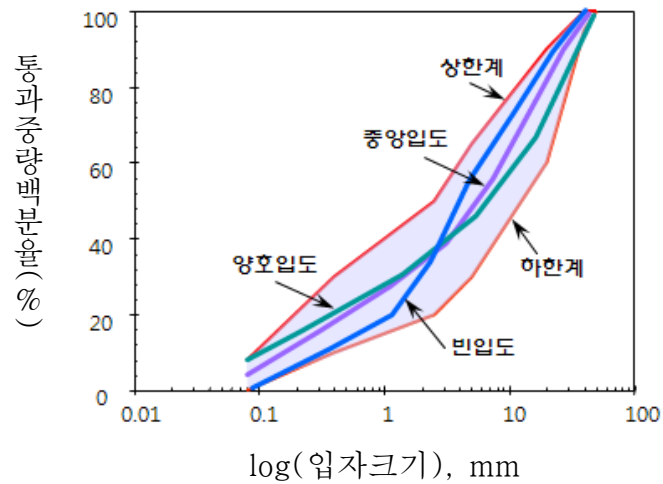
<그림 3.5> 쇄석기층 입도분포
