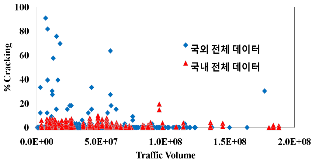
<그림 11.44> 교통량에 따른 국내 및 미국의 시멘트 콘크리트 포장 피로균열율 분포
