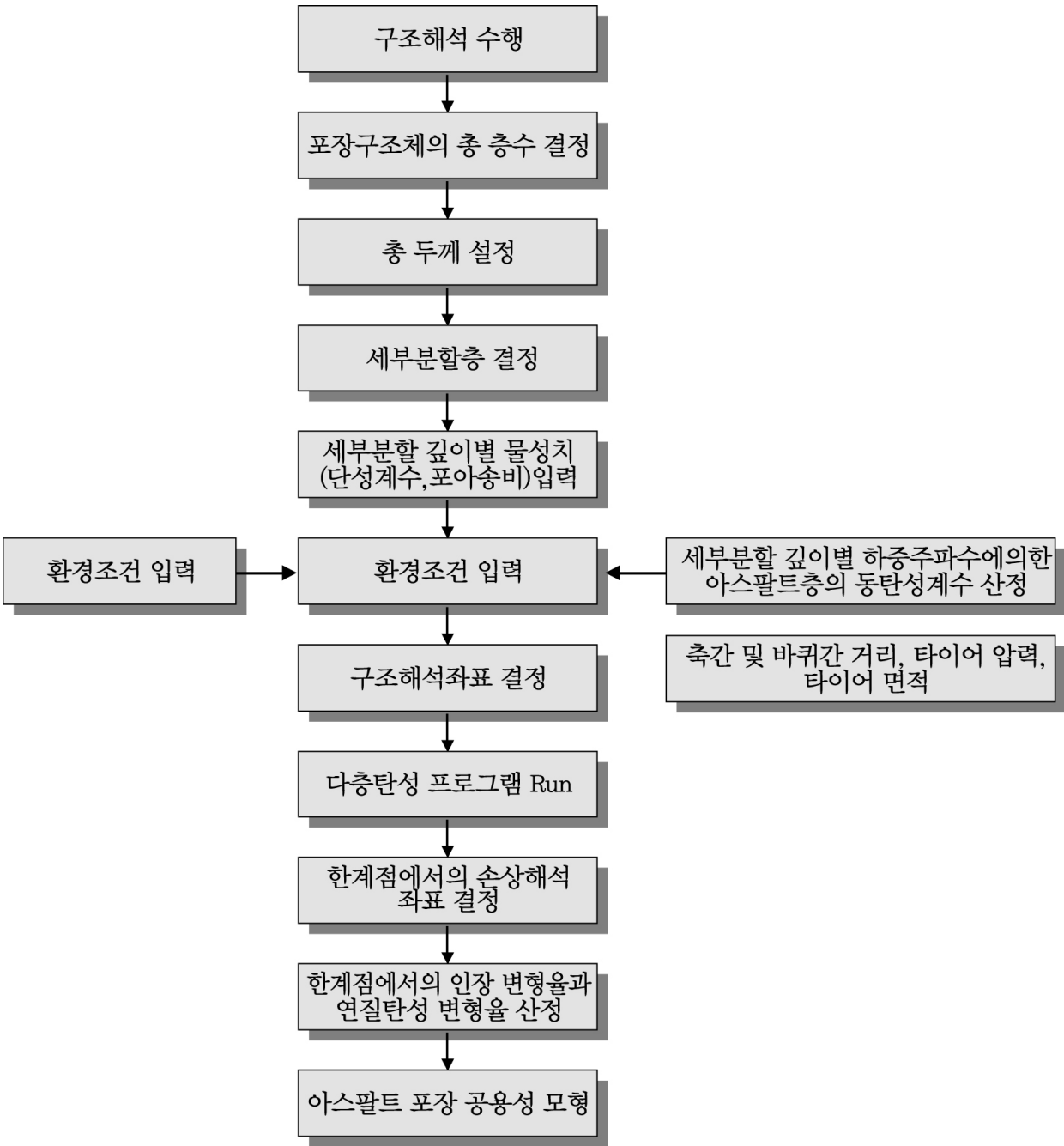
<그림 4.1> 아스팔트 콘크리트 포장 구조해석 절차
