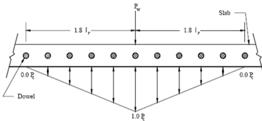
<그림 7.19> Friberg의 Dowel Group Action
