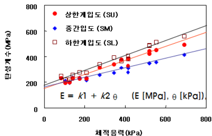
<그림 3.6> 쇄석기층의 일반적인 탄성계수
