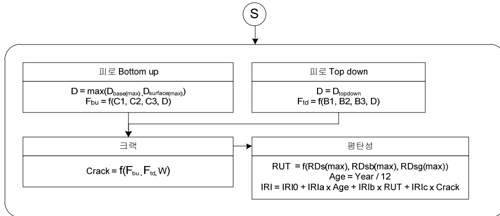
&lt;그림 11.4&gt; 아스팔트 콘크리트 포장층의 평탄성지수 산정 로직
