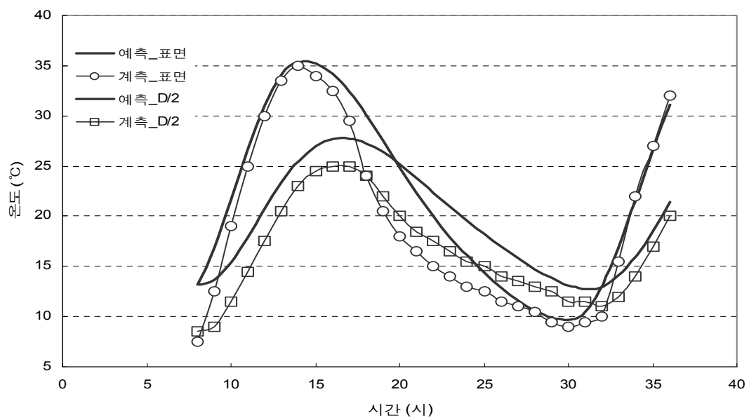
<그림 2.7> 진부령지역의 온도예측 결과(봄)
