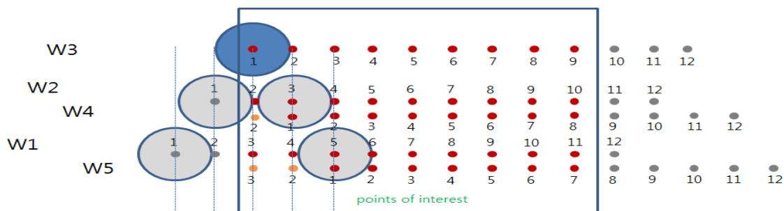
<그림 10.5> 단축단륜 조건에서의 원더링에 따른 대상 측점의 변화
