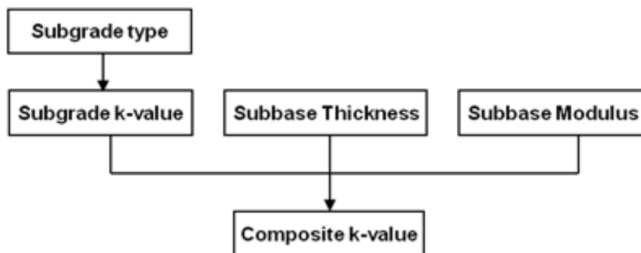
&lt;그림 16.2&gt; 하부지지력 산정 로직
