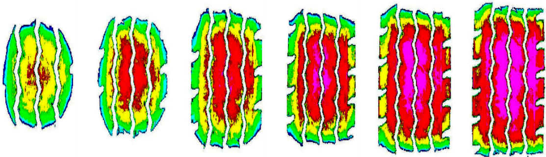
<그림 1.8> 축하중 크기에 따른 접지 면적의 변화
