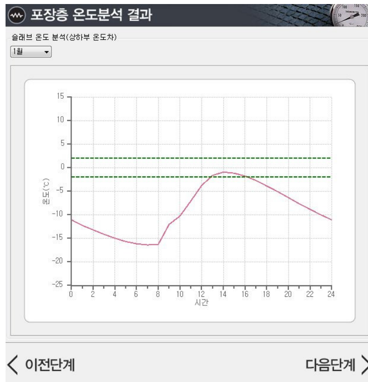
<그림 15.7> 포장층 온도분석 결과
