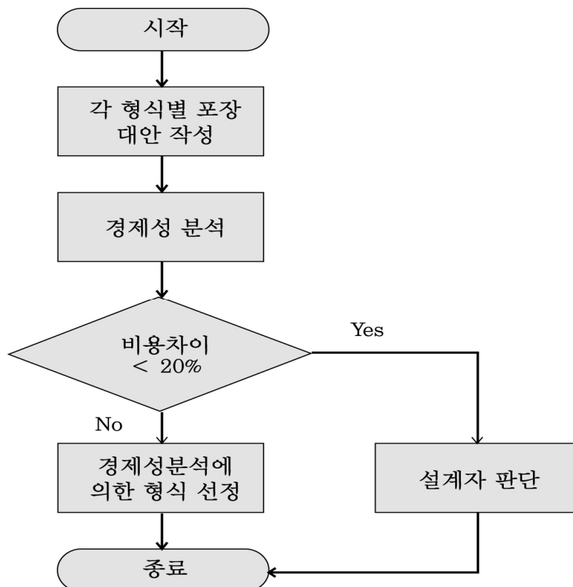
<그림 2.5> 포장형식 선정 절차
