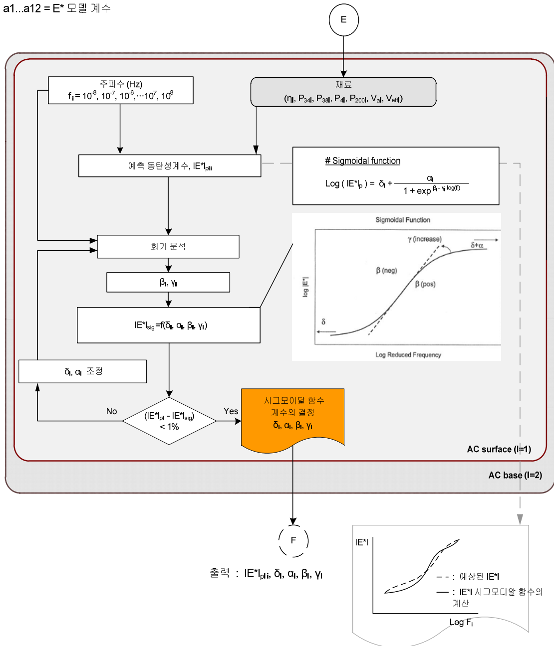
<그림 5.3> 아스팔트 층의 동탄성계수 결정 로직
