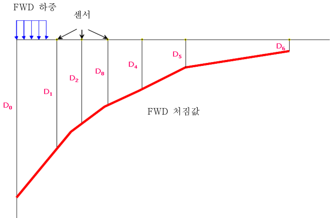
<그림 8.4> 포장 처짐량 측정
