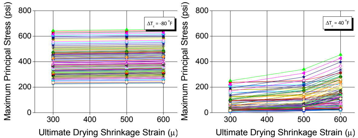
&lt;그림 16.9&gt; 최종건조수축의 영향
