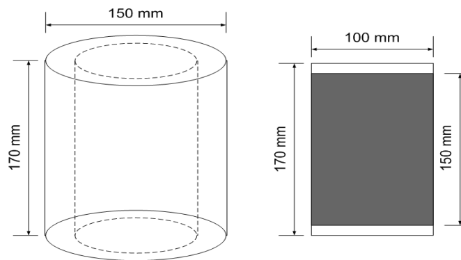
<그림 11.17> 영구변형 시험용 시편의 제작
