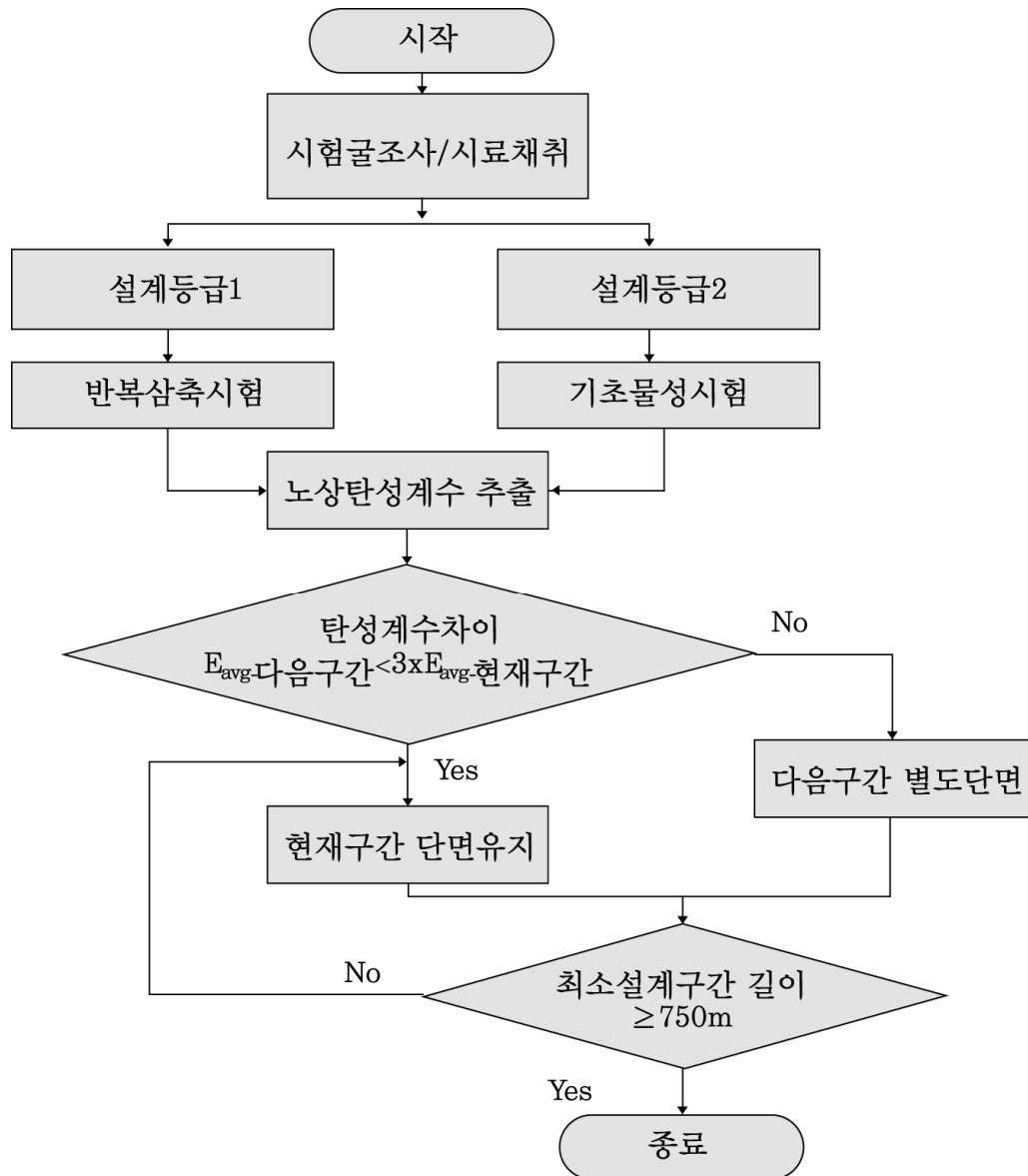
<그림 2.1> 포장설계구간 연장 결정 절차
