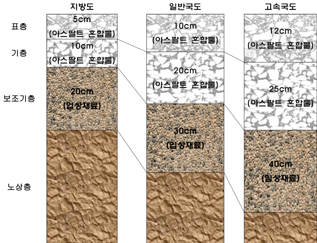
<그림 2.6> 아스팔트 콘크리트 포장의 기본 설계 단면
