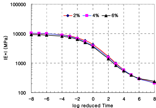
<그림 5.2> 마스터 곡선 (화강암 밀입도 13mm + PG 58-22)
