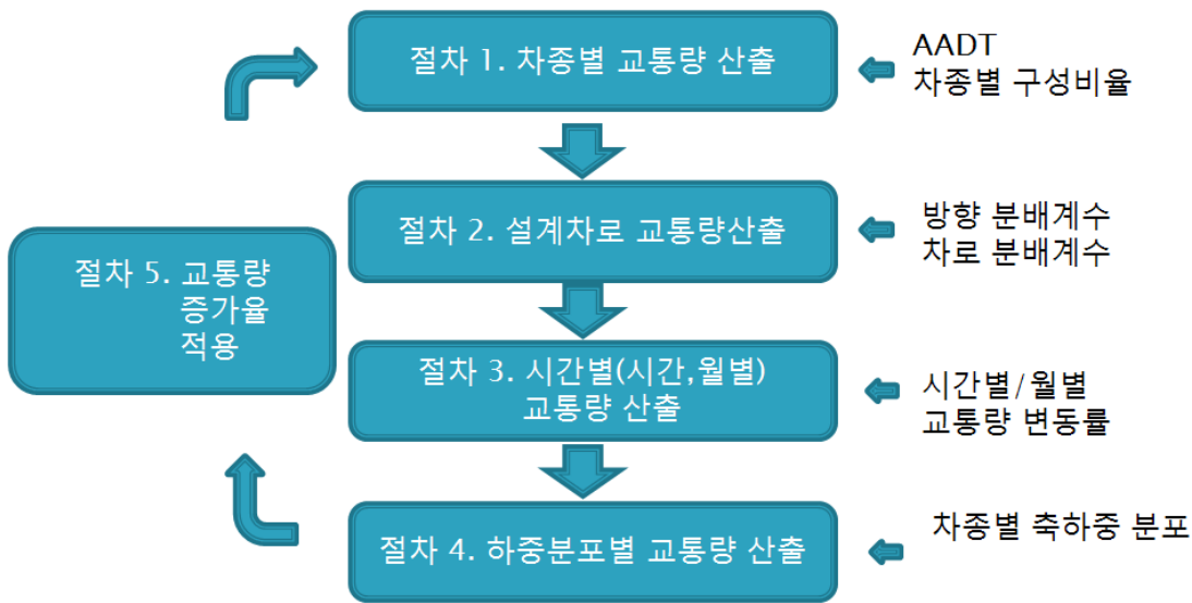
&lt;그림 1.12&gt; 도로포장 설계의 교통량 산출 개념도
