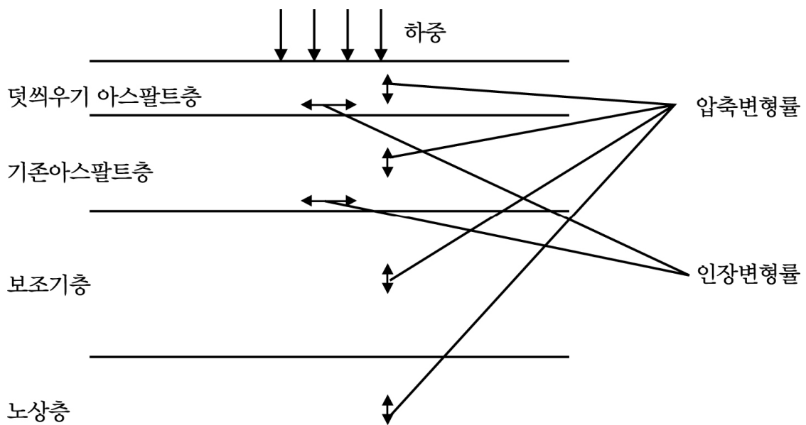
<그림 8.3> 아스팔트 덧씌우기 포장 구조해석
