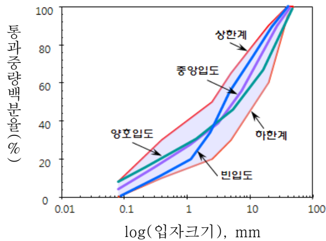
<그림 3.3> 쇄석기층 입도분포
