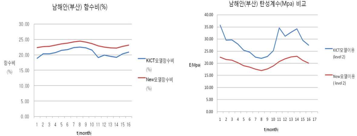
&lt;그림 2.11&gt; 함수비 변화에 따른 탄성계수 변화 비교(남해안)
