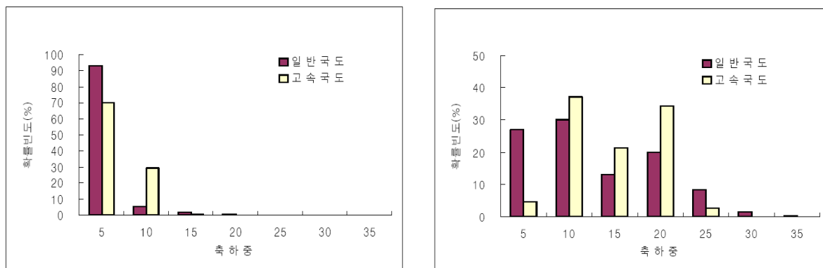
<그림 1.5> 단축 및 복축복륜의 축하중(톤) 비교
