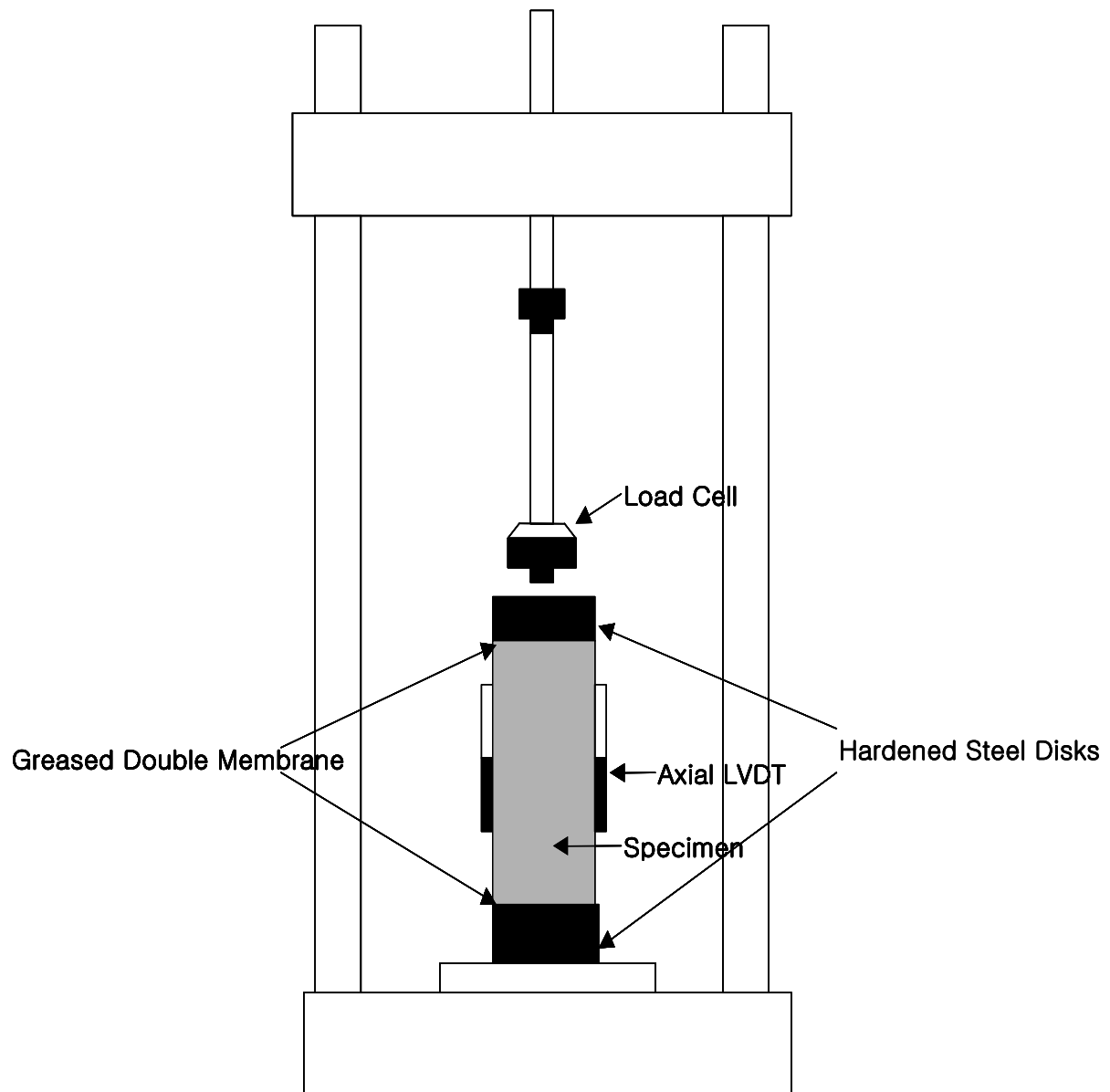
<그림 6.1> 동탄성계수 시험기기 세팅
