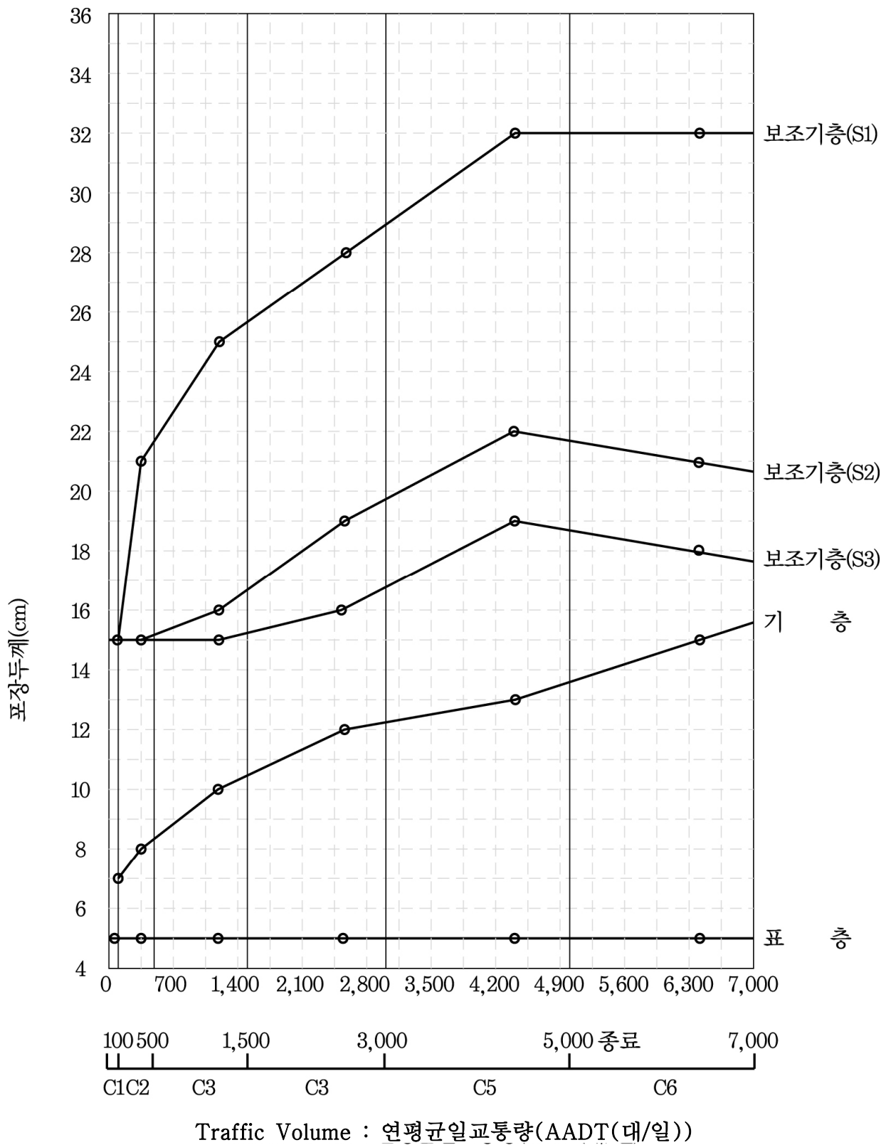
&lt;그림 7.2&gt; 아스팔트 콘크리트 포장의 카달로그 설계그래프
