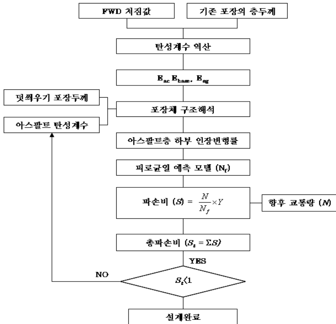
<그림 12.7> 아스팔트 덧씌우기 포장에서 피로균열 예측 흐름도
