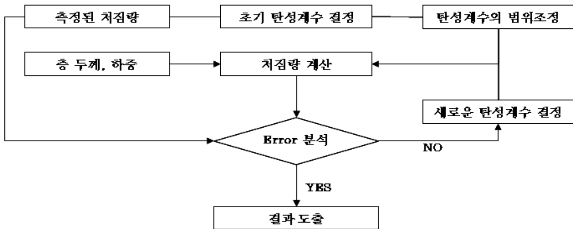
<그림 12.4> 포장층 탄성계수 역산 절차
