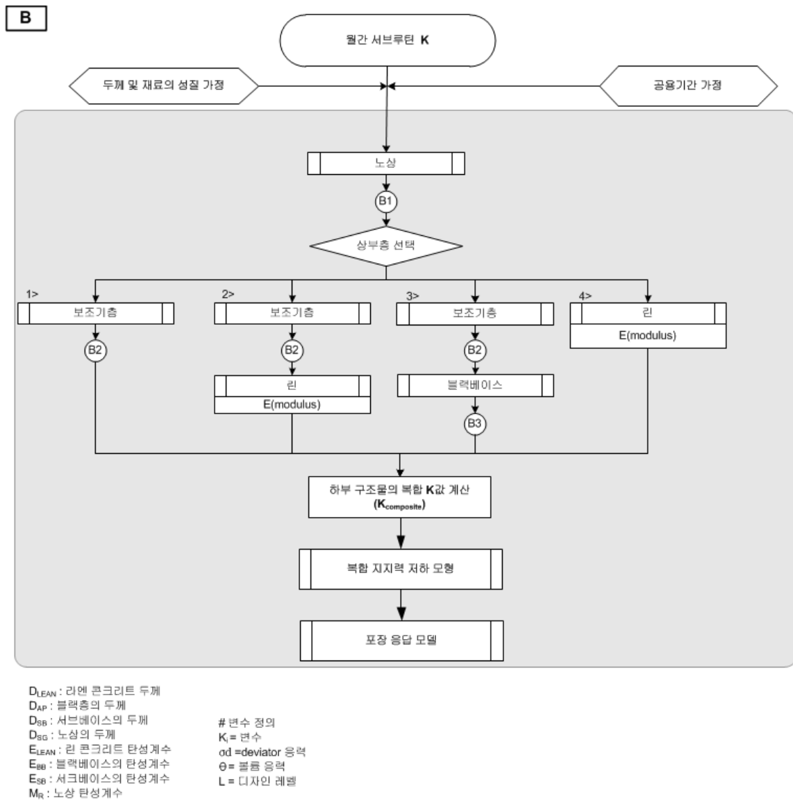
<그림 4.6> 콘크리트 포장 복합 지지력 산정 로직
