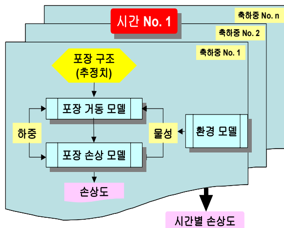
<그림 11.7> 시간별 손상계산
