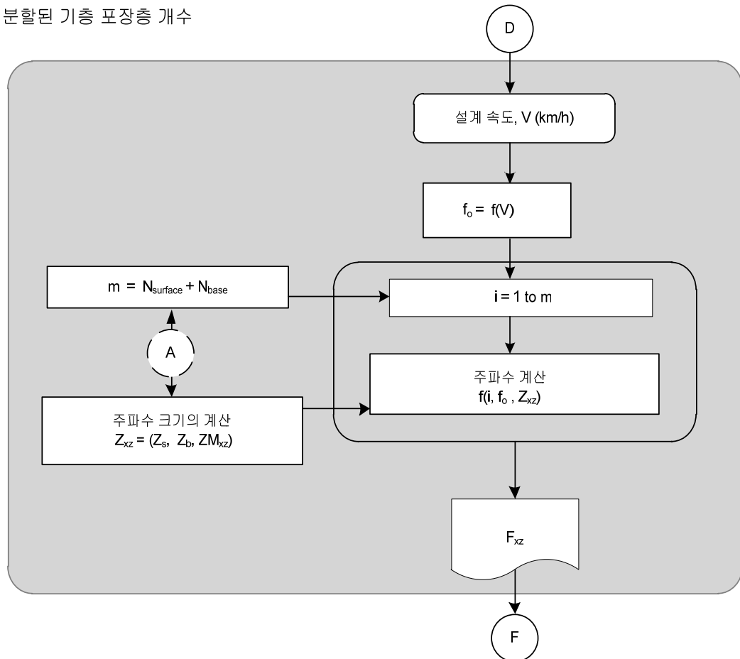
<그림 1.15> 아스팔트 포장의 하중주파수 계산 로직
