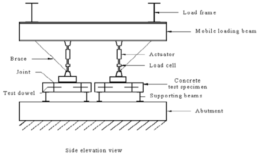
<그림 7.22> 실내의 하중전달 장치 성능평가 실험 개념도
