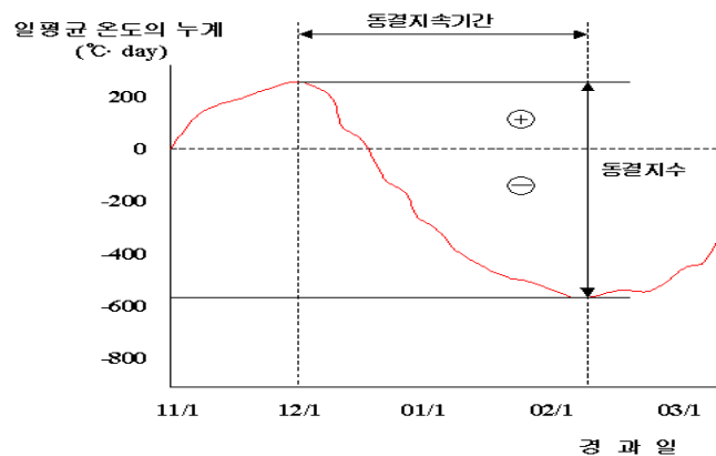
<그림 4.11> 동결지수 산정 방법
