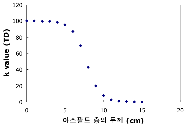
<그림 11.15> 하향균열의 두께 영향 변수 k 의 변화
