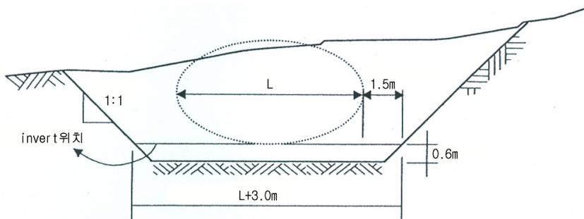
그림 5-2-13 기초지반을 굴착하여 설치하는 경우 구조적 뒤채움 영역
