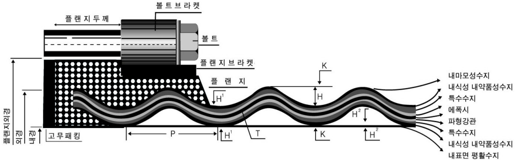
그림 5-2-6 수지파형강관 단면도(평활형)
