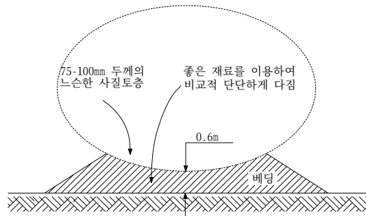
그림 5-2-11 베딩 시공
