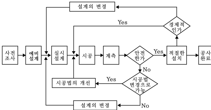
그림 7-10-1 계측관리 계획도
