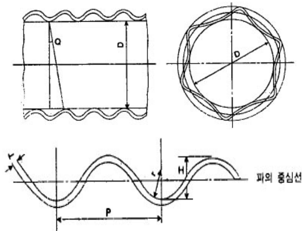
그림 5-2-4 수지파형강관의 단면 모양
