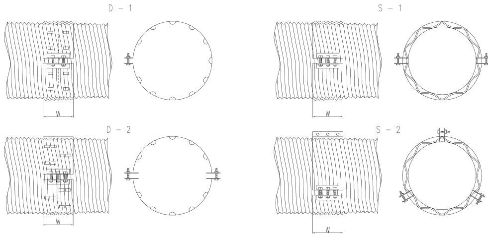
그림 5-2-3 커플링 밴드 형상
