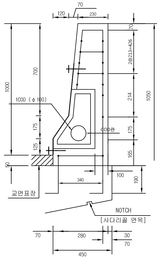
폴박스 설치 방호벽 단면도 1 COD(Φ 100)
