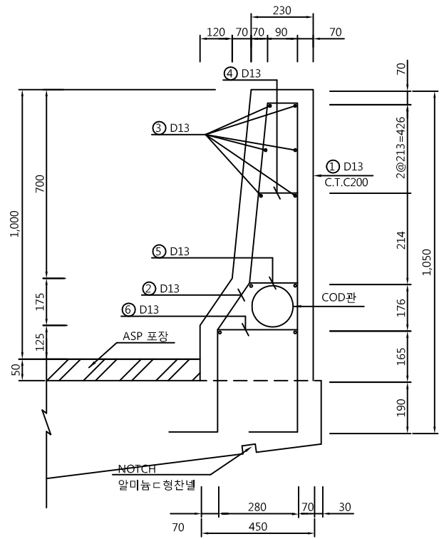
방 호 벽[2] H=1.0 [기계타설] 단 면 도
