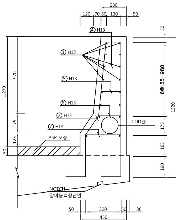
방 호 벽[3] H=1.270 [인력타설] 단 면 도
