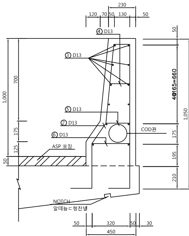
방 호 벽[1] H=1.0 [인력타설] 단 면 도
