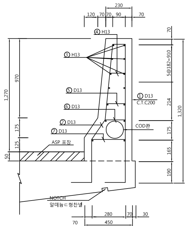
방 호 벽[2] H=1.270 [기계타설] 단 면 도
