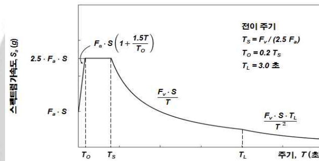
그림 4.3-3 토사지반 수평설계지반운동의 가속도 표준설계응답스펙트럼(5% 감쇠비)
