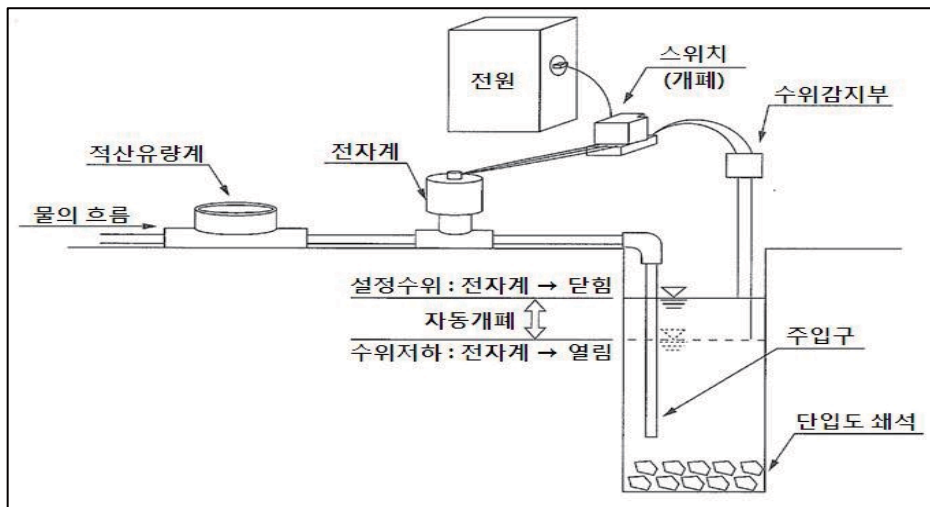
<그림 4-7> 정수위법에 의한 침투실험 상황
