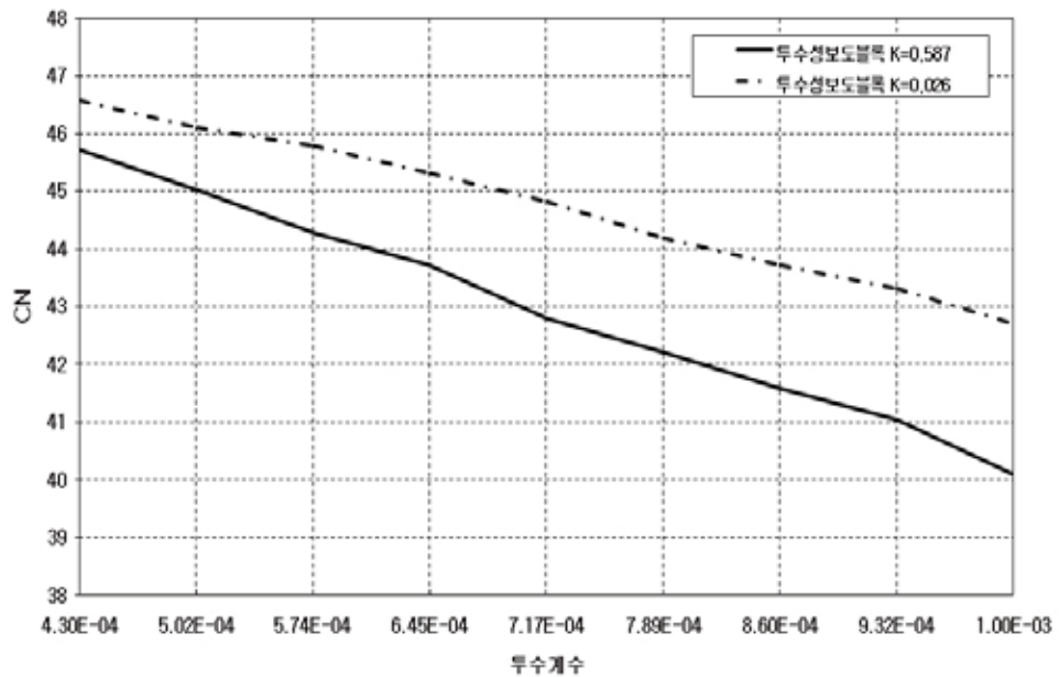
<그림 4-15> 하부토양 투수계수별 CN
