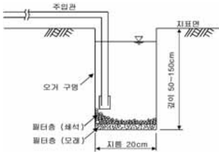
<그림 4-4> Bore-hole법을 이용하는 시험시설
