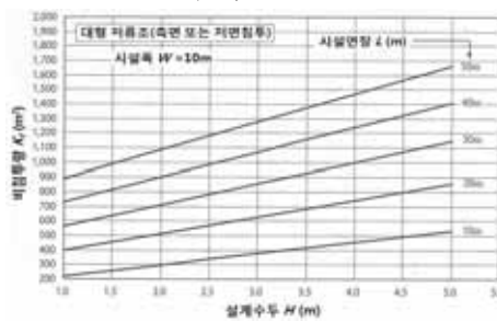
(g) 대형 저류조(측면 또는 저면침투)
