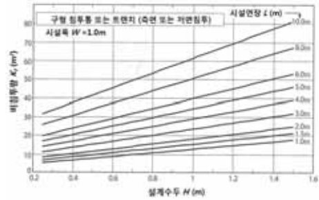
(f) 구형 침투통 또는 트렌치(측면 또는 저면침투) 시설폭 W=1.0m
