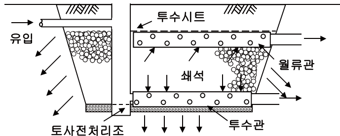
&lt;그림 3-8&gt; 쇄석공극 저류침투시설
