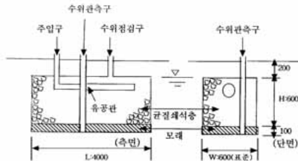
<그림 4-6> 실물시험시설의 예
