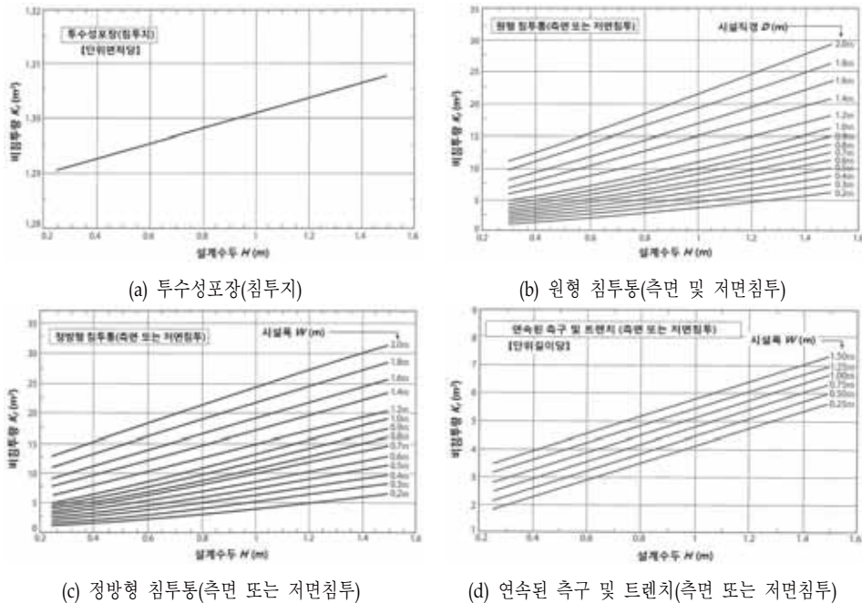
<그림 4-10> 침투시설별 비침투량
