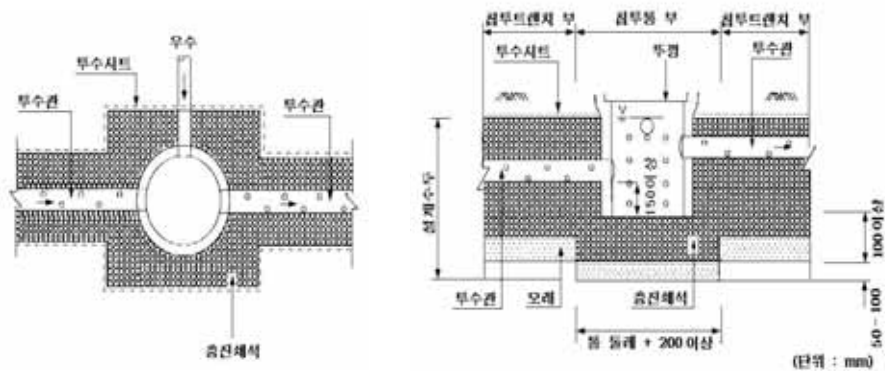
<그림 4-17> 조합하여 설치하는 경우의 표준구조
