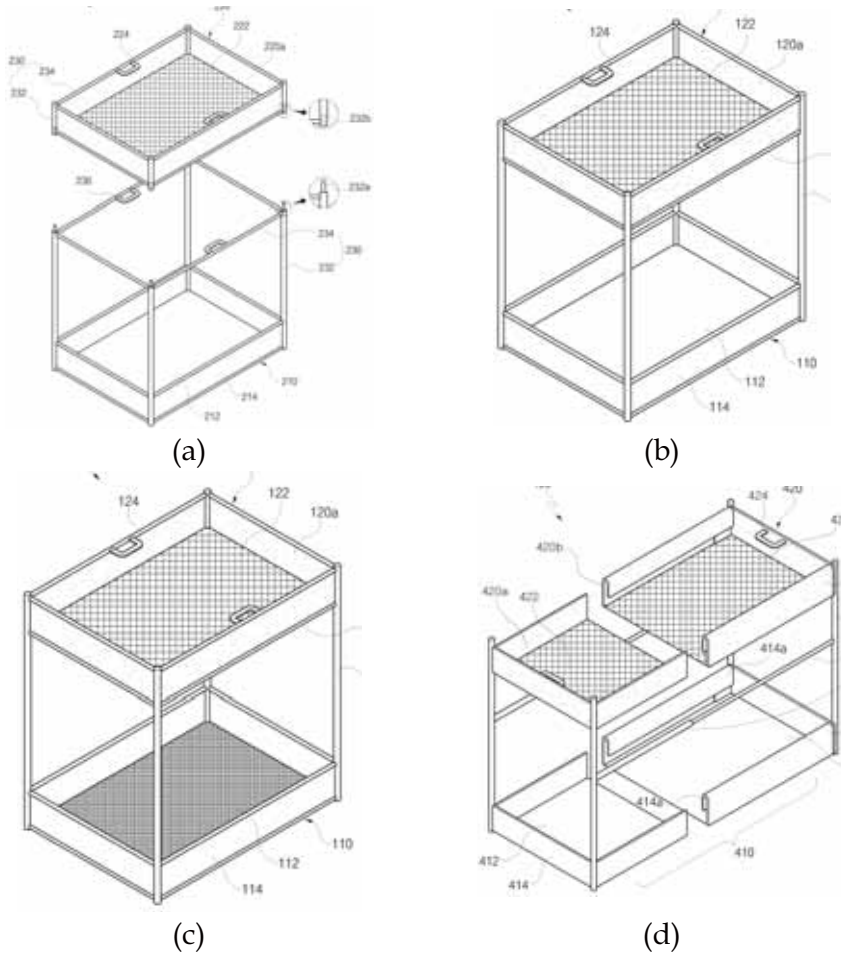
&lt;그림 4-19&gt; 집수정 유지관리구 개요도
