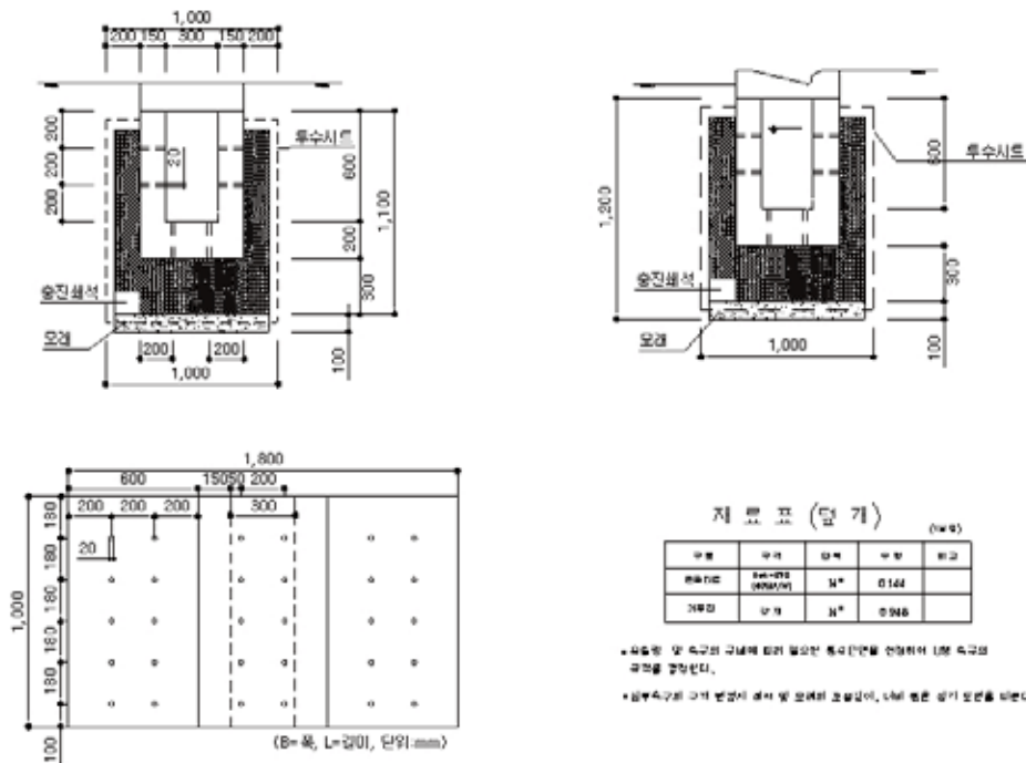
<그림 4-29> 침투측구 표준단면도
