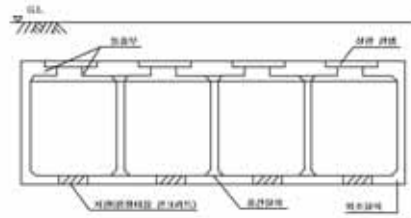
<그림 3-7> 전용 저류시설 시공 및 단면(예)
