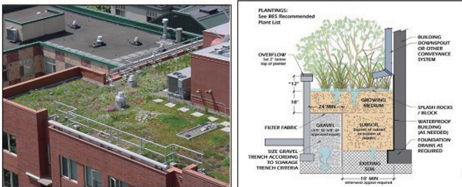
<그림 3-11> 지붕녹화 개념도
