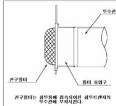
<그림 4-18> 막힘방지 장치 중 상부필터(上), 저부필터(左下), 관구필터(右下)의 예
