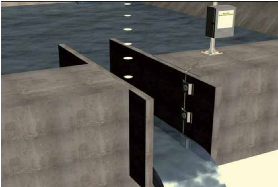
<그림 3-19> 전자과 유속계를 이용한 유속, 유량 측정
