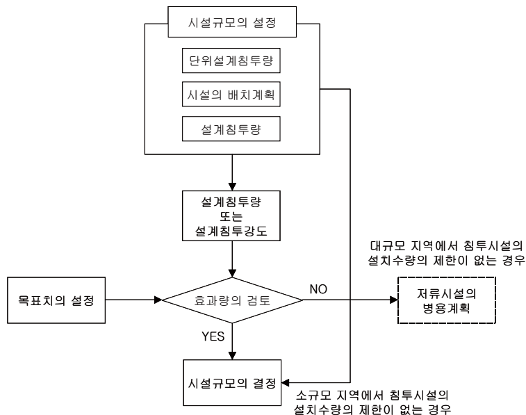
<그림 4-9> 침투시설 규모 결정 절차
