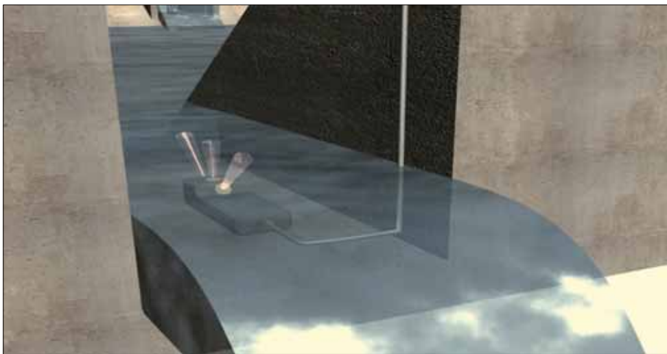
<그림 3-17> 도플러 방식의 초음파센서 (유속, 수심 프로파일 측정)를 이용한 유속, 유량 측정
