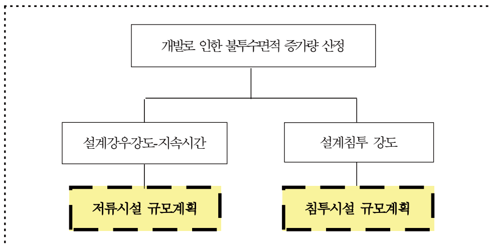
<그림 1-2> 지역내 저류시설 계획절차
