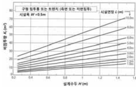
(e) 구형 침투통 또는 트렌치(측면 또는 저면침투) 시설폭 W=0.5m
