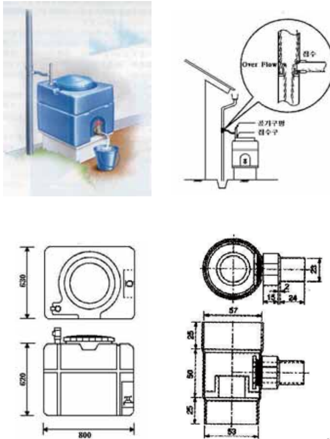
<그림 3-9> 주택단위 저류시설(탱크)
