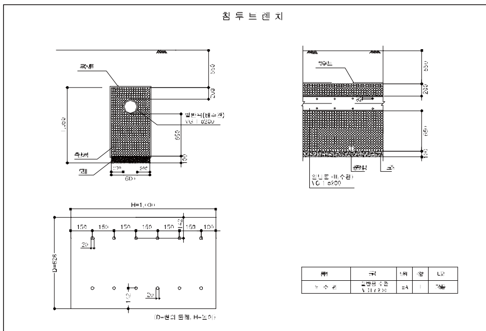
<그림 4-26> 침투트렌치 표준단면도
