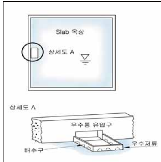
<그림 3-10> 지붕저류의 개념도
