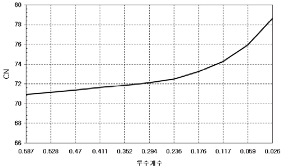
<그림 4-14> 투수성 보도블록 투수계수별 CN
