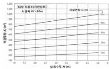
(h) 대형 저류조(저면침투)
