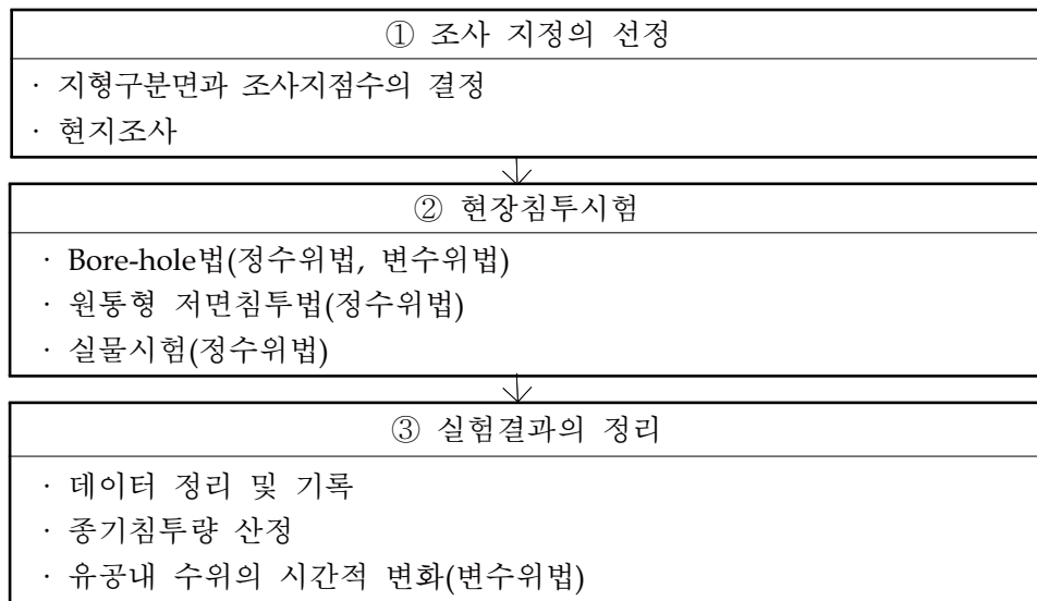
&lt;그림 4-3&gt; 현장침투시험 절차
