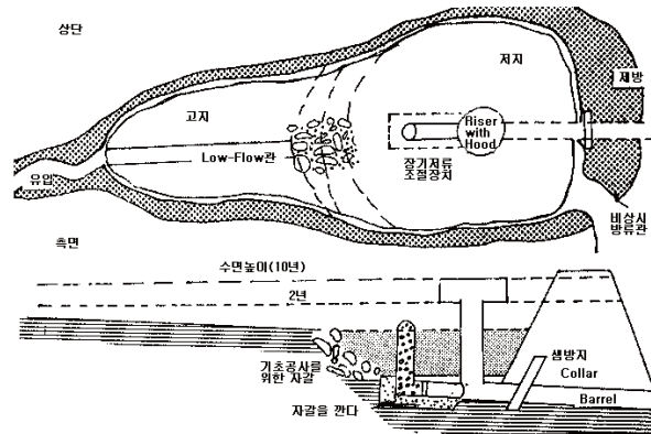
〈그림 3-2〉 다용도 건식저류지 개념도
