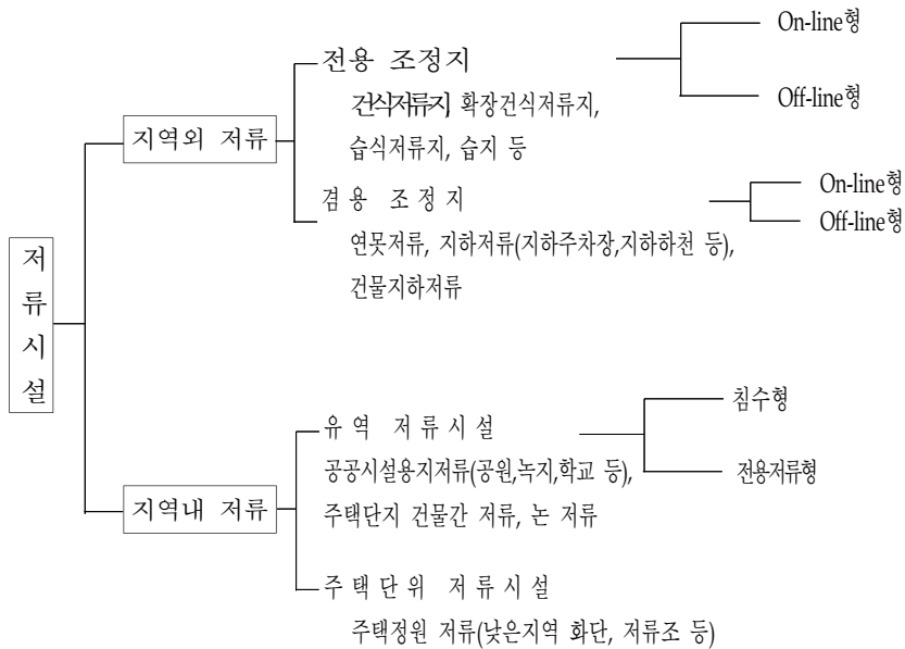
<그림 3-1> 저류시설의 종류
