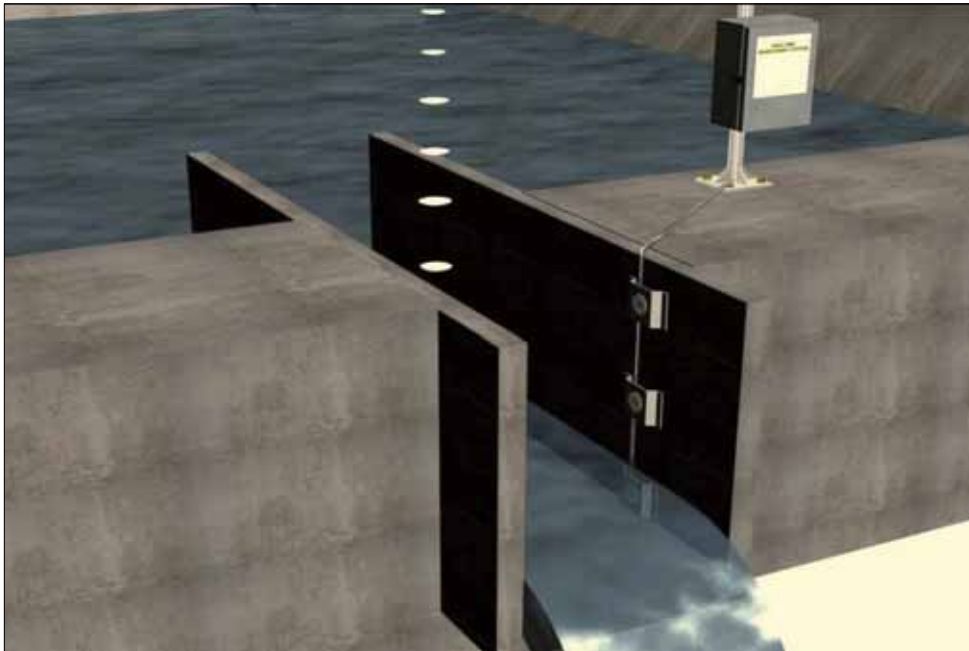
<그림 3-18> 전자기(Electro Magnetic) 센서를 이용한 유속, 유량 측정
