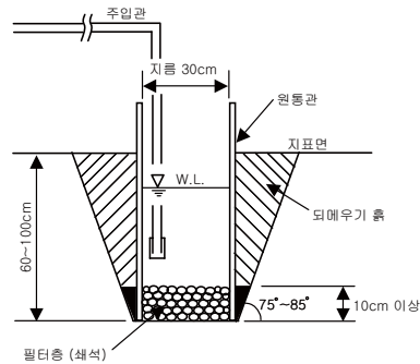
<그림 4-5> 저면침투법을 이용하는 시험시설
