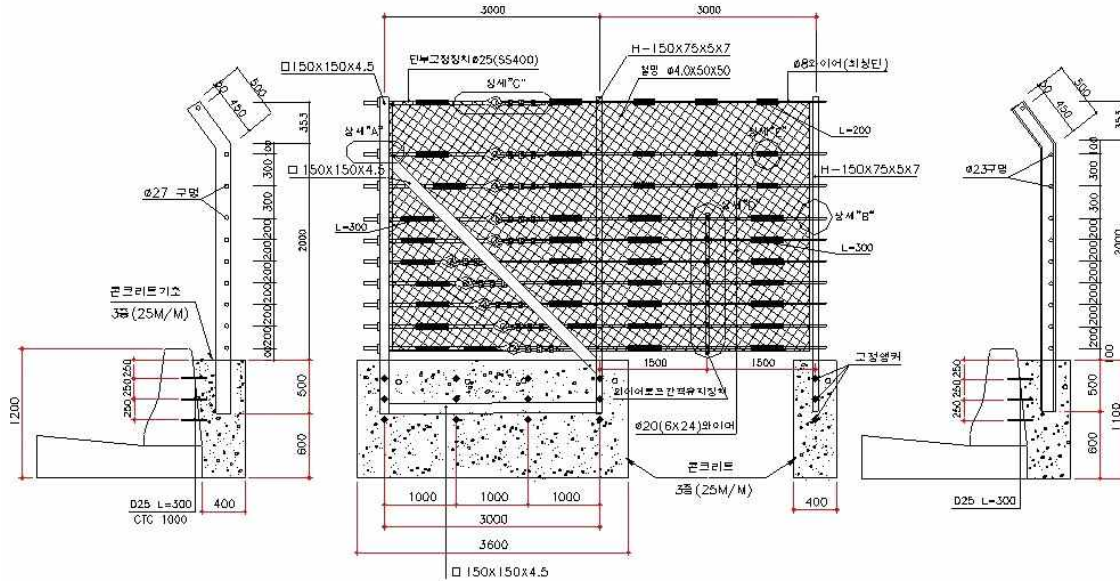
낙석방지울타리 (TYPE-2)
