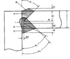
(7) k형 모서리이음용접
