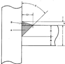
(11) 베벨형 부분용접 T이음용접
