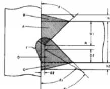
(9) k형 T이음용접
