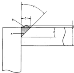
(12) 베벨형 부분용접 모서리이음용접
