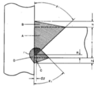
(8) 베벨형 T이음용접
