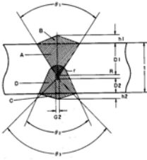
(5) x형 판이음용접
