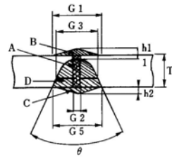
(2) I 형 판이음용접
