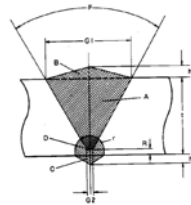
(4) V 형 판이음용접
