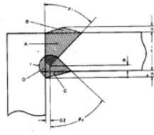
(6) 베벨형 모서리이음용접
