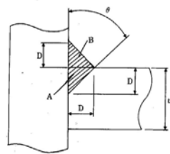
(13) 베벨형 부분용접과 모서리이음용접의 병용
