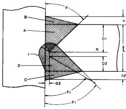
(9) K형 T이음용접
