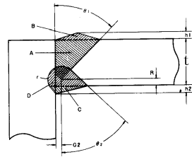
(6) 베벨형 모서리이음용접
