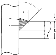
(11) 베벨형 부분용입 T이음용접
