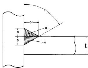
(10) 베벨형 필렛 T이음용접
