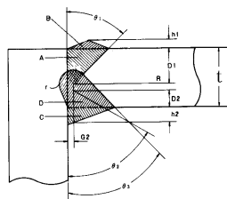
(7) K형 모서리이음용접
