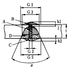
(2) I형 판이음용접
