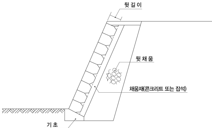
[돌쌓기 표준도]
