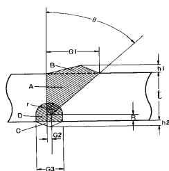
(3) 베벨형 판이음용접
