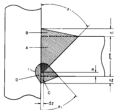
(8) 베벨형 T이음용접
