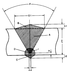
(4) V형 판이음용접
