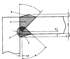
(6) 베벨형 모서리이음용접
