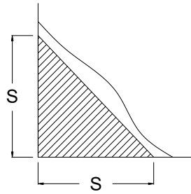
(1) 필렛용접
