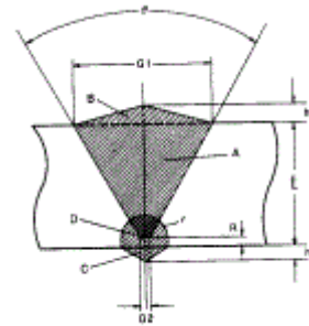
(4) V형 판이음용접
