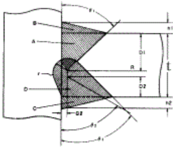
(9) K형 T이음용접
