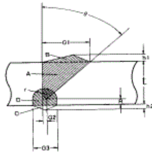
(3) 베벨형 판이음용접
