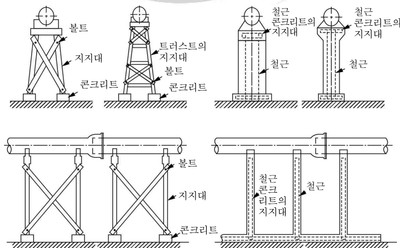
그림 3.3-1 지하매설물 보호도(예시) : 가스관 보호도(받치는 경우)
