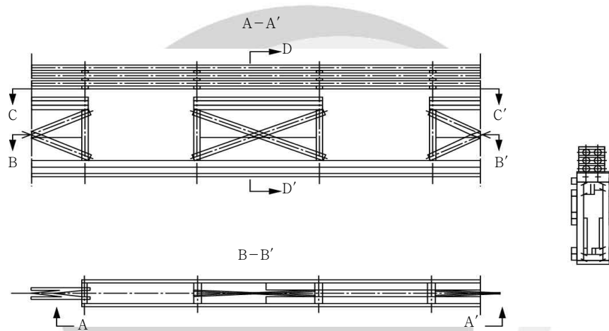
그림 3.3-6 지하매설물 보호도(예시) : 통신지중 케이블 보호도(받치는 경우)
