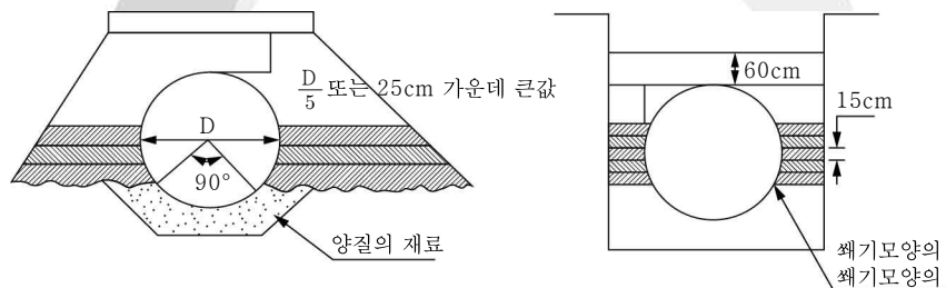
그림 3.2-3 흙쌓기와 뒤채움 기준
