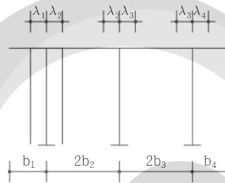
그림 4.8-5 플랜지의 유효폭
