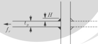
그림 4.1-1 횡방향 응력을 받는 필릿용접 목두께에 대한 허용피로응력범위
