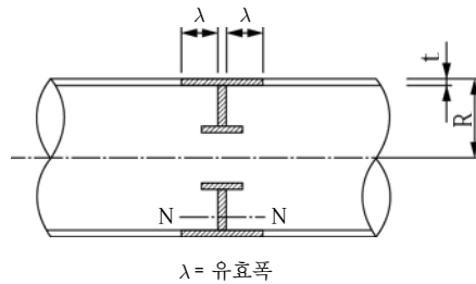
그림 4.8-2 강관의 유효폭
