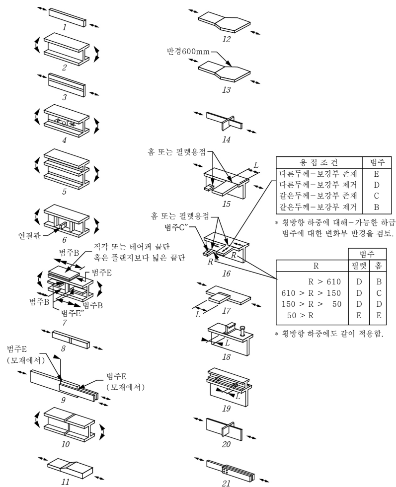
그림 4.1-2 범주의 분류 예
