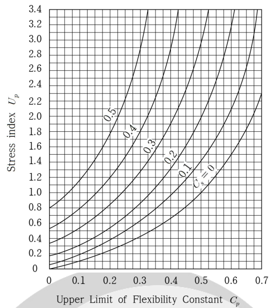
그림 4.2-1 주부재의 한계연성도계수
