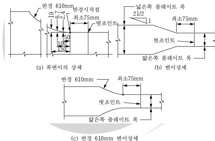
그림 4.2-1 이음부 상세
