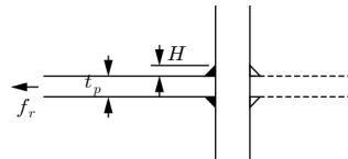
그림 4.1-1 횡방향 응력을 받는 필릿용접 목두께에 대한 허용피로응력범위
