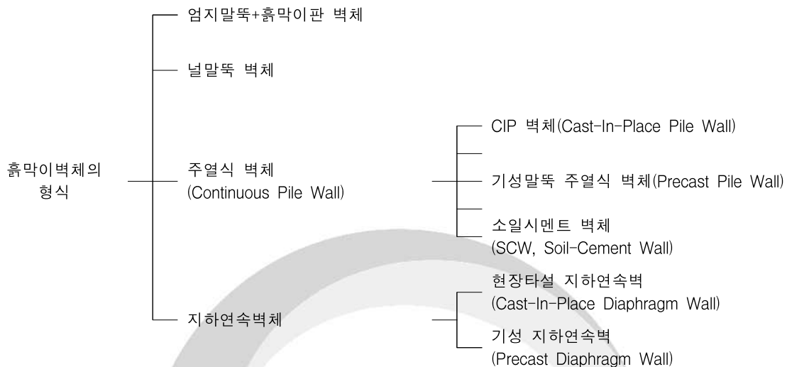
그림 3.1-1 흙막이벽체 형식
