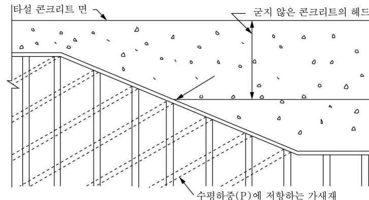
그림 1.6-1 횡방향 또는 종방향 기울기에 의한 수평하중
