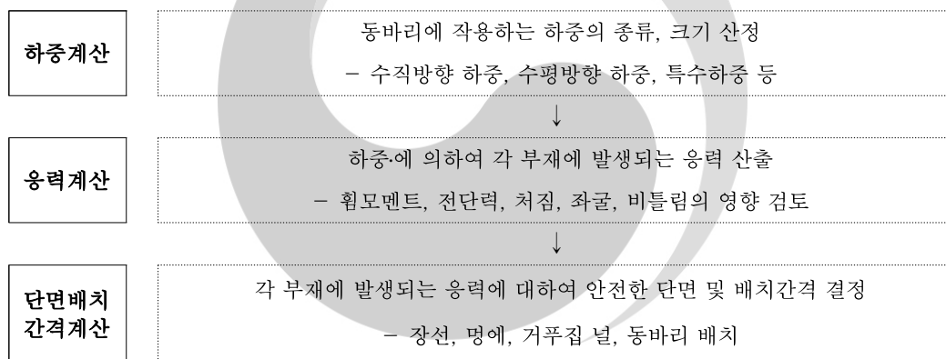
그림 1.10-1 구조설계 순서도
