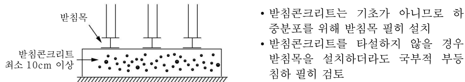
그림 3.3-1 허용지지력에 근거한 하부 기초의 지지 형식
