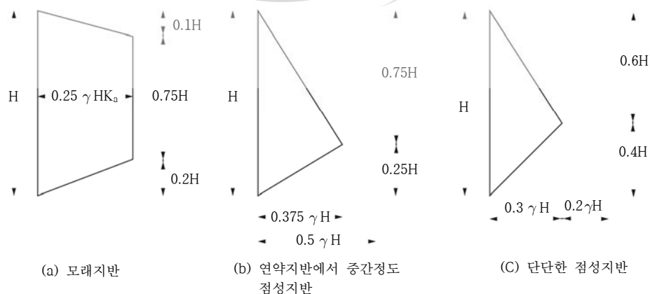
그림 1.3-2 Tschebotarioff(1973)의 토압분포도
