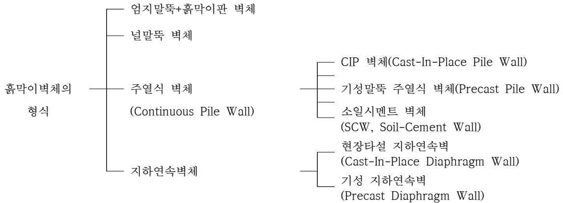
그림 1.2-1 흙막이벽체 형식
