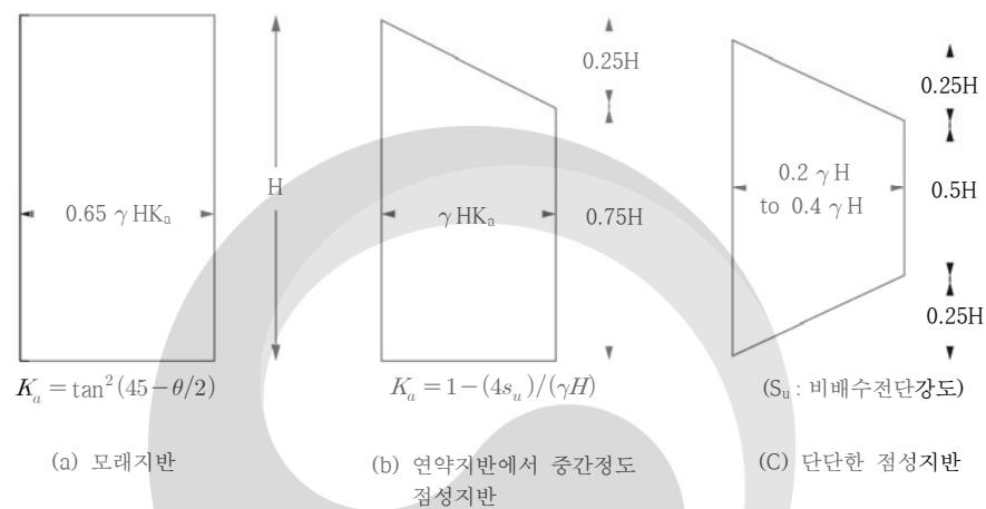
그림 1.3-1 Peck(1969)의 수정토압분포도
