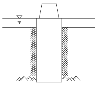
그림 4.1-3 부력 또는 양압력의 작용이 확실하지 않은 경우
