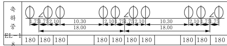
그림 4.1.8 EL표준열차하중(단위:kN/m)
