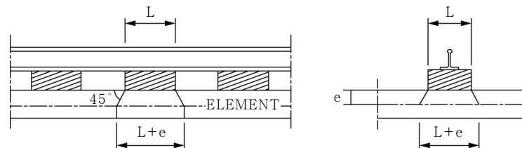
그림 4.1.7 콘크리트 도상 경우의 하중 분포도
