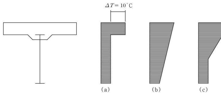
그림 4.1-10 온도차의 분포상태
