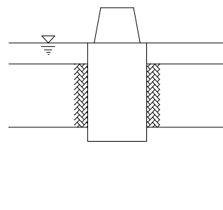
그림 4.1-3 부력 또는 양압력의 작용이 확실하지 않은 경우
