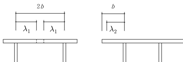
그림 4.8-1 플랜지의 유효폭
