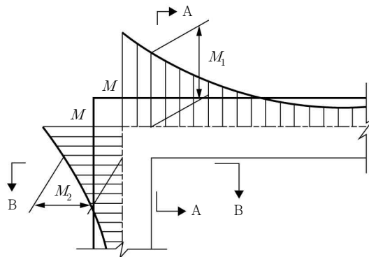
그림 4.12-1 모서리부의 설계휨모멘트
