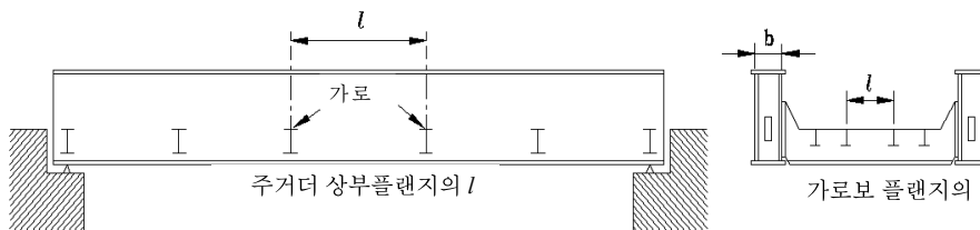
그림 4.2-5 하로 박스거더교
