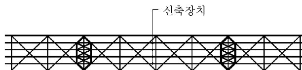
그림 4.7-2 신축장치가 있는 경우의 제동트러스 위치
