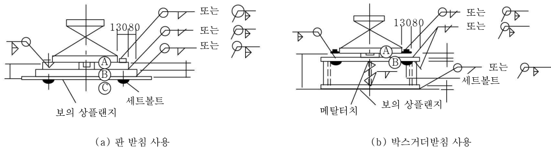
그림 4.12-10 교량받침의 연결방법
