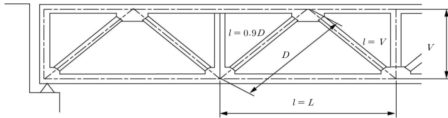
그림 4.2-9 트러스
