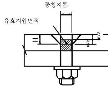
그림 4.6-9 겹치머리볼트의 유효지압면적
