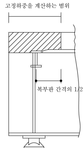
그림 4.9-6 단부 버팀재
