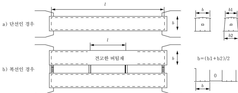
그림 4.2-2 상로 박스거더교
