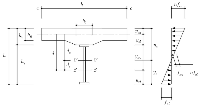
그림 4.9-1 합성거더의 기호
