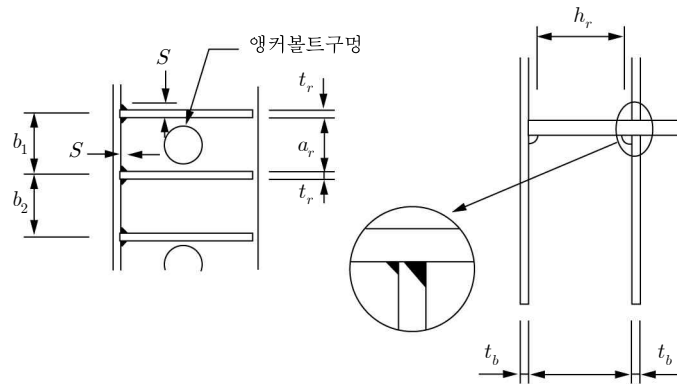
그림 4.12-6 리브의 설치
