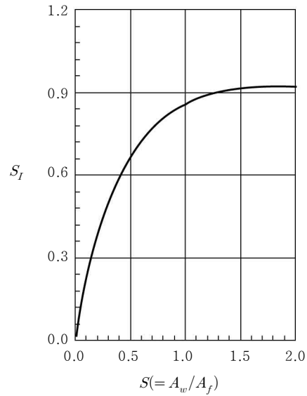
그림 4.12-3 전단지연의 추정도
