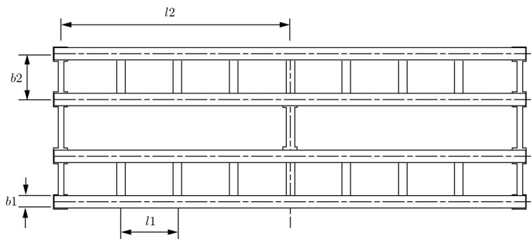
그림 4.2-8 드워프 거더교
