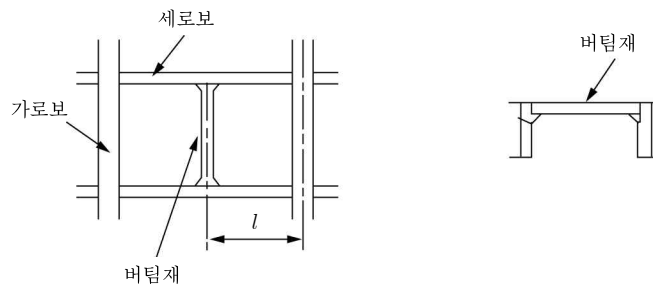
그림 4.2-4 세로보
