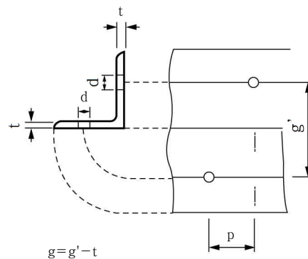
그림 4.6-11 L형강의 전개방법
