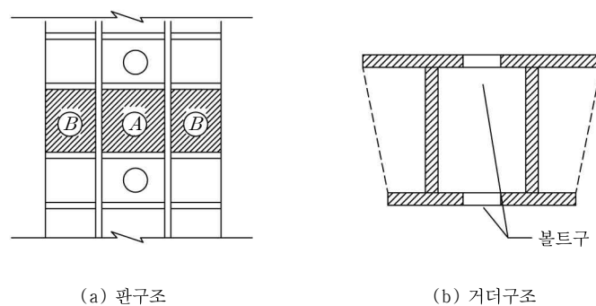
그림 4.12-7 앵커프레임의 구조
