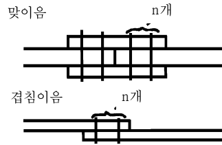
그림 4.6-8 응력계산에 사용되는 볼트의 수
