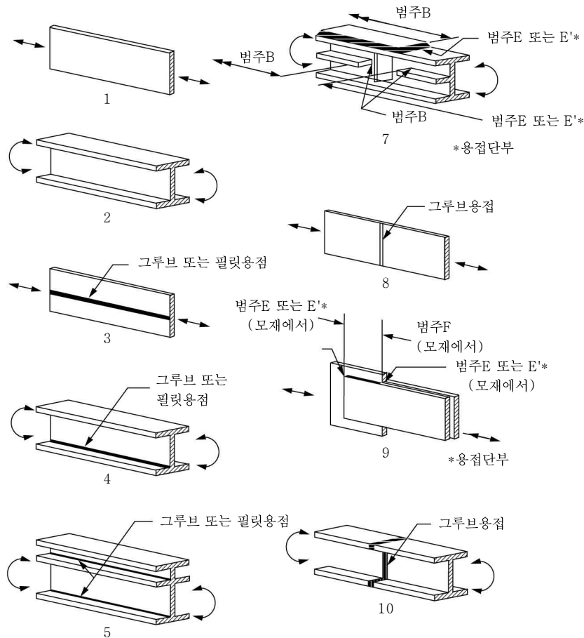
그림 4.2-11 피로상세범주
