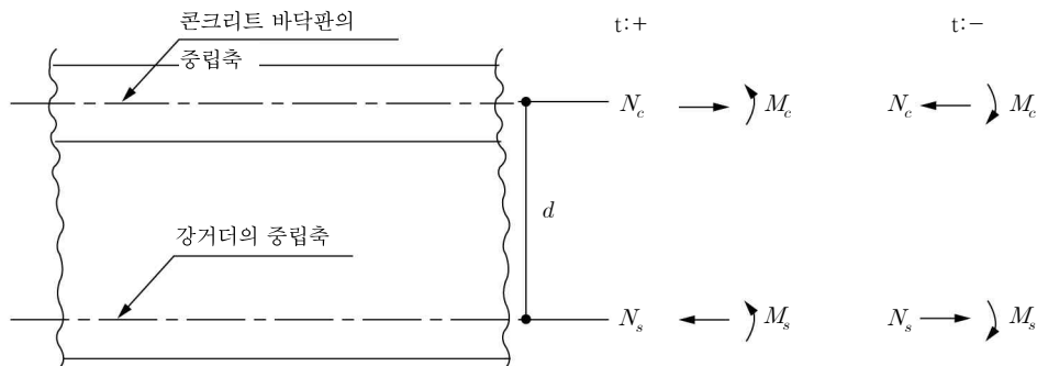
그림 4.9-5 온도차에 의해 발생되는 합성거더의 단면력
