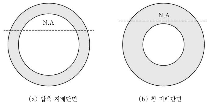
그림 2.6-1 극한상태에서의 중립축 위치에 따른 단면구분
