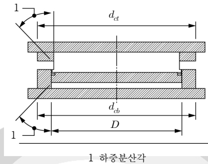
그림 4.2-3 구성요소에 의한 하중분산
