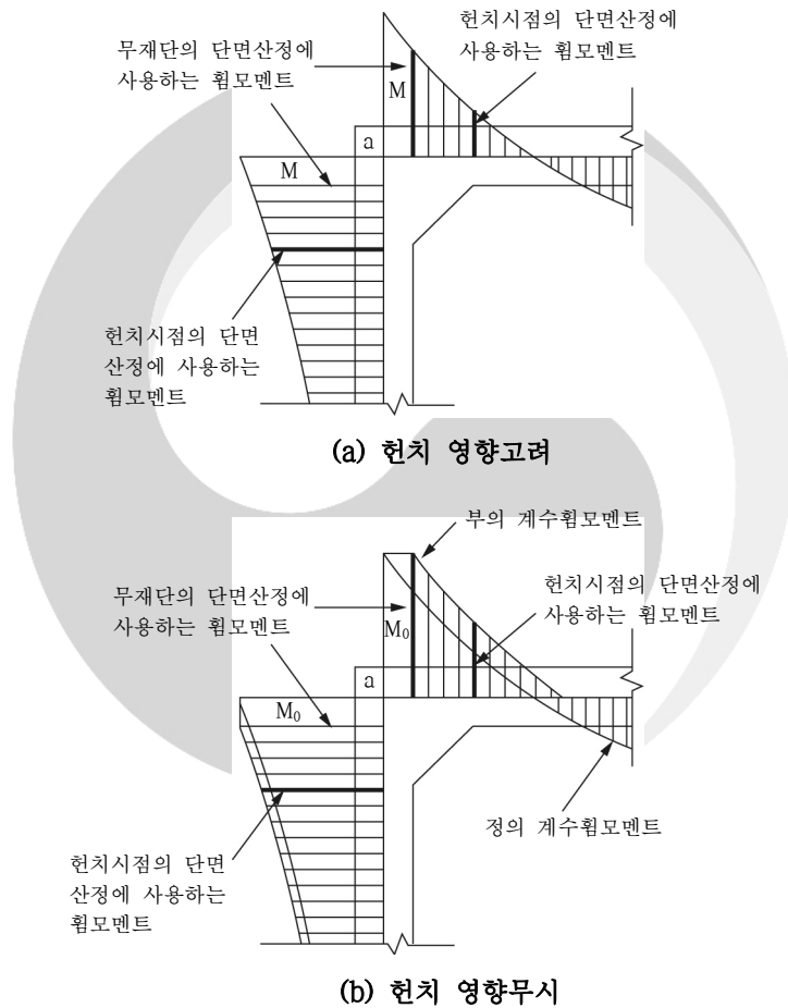
그림 4.12-5 라멘부재 절점부의 설계휨모멘트
