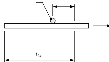
(d) 횡철근용접갈고리
