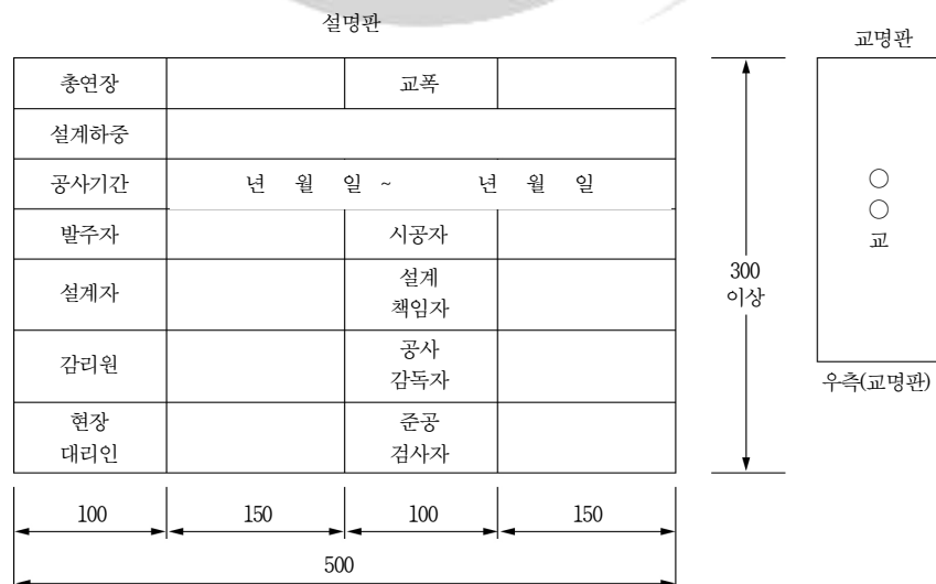
그림 1.7-1 교명판
