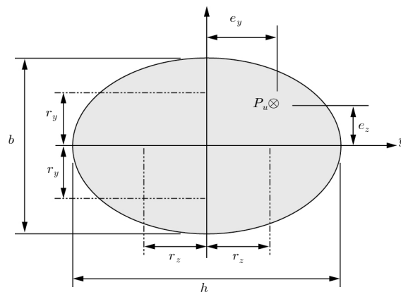
그림 4.1-2 편심의 정의
