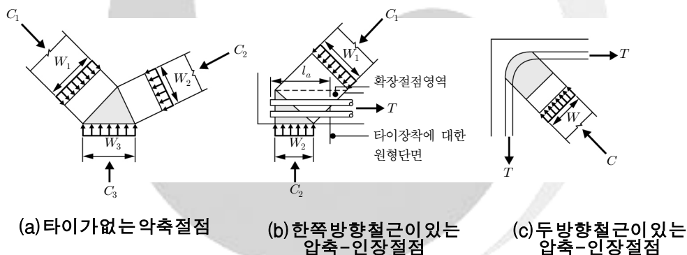
그림 4.1-13 절점의 종류
