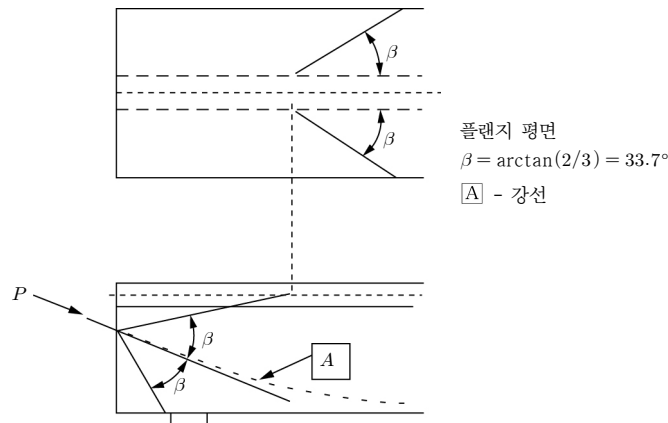
그림 4.6-21 프리스트레스의 전달
