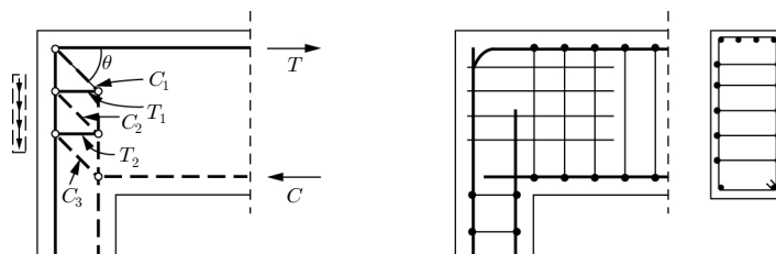
(b)기둥과보의깊이가크게다른경우
