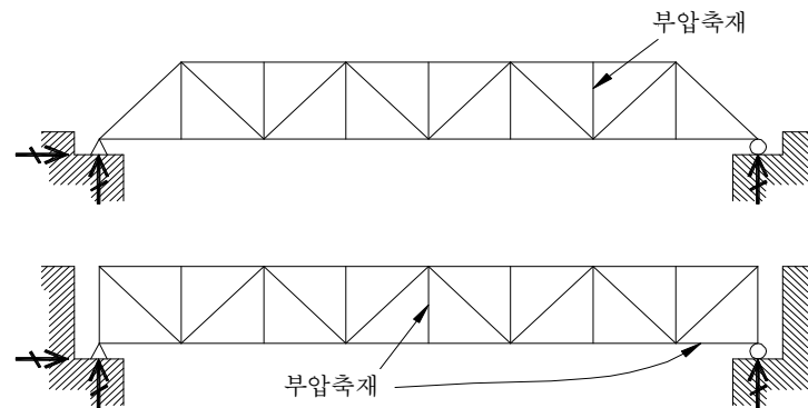
그림 4.1-1 부압축재
