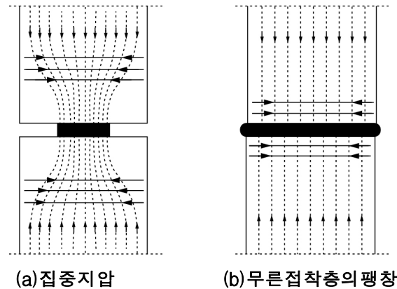
그림 4.7-3 압축연결부의 횡방향 인장 응력
