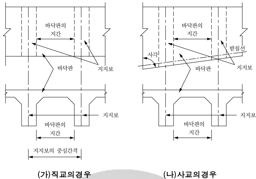
그림 4.6-3 단순판 및 연속판의 지간
