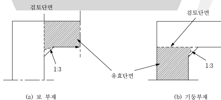
그림 4.2-5 헌치의 유효부분
