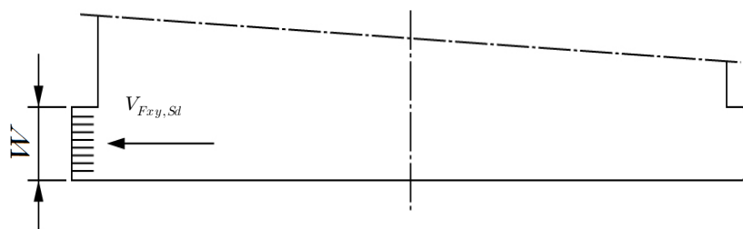
그림 4.2-4 직선 접촉면
