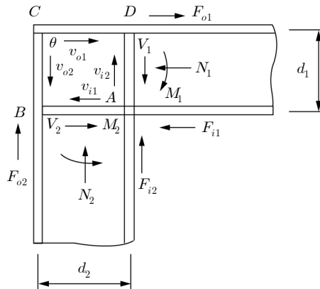
그림 4.12-2 모서리부에 작용하는 외력
