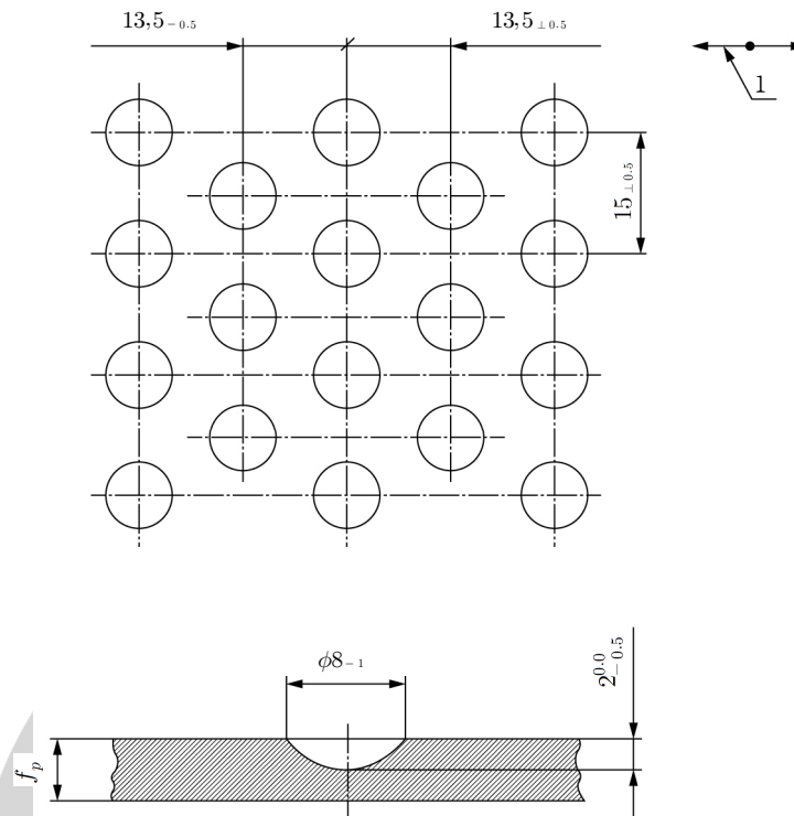
그림 4.2-8 댐플의 형상과 패턴
