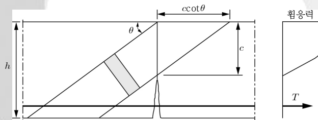
그림 4.1.5 세그먼트 조립 공법으로 시공된 교량 상부구조 복부의 경사 응력장의 제한
