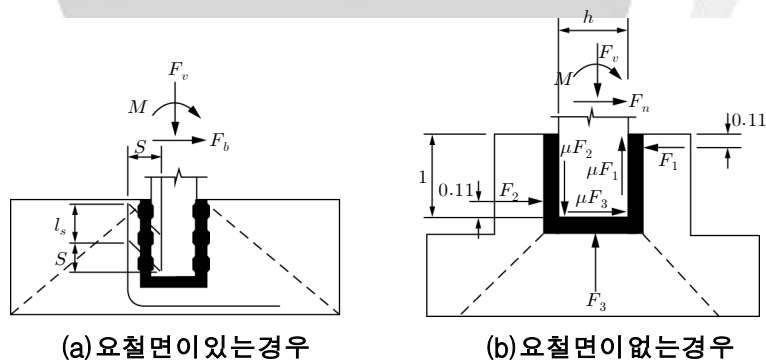
그림 4.7-7 포켓기초
