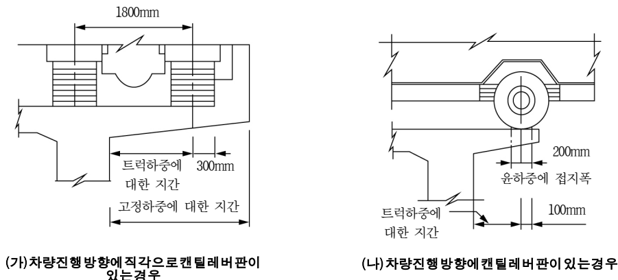
그림 4.6-4 캔틸레버판의 지간
