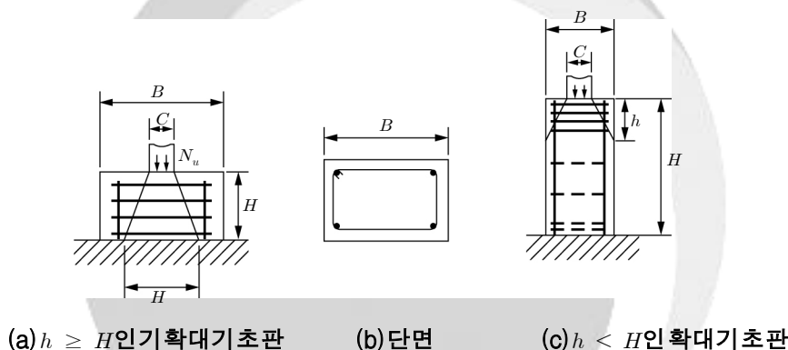
그림 4.6-15 암반 위 기초의 쏄임 방지 철근
