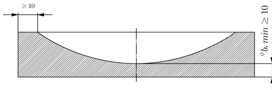
그림 4.2-6 오목한 면을 가진 지지판의 치수 제한
