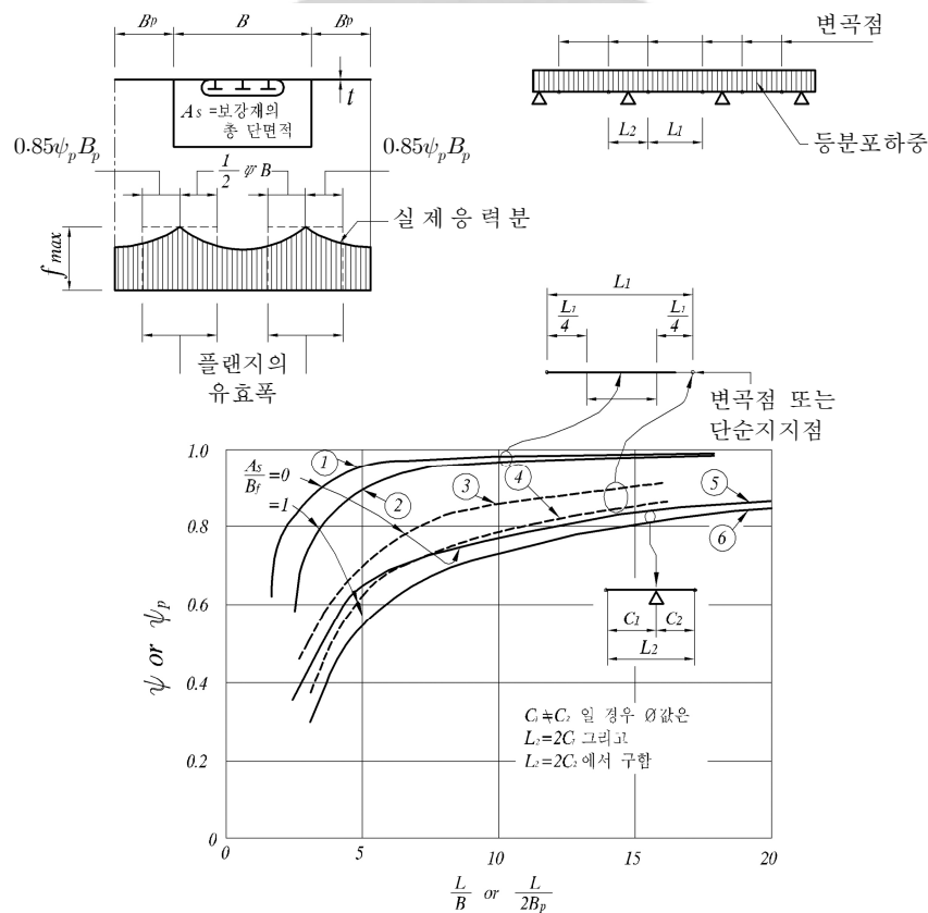
그림 4.6-10 바닥판의 유효폭
