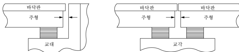
그림 4.2-2 교량의 여유간격
