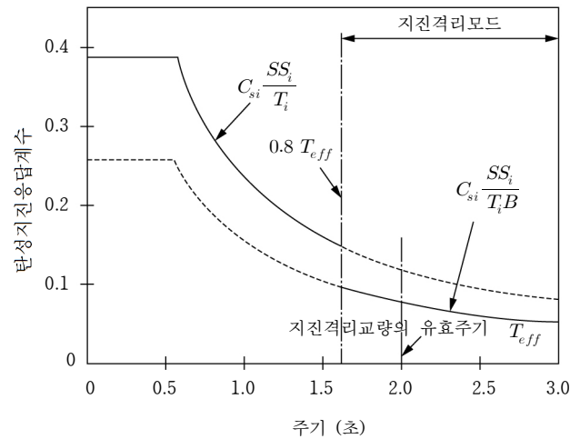
그림 4.7-2 지진격리교량의 탄성지진응답계수
