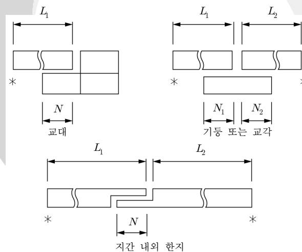
그림 4.2-1 최소 받침지지길이 규정에 관한 치수
