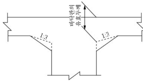
그림 4.9-3 현치부분의 슬래브의 유효깊이
