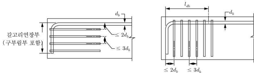
그림 4.5-7 표 4.5-4에 규정한 표준갈고리 연장부를 띠철근 또는 스티럽을 정착된 철근에 평행으로 둘러싼 경우
