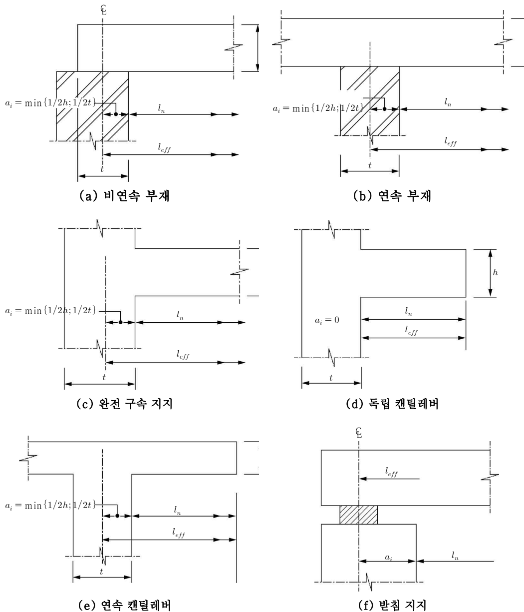
그림 1.5-1 구속조건에 따른 유효경간
