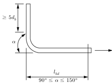
(a) 구부림 각도가 90^\circ 에서 150^\circ 사이인
