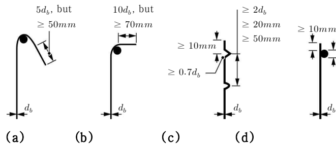
그림 4.5-8 스텝, 락철근의 정착
