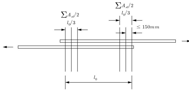
(a) 인장철근
