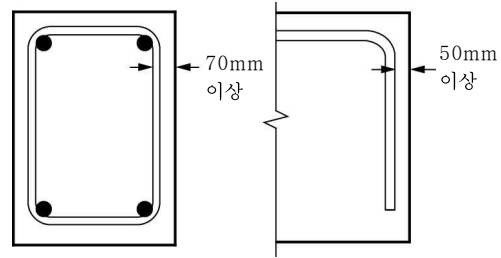
그림 4.5-6 표 4.5-4에 규정한 표준갈고리의 피복두께
