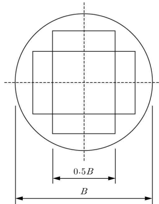
그림 4.6-13 원형 확대기초판의 직교 철근
