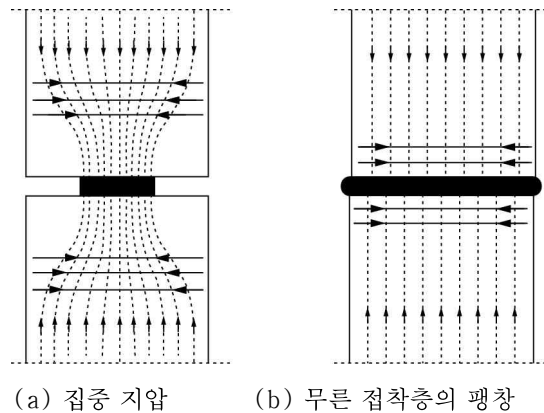
그림 4.7-3 압축연결부의 횡방향 인장 응력
