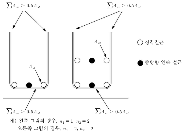
그림 4.5-14 횡방향 압축력이 작용하지 않는 구역에서 지름이 큰 철근을 정착
