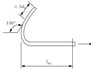
(b) 구부림 각도가 150^\circ 이상인 갈고리
