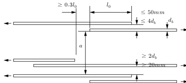
그림 4.5-10 인접 겹침이음
