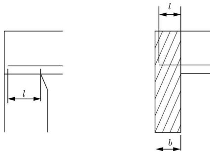
(a) 직접 반력이 작용하는 경우 (b) 간접 반력이 작용하는 경우
