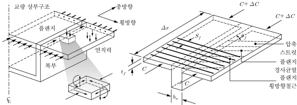
그림 4.1-6 플랜지의 전단
