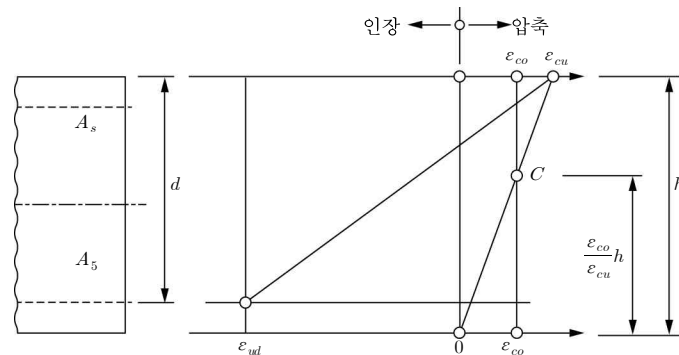
그림 4.1-1 극한한계상태의 단면 변형률 분포
