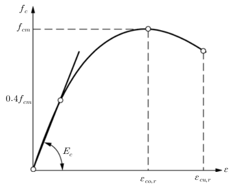
그림 3.1-1 비선형 해석을 위한 콘크리트의 응력-변형률 곡선
