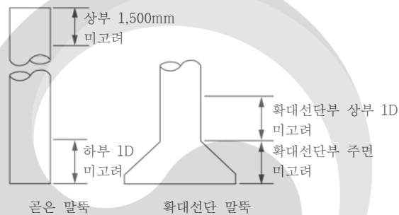
그림 3.4-1 주면마찰력을 계산할 때 고려하지 않는 현장타설말뚝의 각 부분에 대한 설명 (O'Neill과 Reese, 1999)
