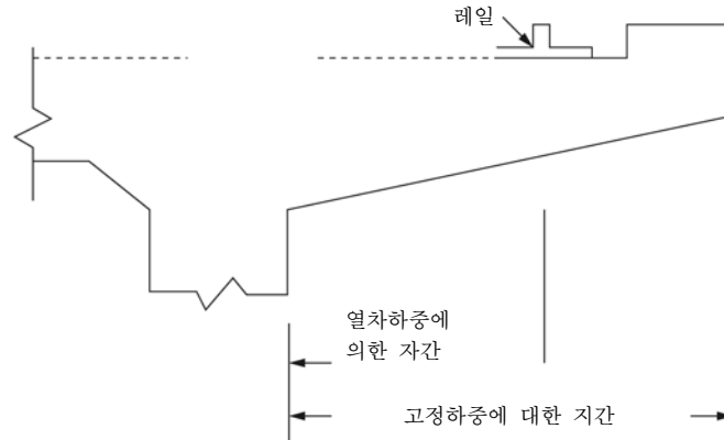
그림 4.8-2 캔틸레버판의 지간
