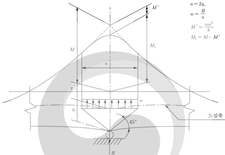
그림 4.11-3 중간지점상의 설계휨모멘트
