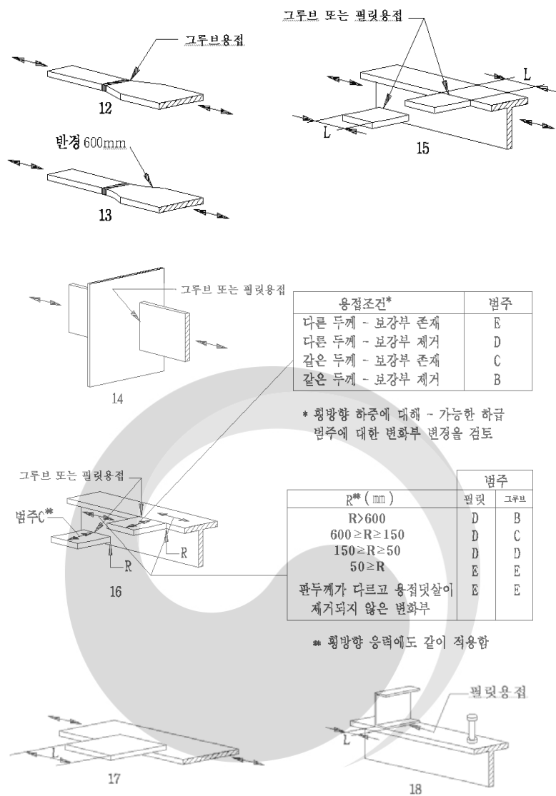
그림 4.2-11 피로상세범주(계속)
