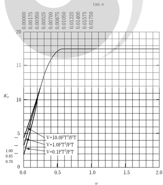
그림 3.3-8 \phi_f=40^\circ 일 경우 K_\delta (Hannigan 등, 2006)
