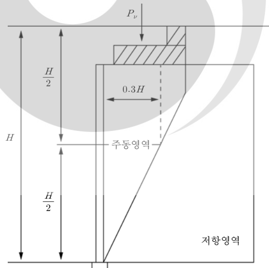
그림 3.9-12 상재 슬래브의 크기가 클 경우 최대 인장력 선의 위치(비신장성 보강재)
