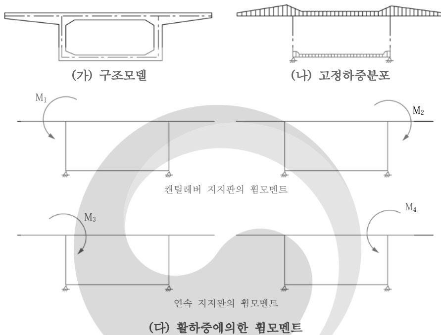
그림 4.13-5 하부플랜지 및 복부의 휨모멘트
