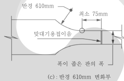
그림 4.9-1 이음부 상세
