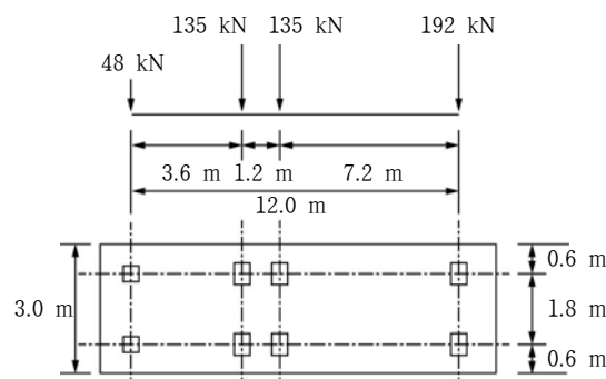
그림 4.3-1 표준트럭하중
