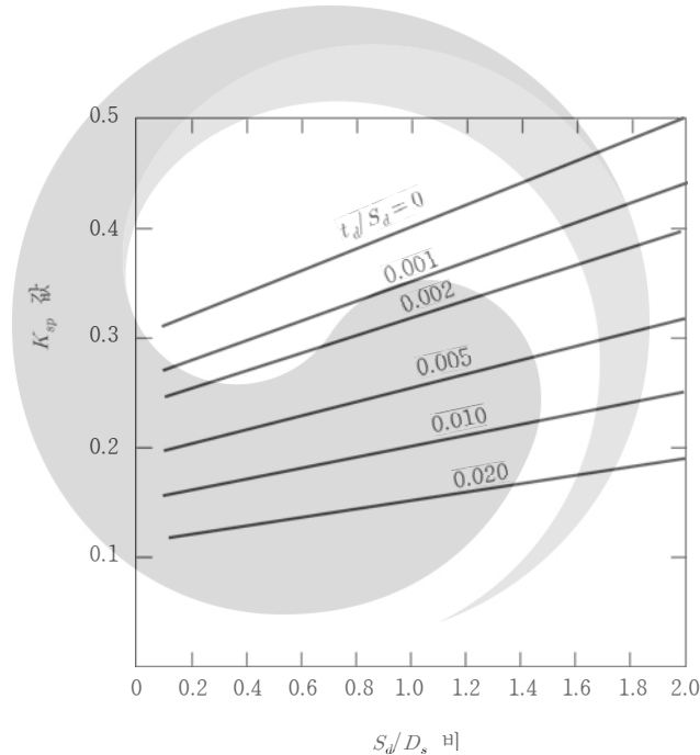
그림 3.3-14 지지력계수 (캐나다 지반공학회, 1985)
