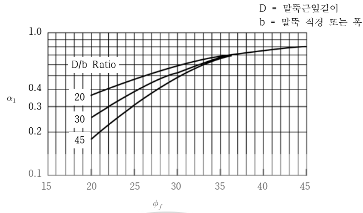
그림 3.3-11 \alpha_t 계수 (Hannigan 등, 2006)
