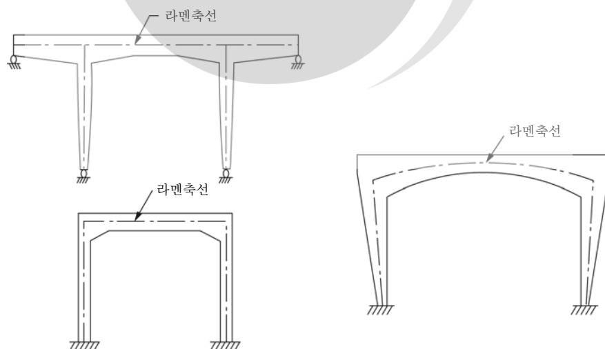
(a) 라멘축선의 변화를 무시해도 좋은 경우
