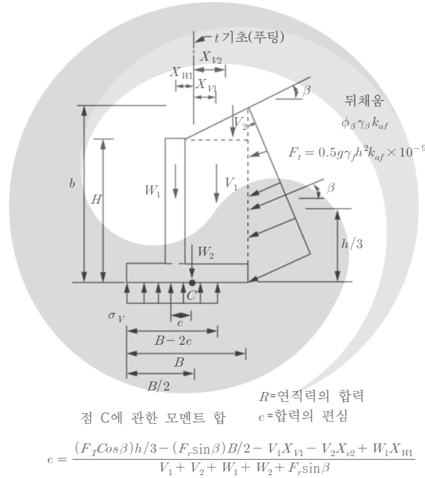
그림 3.5-1 토질기초에 지지된 벽체의 지지력 기준
