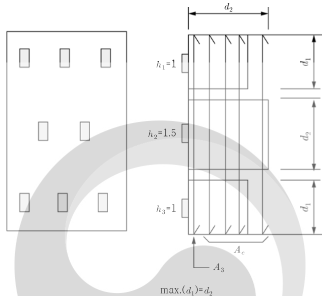
그림 4.5-2 파열효과와 표면효과에 대한 철근보강
