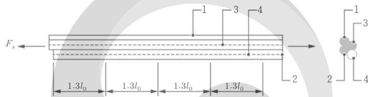
그림 4.5-16 4개의 철근을 포함하는 인장 영역의 겹침이음 연결부
