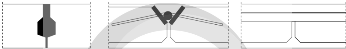
(a) 콘크리트 또는 그라우팅 연결 (b) 용접 또는 볼트 연결 (c) 배근된 마감 연결
