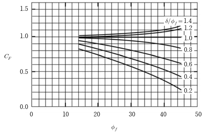
그림 3.3-9 \delta \approx \phi_f 일 경우 K_\delta 의 수정계수 (Hannigan 등, 2006)
