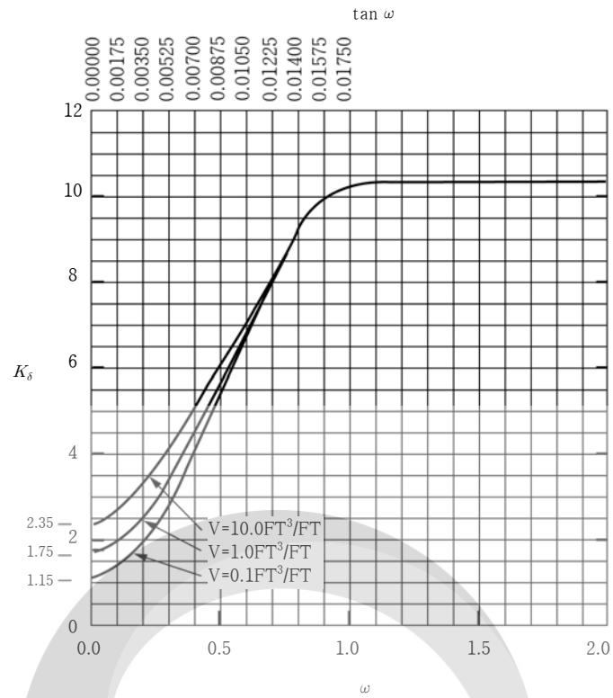
그림 3.3-7 \phi_f=35^\circ 일 경우 K_\delta (Hannigan 등, 2006)
