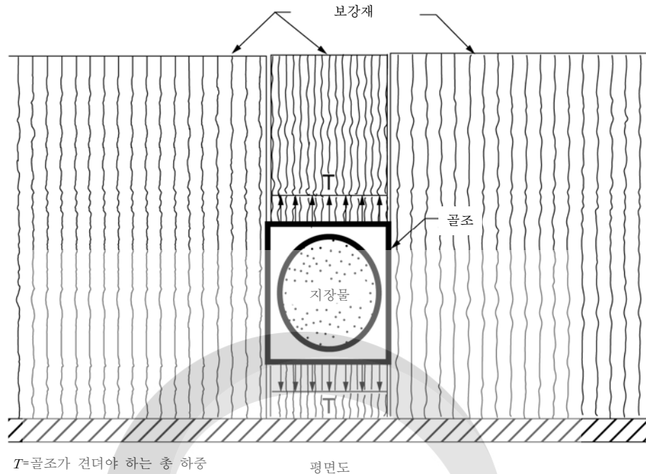
그림 3.9-13 뒤택음 방해물 주위의 보강토의 구조적인 연결
