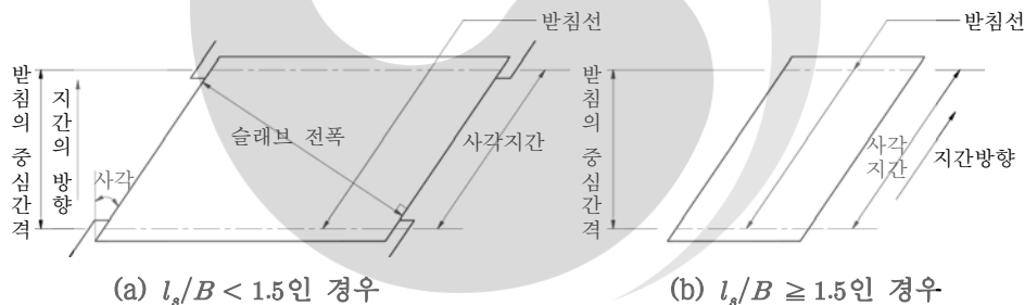
그림 4.9.2 사각슬래브교의 지간방향
