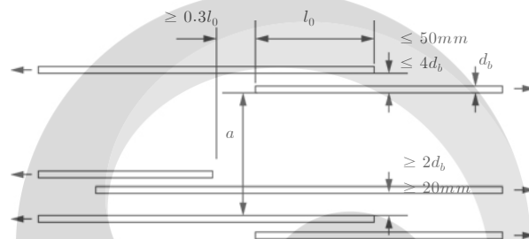
그림 4.5-10 인접 겹침이음
