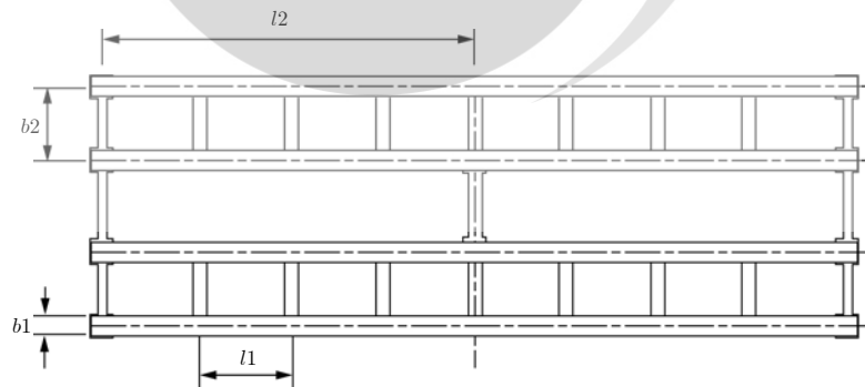
그림 4.2-8 드워프 거더교
