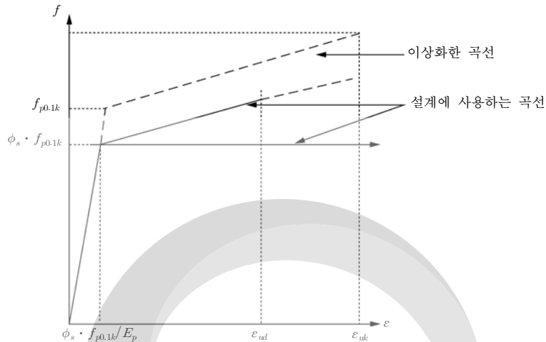
그림 3.3-1 프리스트레싱 강재의 설계응력-변형률 관계
