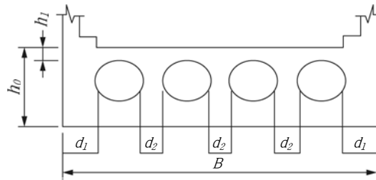
(a) 속 빈 슬래브교의 단면형상
