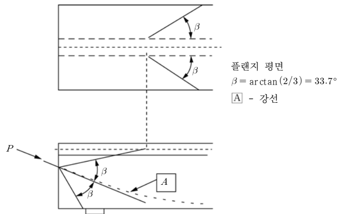
그림 4.6-21 프리스트레스의 전달
