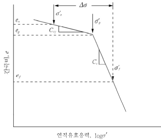
그림 3.2-2 과압밀 점성토의 전형적인 압밀곡선 - 간극비 대 연직유효응력(EPRI, 1983)
