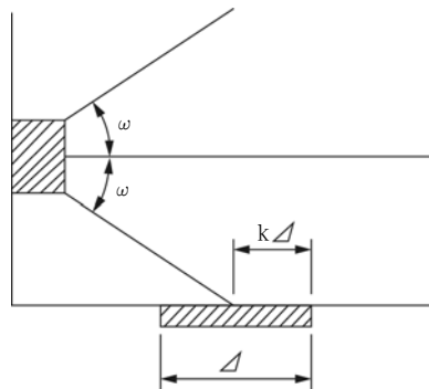
그림 4.5-9 최소 보강 계산 방법
