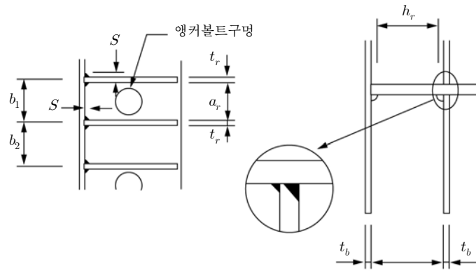
그림 4.12-6 리브의 설치
