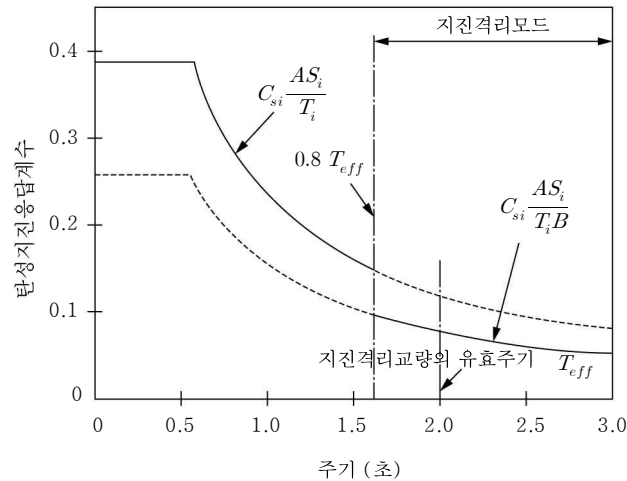
그림 2.7-2 지진력리모드의 탄성지진응답계수
