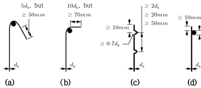
그림 4.5-8 스티럽, 락철근의 정착
