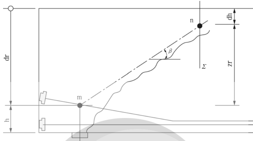
그림 4.5-5 단부 스트럿
