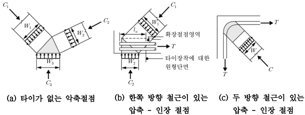
그림 4.1-13 절점의 종류
