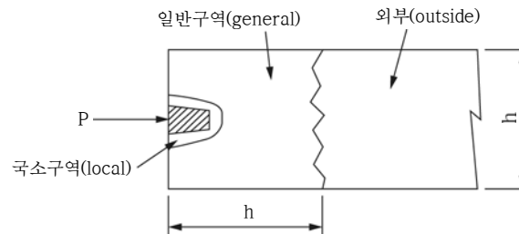
그림 1.2-1 정착구역
