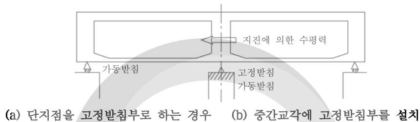
그림 4.11-5 고정받침부에서의 수평반력
