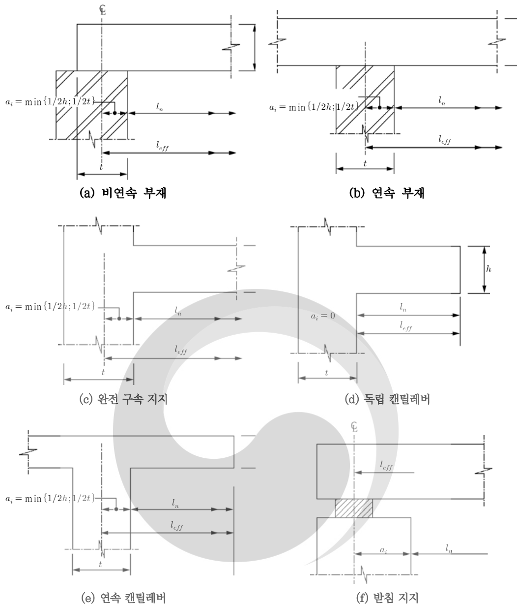
그림 1.5-1 구조조건에 따른 유효경간
