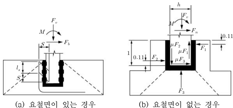
그림 4.7-7 포켓기초
