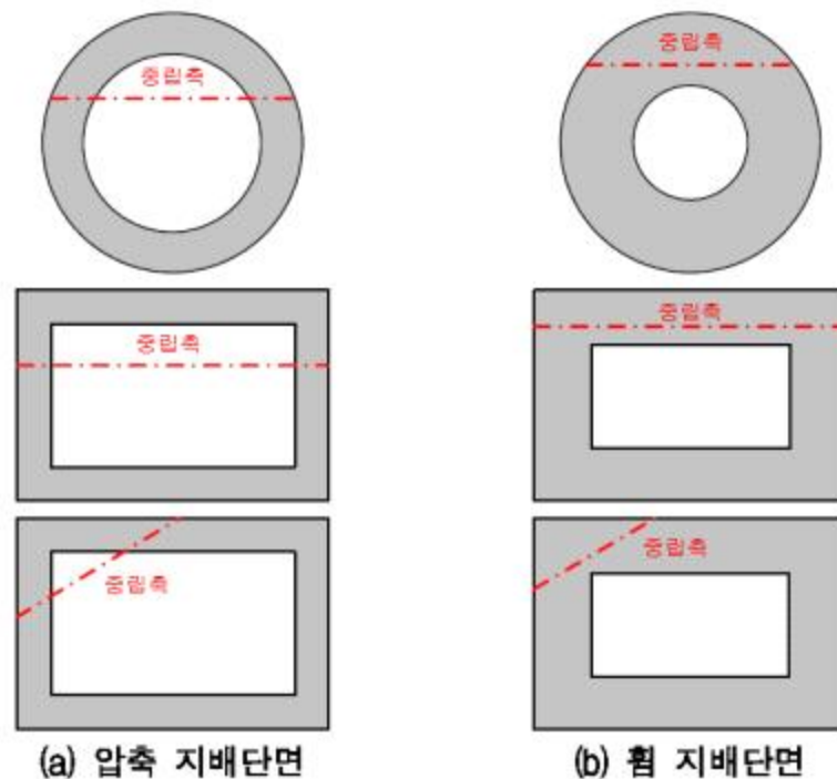
그림 2.6-1 극한상태에서의 중립축 위치에 따른 단면구분
