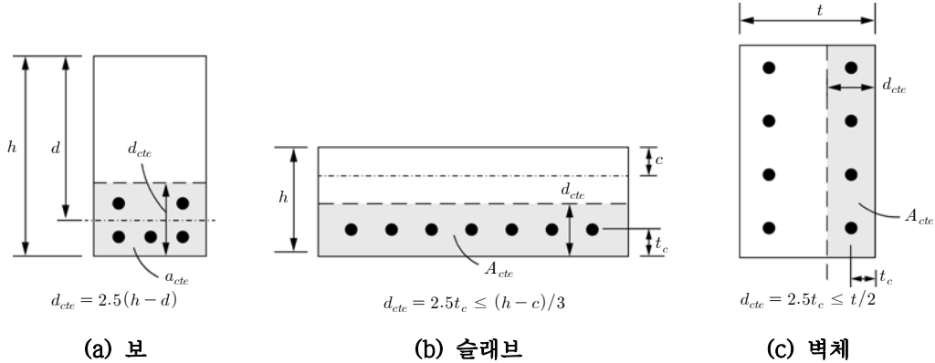
그림 4.2-1 유효 인장 면적
