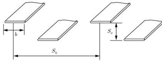
불연속 토목섬유 보강재
