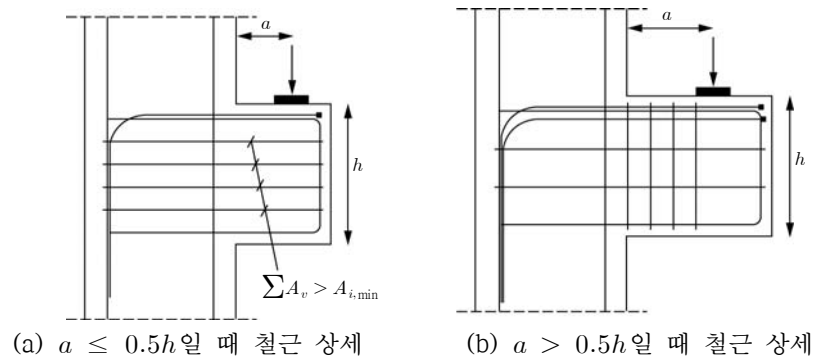
그림 4.6-20 내민발침의 철근 상세
