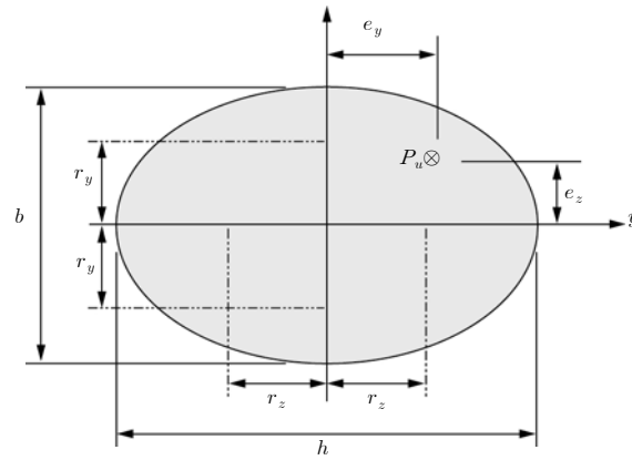
그림 4.1-2 편심의 정의
