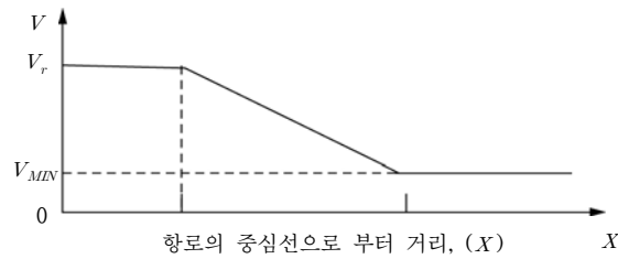
그림 4.18-3 설계충돌속도의 분포도
