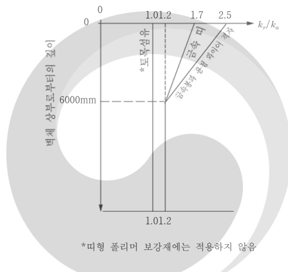
그림 3.9-6 보강토 응력의 깊이에 따른 횡토압 비 k_r/K_a 의 변화
