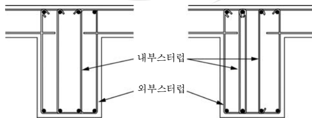
그림 4.6-4 전단철근의 예
