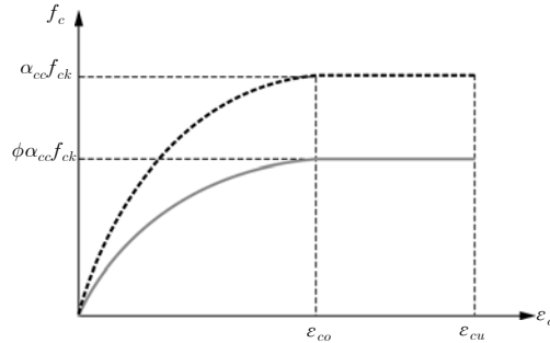
그림 3.1-3 단면설계를 위한 응력-변형률 곡선
