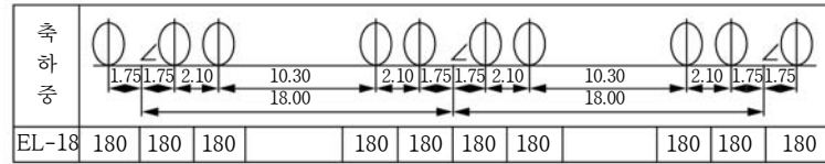
그림 4.1.8 EL표준열차하중(단위:kN/m)
