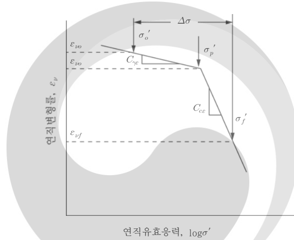
그림 3.2-3 과압밀 점성토의 전형적인 압밀곡선 - 연직변형률 대 연직유효응력(EPRI, 1983)
