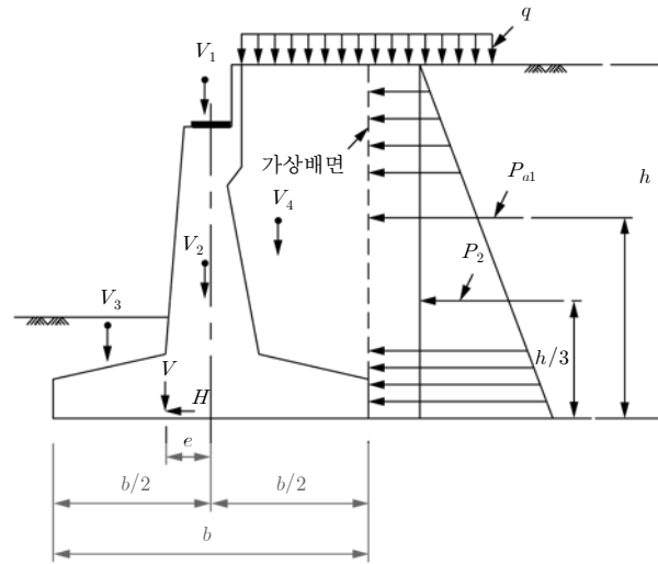
그림 4.2-3 안정계산(평상시)
