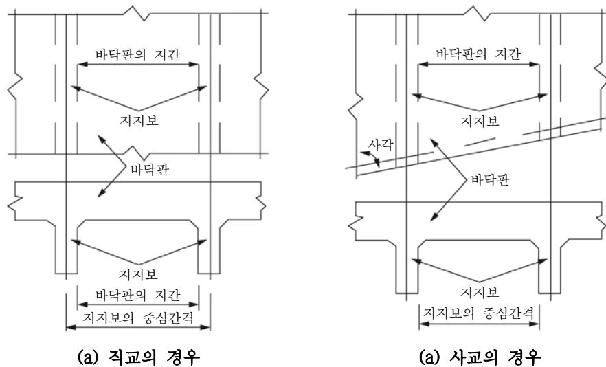
그림 4.-1 단순판 및 연속판의 지간
