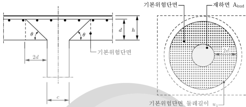
그림 4.1-9 뚫림전단 검증모델
