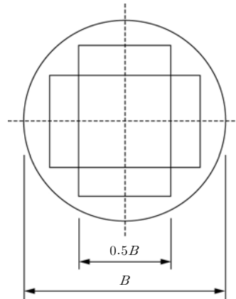
그림 4.6-13 원형 확대기초판의 직교 철근
