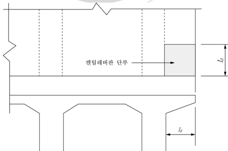
그림 4.8-9 캔틸레버판의 단부
