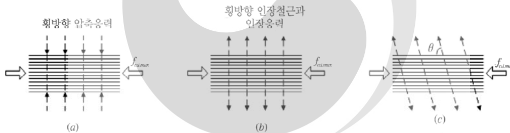
그림 4.1-12 콘크리트 스트럿의 종류
