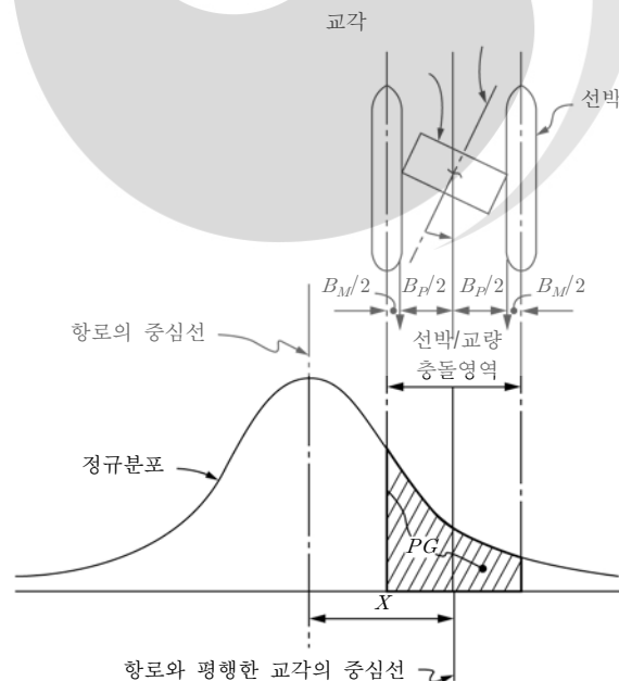
그림 4.18-2 교각충돌의 기하학적 확률
