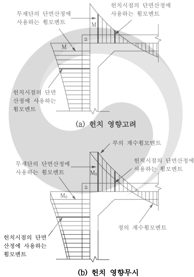
그림 4.12-5 라멘부재 절점부의 설계휨모멘트
