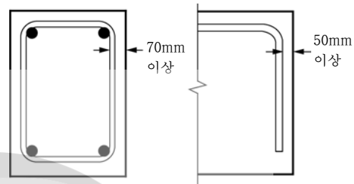
그림 4.5-6 표 4.5-4에 규정한 표준갈고리의 피복두께
