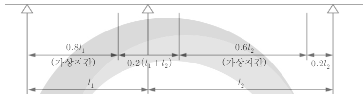
그림 4.11-1 연속슬래브교의 가상지간
