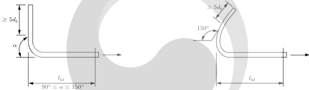
(a) 구부림 각도가 90^\circ 에서 150^\circ 사이인 갈고리
