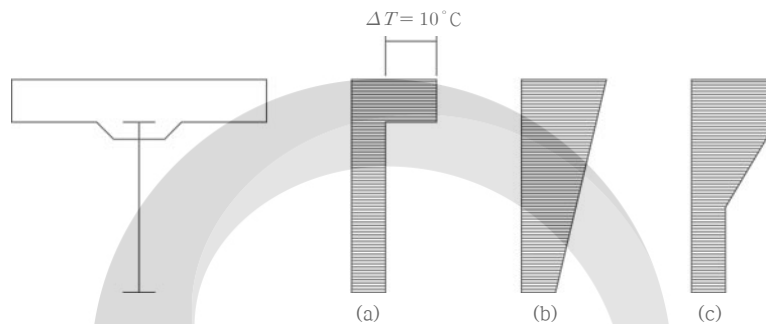
그림 4.1-10 온도차의 분포상태
