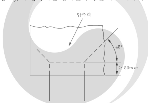
그림 4.6-12 정착 성능이 증가하는 압축영역의 확대
