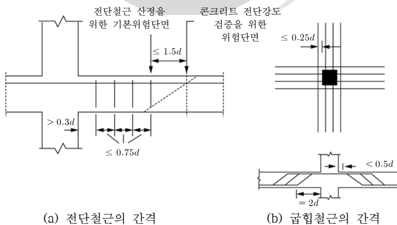
그림 4.6.11 2방향 전단철근
