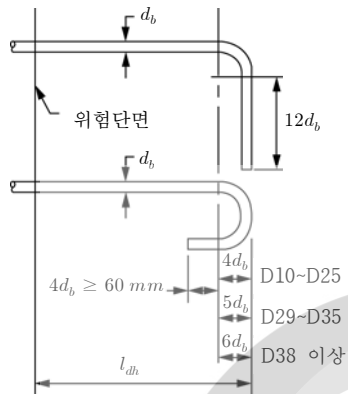
그림 4.5-5 표준갈고리의 정착을 위한 갈고리 철근 상세
