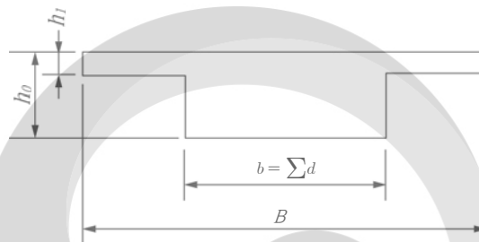
그림 4.9-1 속 빈 슬래브교의 가상 T형단면
