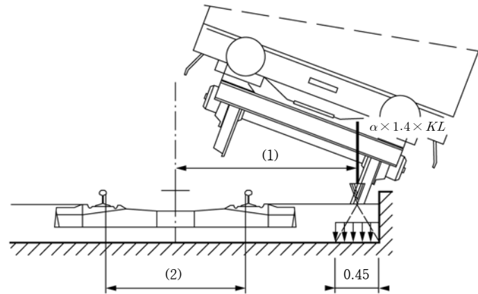
그림 4.1-13 탈선상황 II (KRL-2012하중의 등분포하중만 재하)
