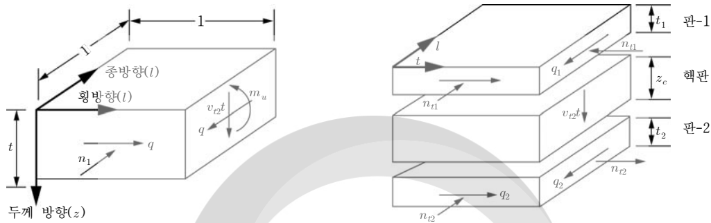
그림 4.1-16 셀요소를 접판요소로 변환
