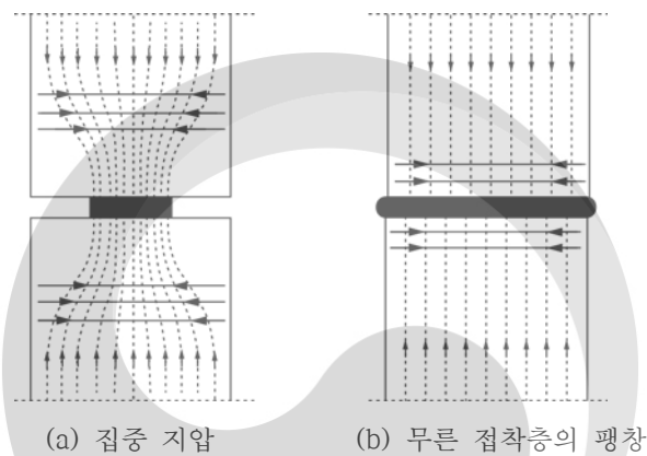
그림 4.7-3 압축연결부의 횡방향 인장 응력
