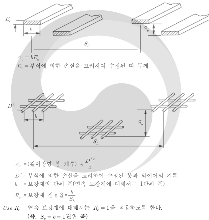
그림 3.9-9 금속 보강재에 대한 보강재 점유율
