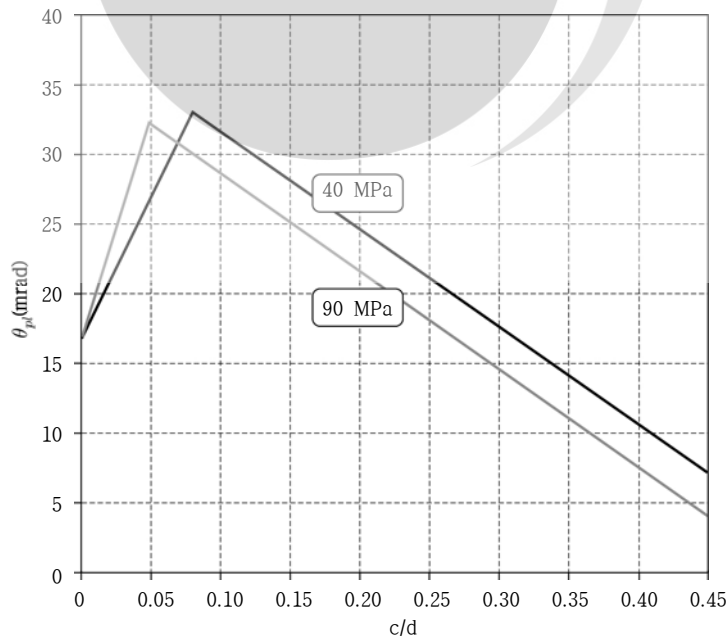
그림 1.5-2 기준 소성회전각( \theta_{pl} )
