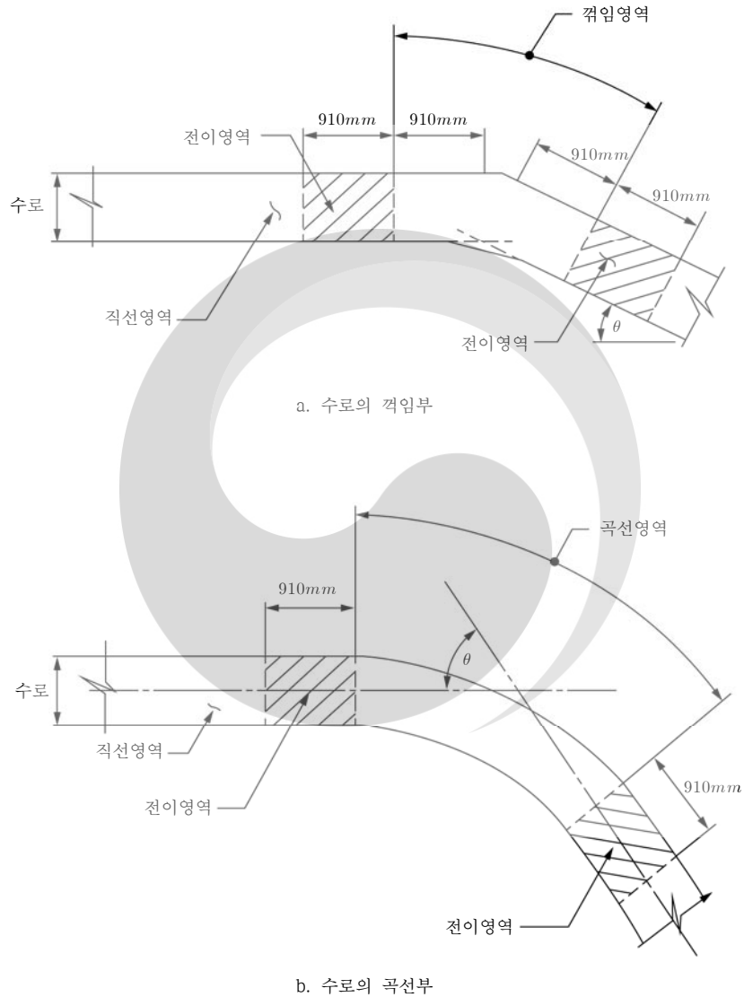
그림 4.18-1 교량 위치에 대한 수로 영역
