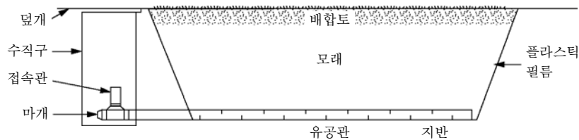
그림 4.2-5 모래층셀지반(PURR-WICK system)
