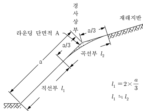
그림 4.4-1 땅깍기 비탈면의 라운딩 처리
