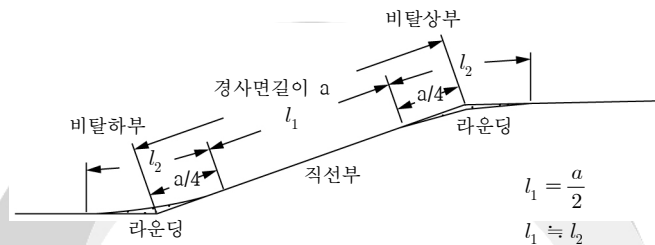
그림 4.4-2 흙쌓기 비탈면의 라운딩 처리
