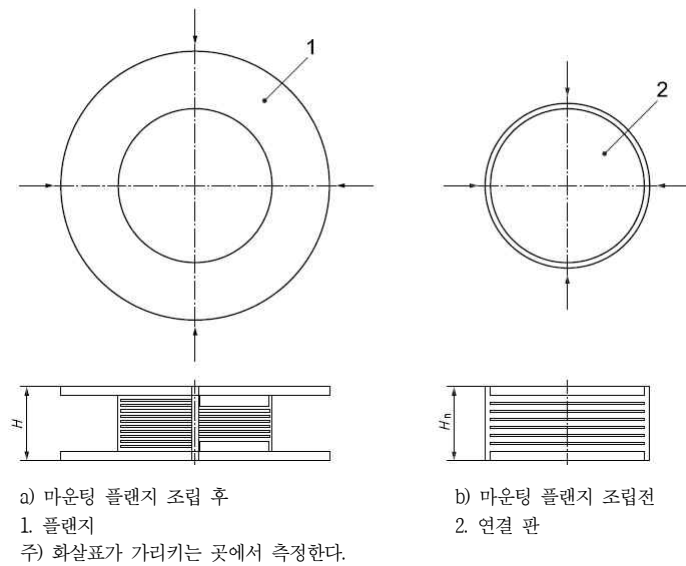
그림 2.9-2 원형 납 면진받침의 높이 측정 위치
