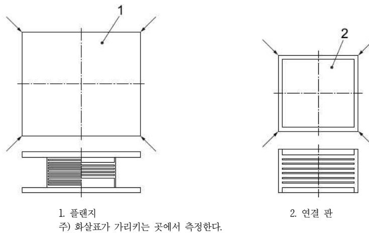
그림 2.9-3 직사각형 납 면진받침의 높이 측정 위치
