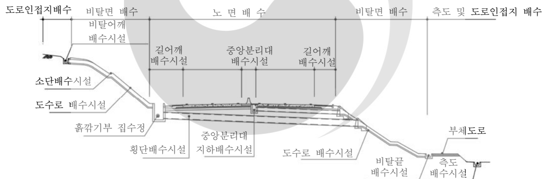
그림 1.3-1 배수시설의 명칭 및 구분
