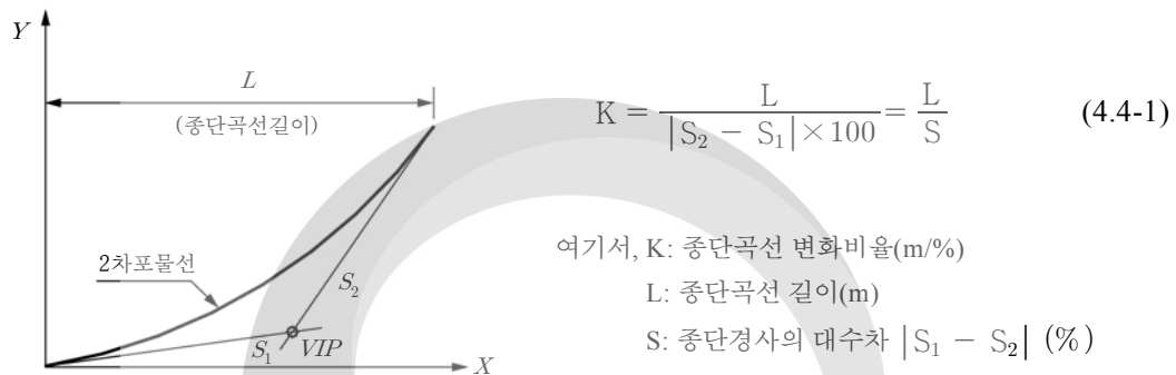
그림 4.4-1 종단곡선 변화비율
