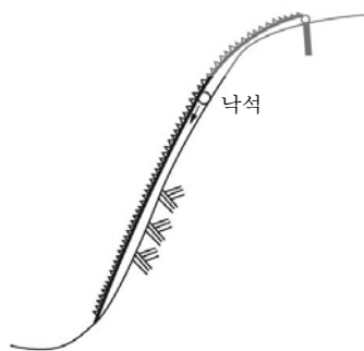
그림 4.2-2 비포켓식 낙석방지망 포켓식 낙석방지망
