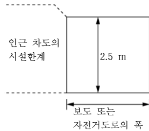
그림 4.10-1 보도 및 자전거도로의 시설한계
