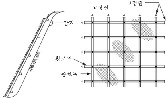
그림 4.2-1 비포켓식 낙석방지망
