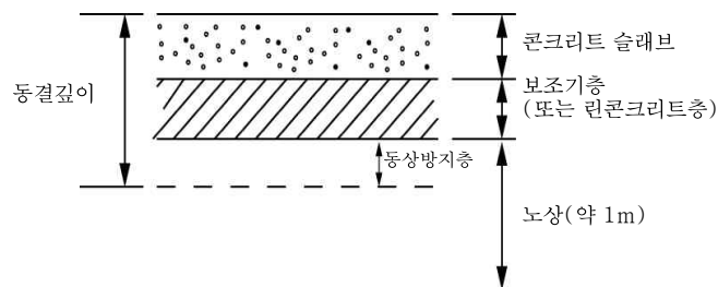
그림 1.3-2 콘크리트 포장의 구성 및 각층의 명칭
