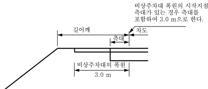
그림 4.3-2 비상주차대 횡단면도
