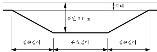
그림 4.3-1 비상주차대 평면도(예)
