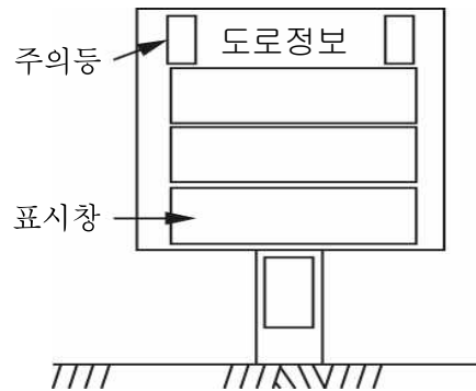
그림 4.4-2 B형 정보판
