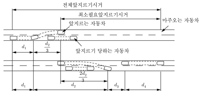
그림 4.2-1 앞지르기시거의 산정
