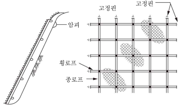
그림 4.2-1 비포켓식 낙석방지망
