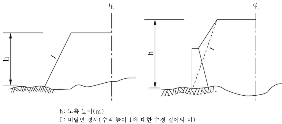
그림 4.3-2 흙쌓기부의 비탈면 경사 그림 4.3-3 구조물이 있는 경우 비탈면 경사
