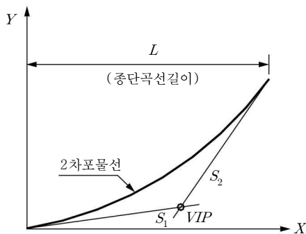
그림 4.4-1 종단곡선 변화비율
