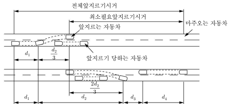
그림 4.2-1 앞지르گی시거의 산정
