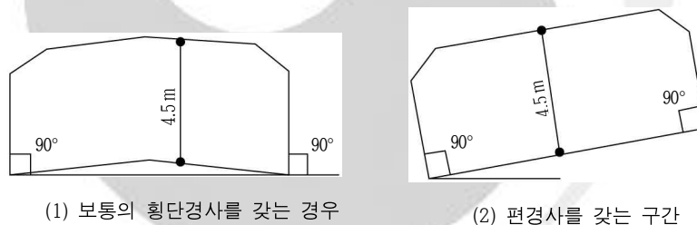
그림 4.10-2 횡단경사구간의 시설한계
